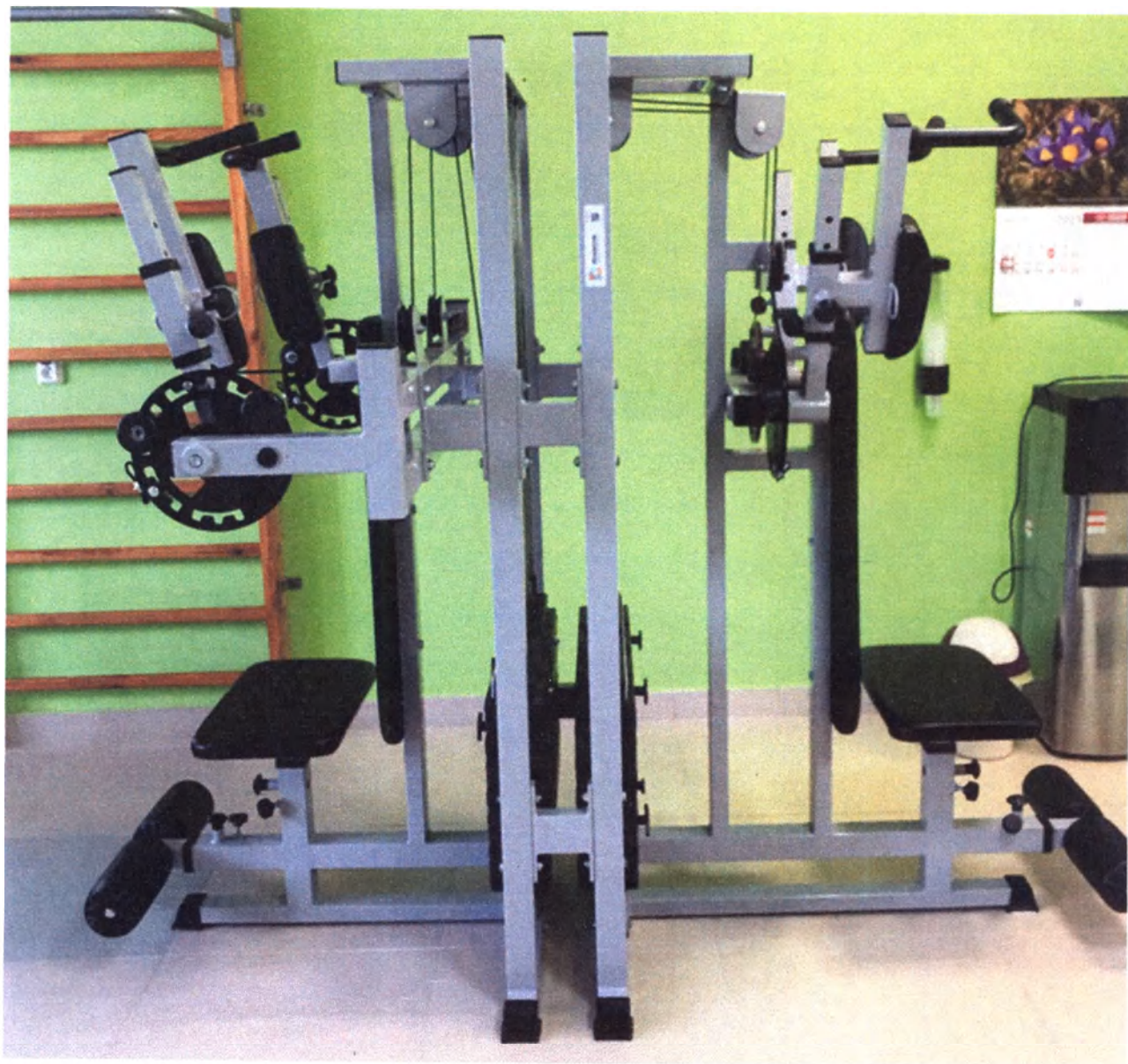
Фотографическое изображение 11 – Общий вид. Тренажер Ильясова «РУКИ-ВВЕРХ», многофункциональный (ТИРМ)
