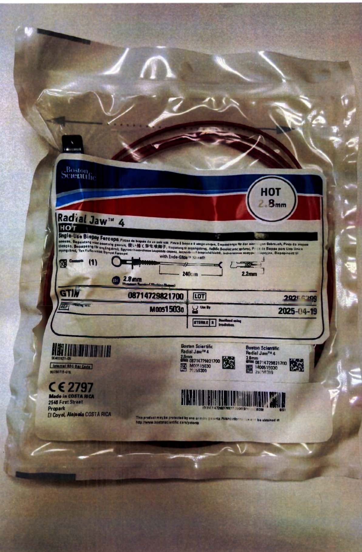
Запечатываемый пакет МИ «Щипцы эндоскопические биопсийные одноразовые Radial Jaw 4, для горячей биопсии» (сторона 1)
