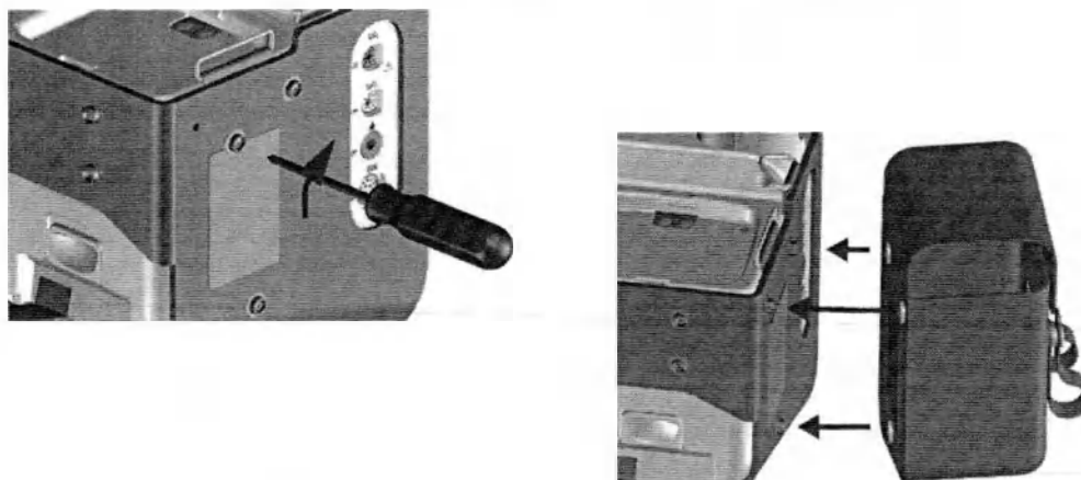
Рис. 23 Крепление лотка и боковых футляров для переноски
