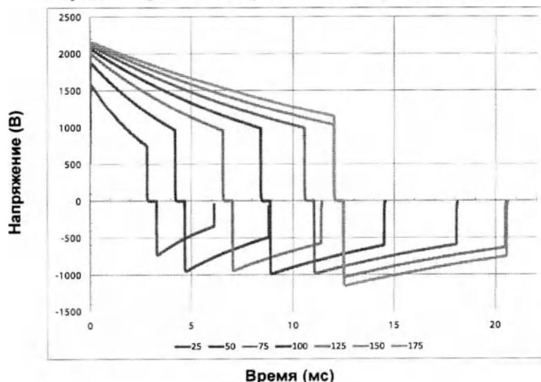
Рис. 80 Импульс SMART Biphasic
