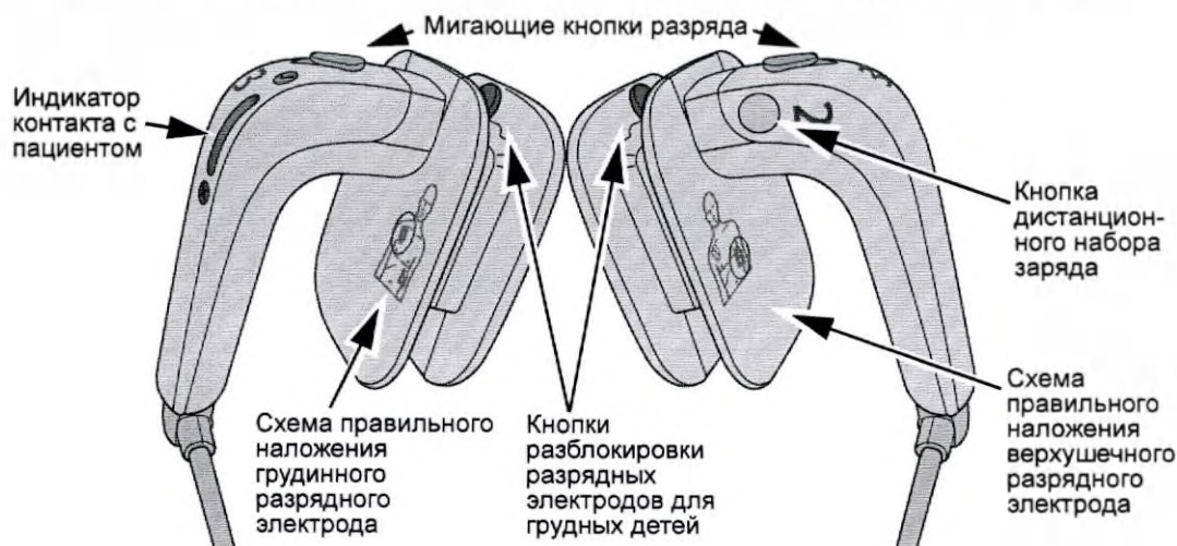
Рис. 12 Характеристики наружных разрядных электродов: M3543A
