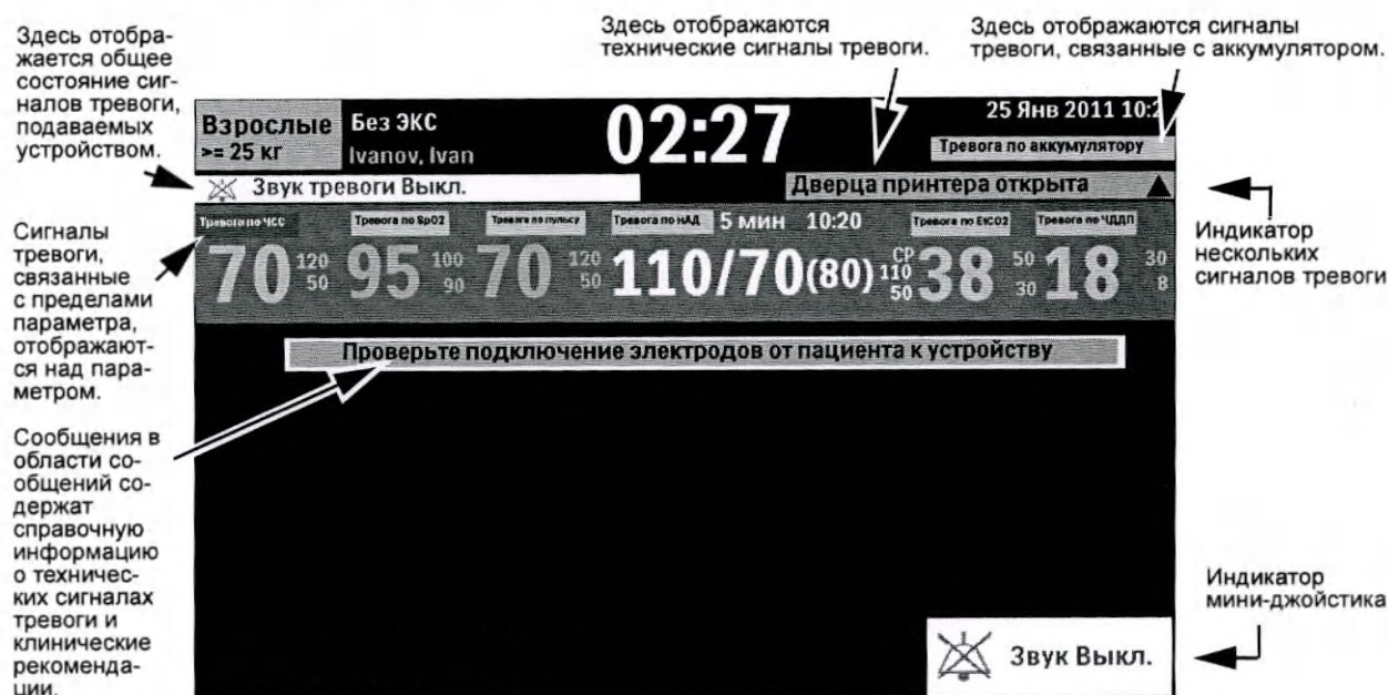
Рис. 35 Области экрана, где отображаются уведомления о сигналах тревоги
