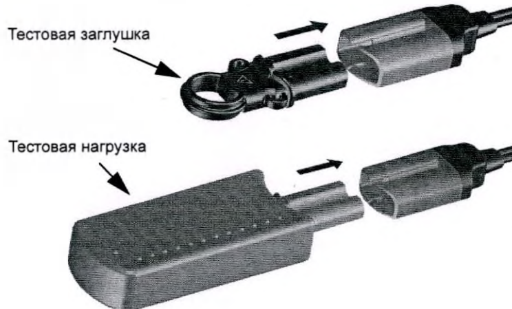
Рис. 21 Подключение тестовой заглушки/нагрузки дефибриллятора
