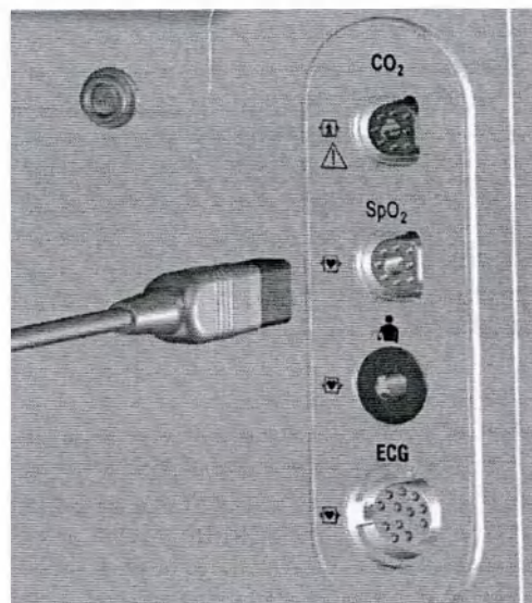
Рис. 9 Подключение кабеля SpO 2
