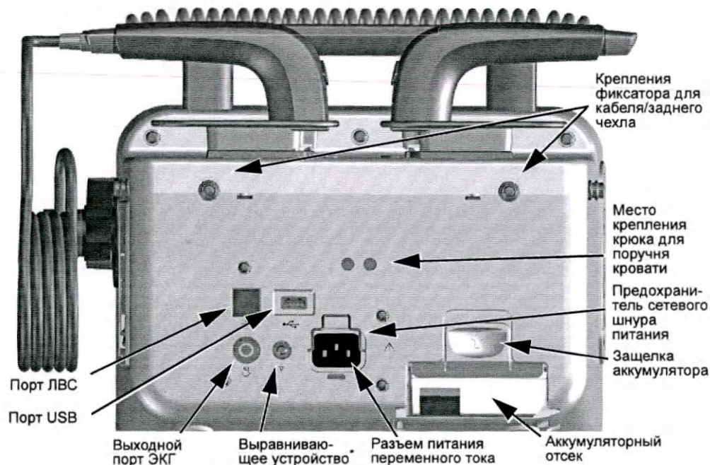
Рис. 15 Задняя панель
