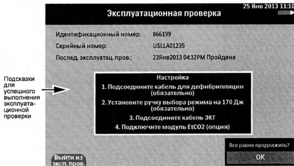
Рис. 73 Экран настройки эксплуатационной проверки
