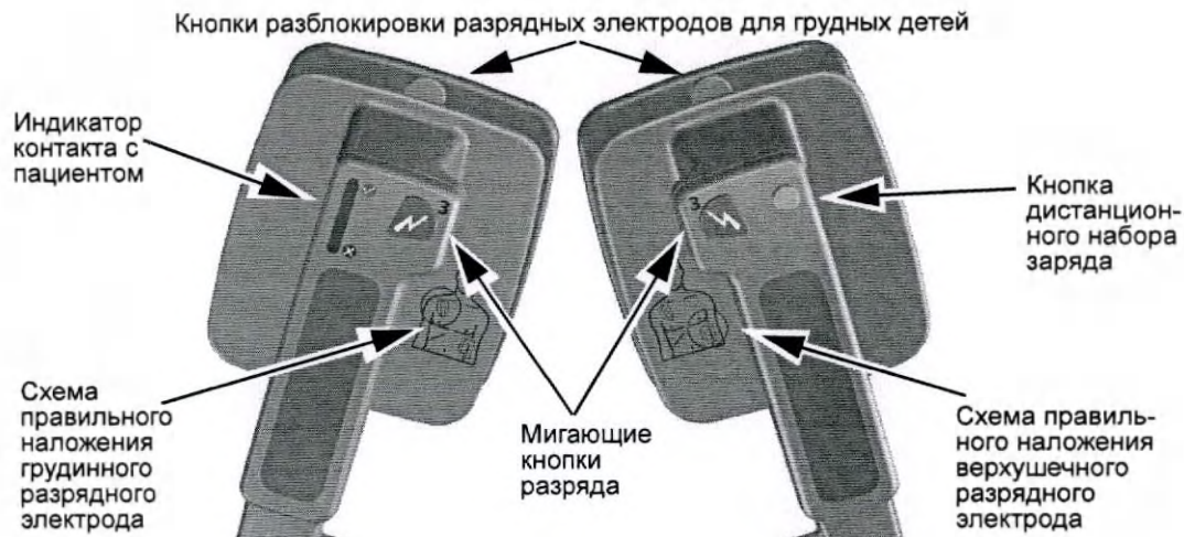
Рис. 13 Характеристики наружных разрядных электродов: 989803196431
