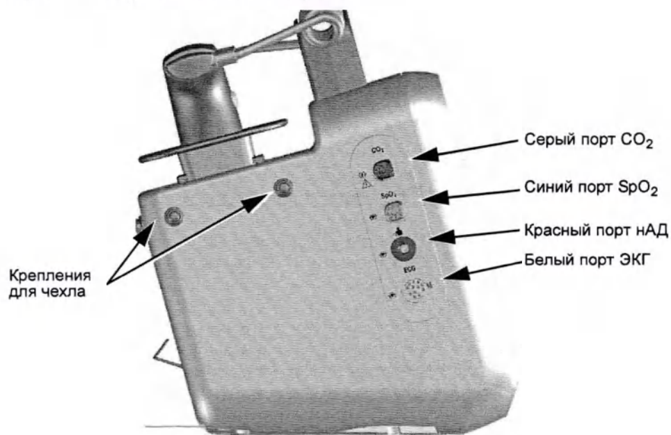
Рис. 6 Сторона для мониторинга
