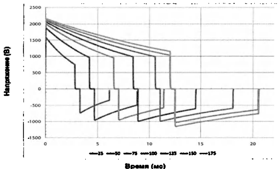
Бифазный импульс Philips Smart, 200 Дж при 25-175 Ом
