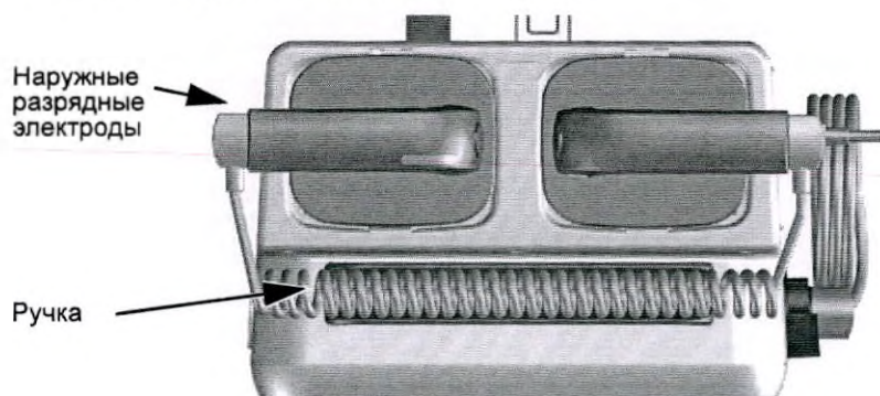
Рис. 11 Верхняя панель
