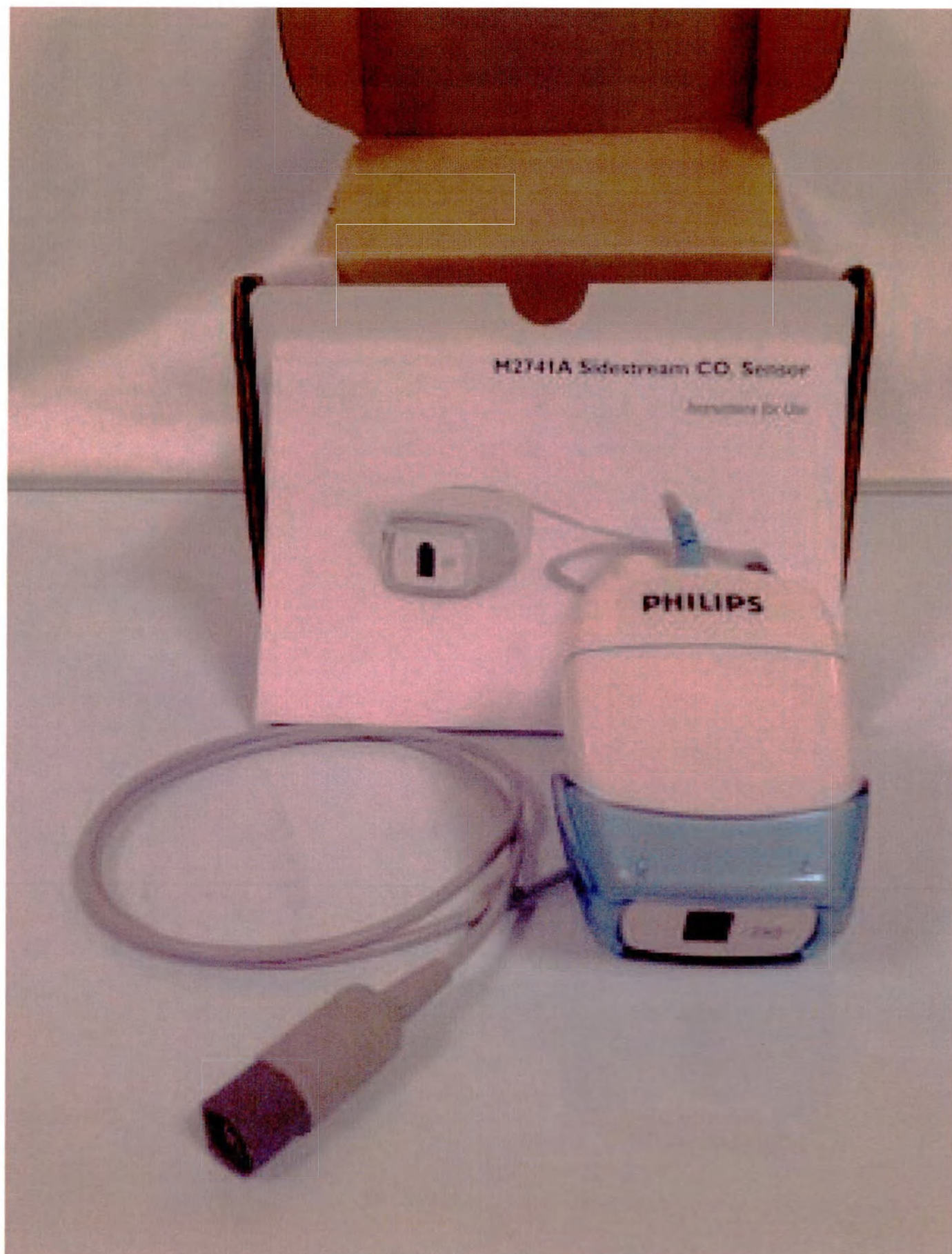
33. Датчик CO 2 для измерений в боковом потоке.
