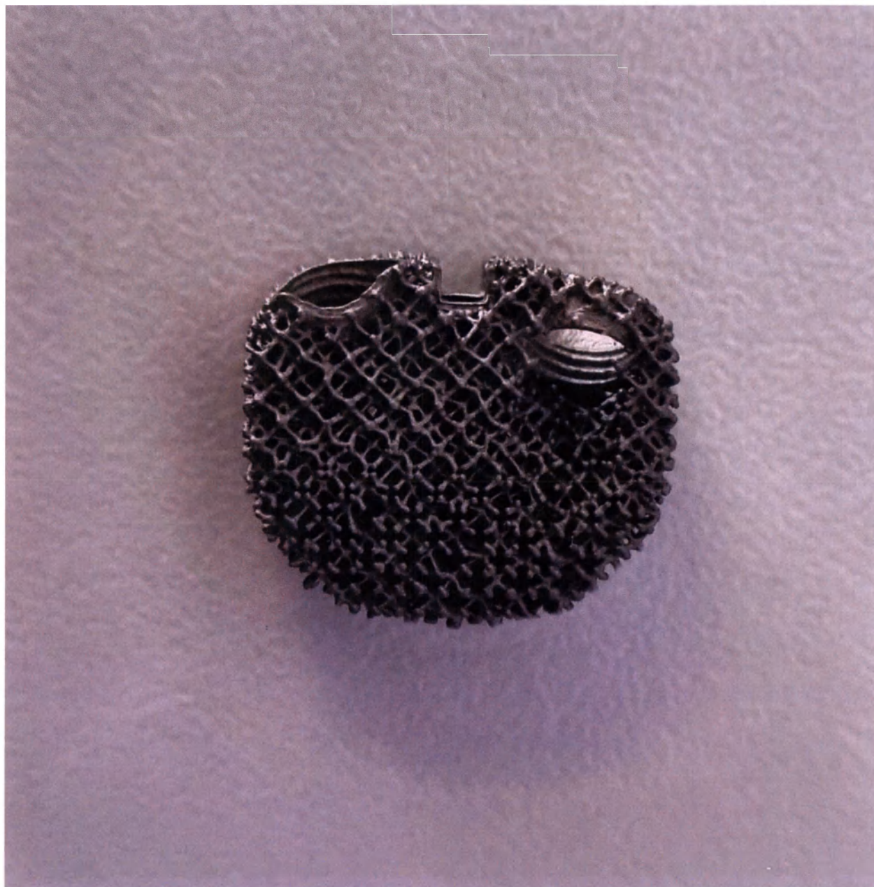
1.4 Кейдж межтеловой пористый 12x16 (от 5 мм до 12 мм с шагом 1 мм и углами 0°, 4°, 8°)
