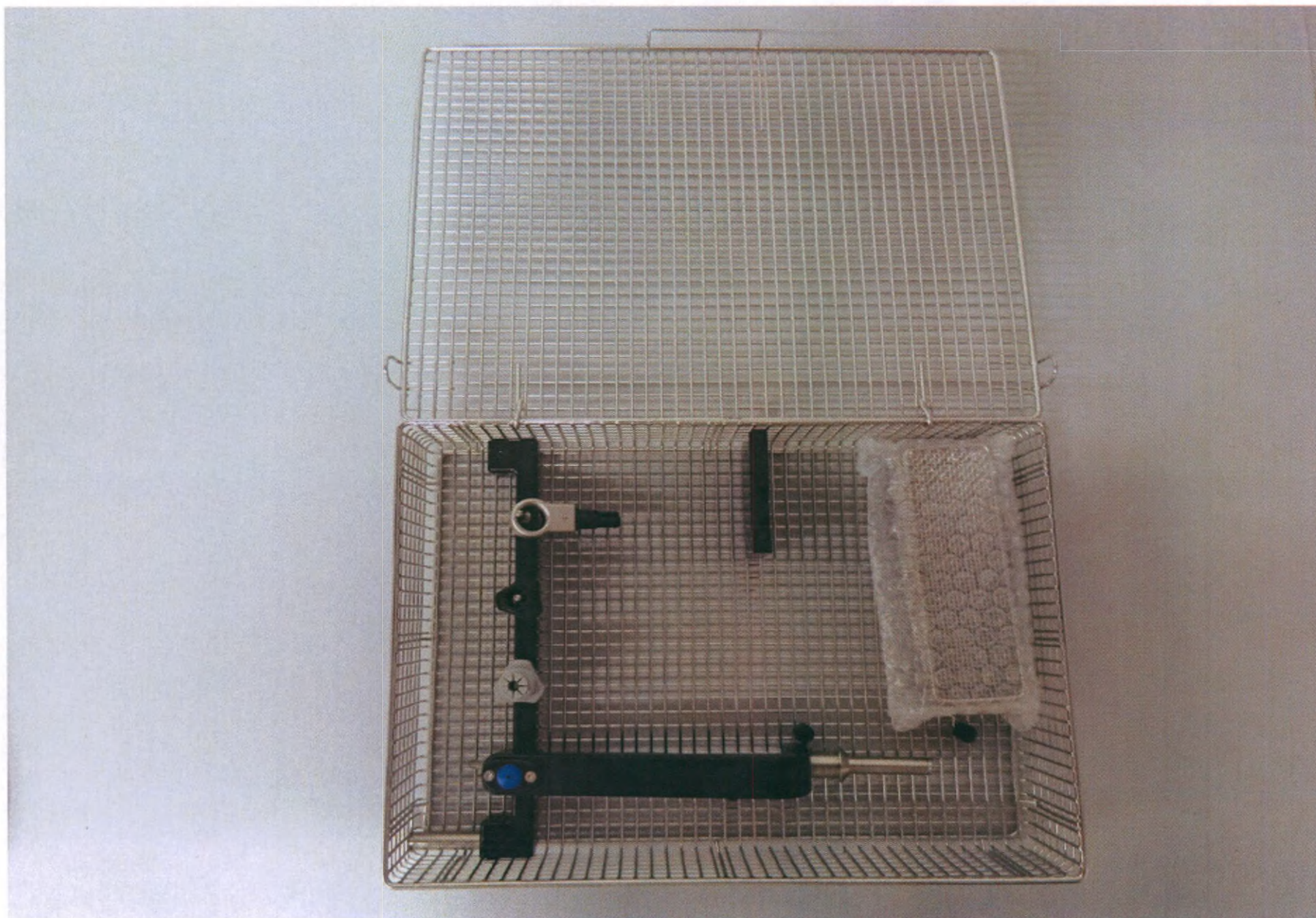
3.Корзина для стерилизации, в составе (общий вид)
