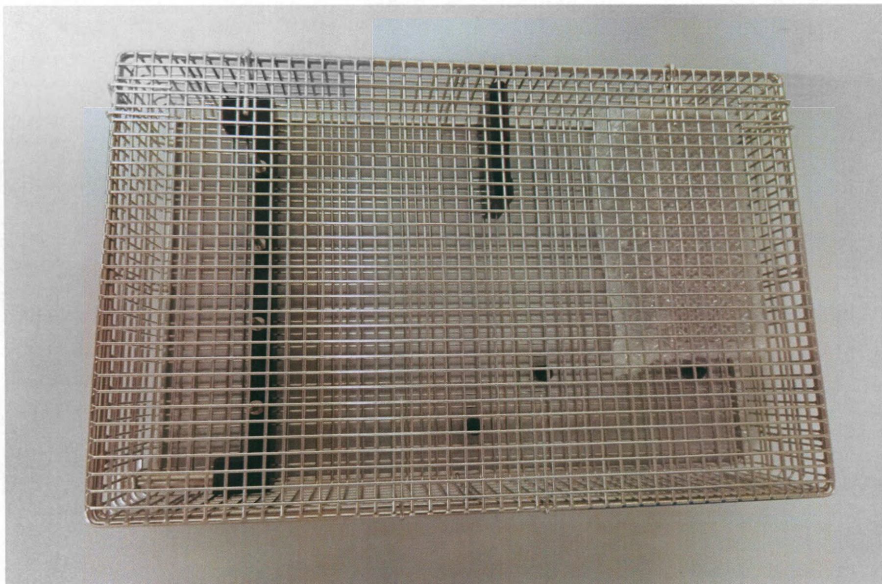
3.1. Корзина для стерилизации (общий вид)
