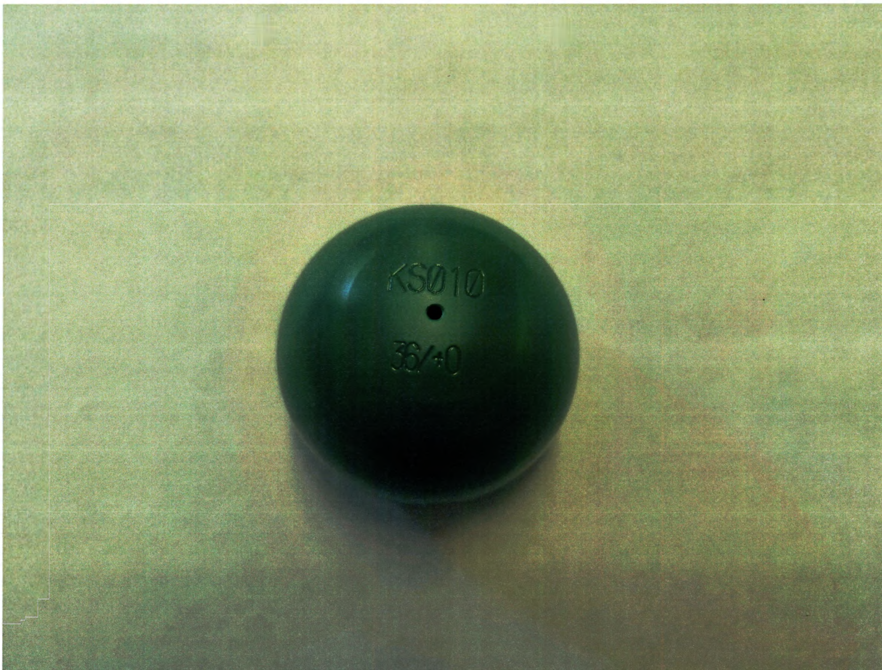
Рис. 10. Головка примерочная KS010, под имплантат головки бедренной типоразмера 36/+0; цвет зеленый Имеют идентичный вид, отличаются размерным рядом: Головка примерочная KS010, под имплантат головки бедренной типоразмеров: 36/-3.5, 36/+0, 36/+3.5, 36/+7
