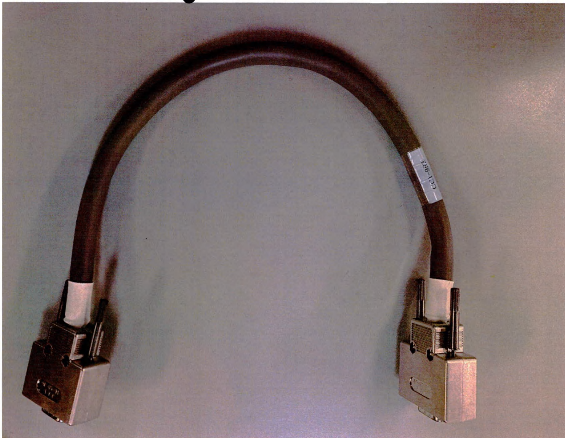
Кабель соединительный, в исполнении CC1-9R3
