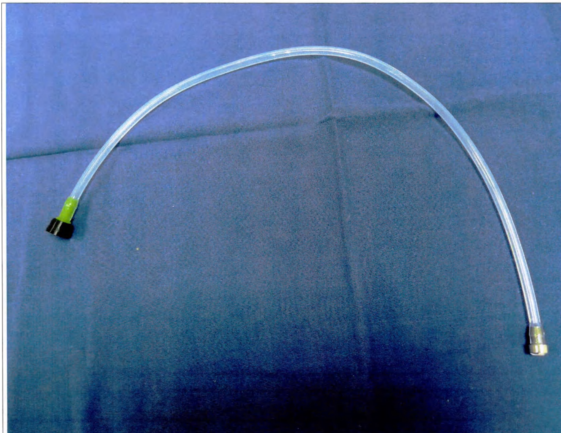
Рис. 16. Адаптер для аспирационной очистки (МН-856)
