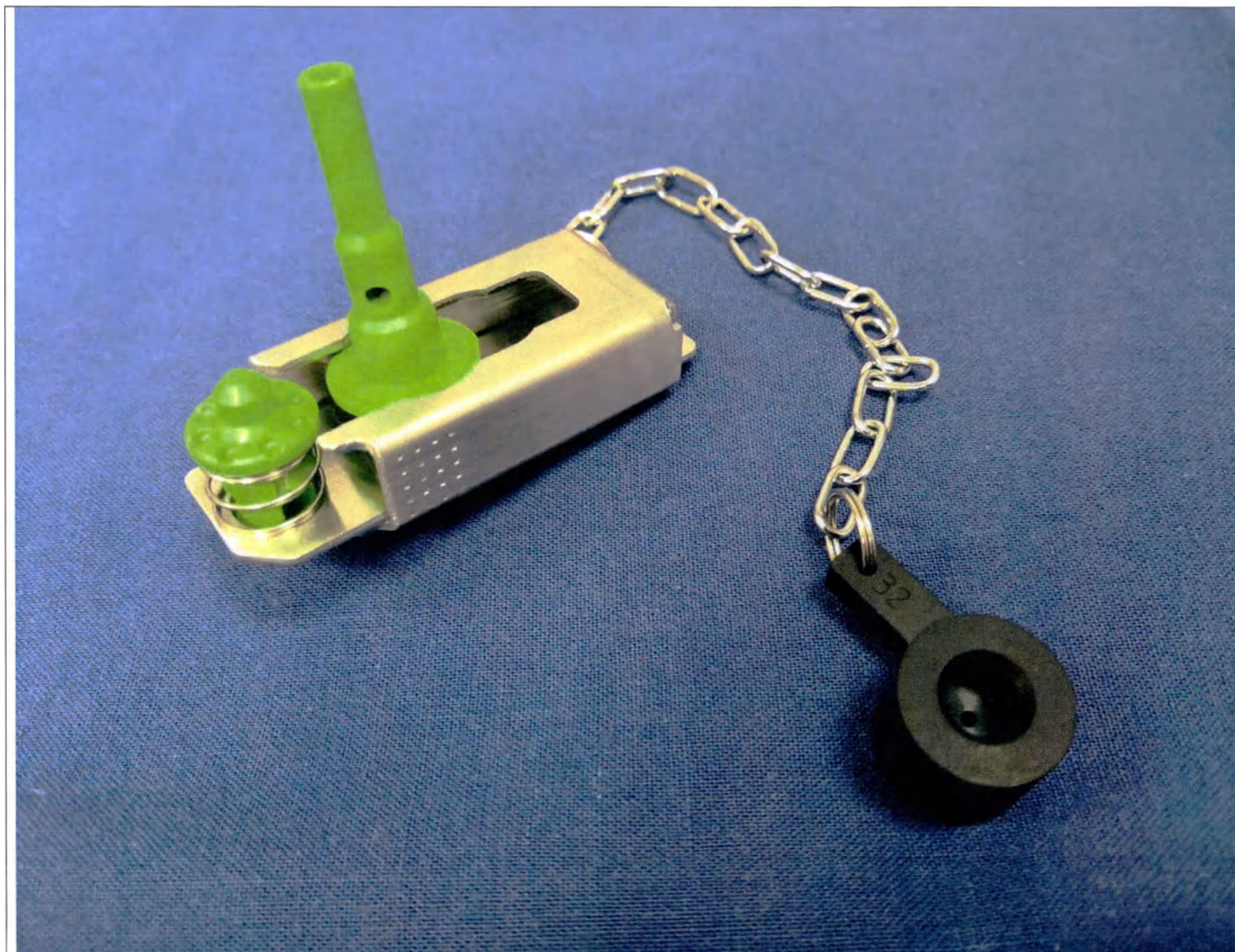
Рис. 13. Заглушка для канала (МН-944)
