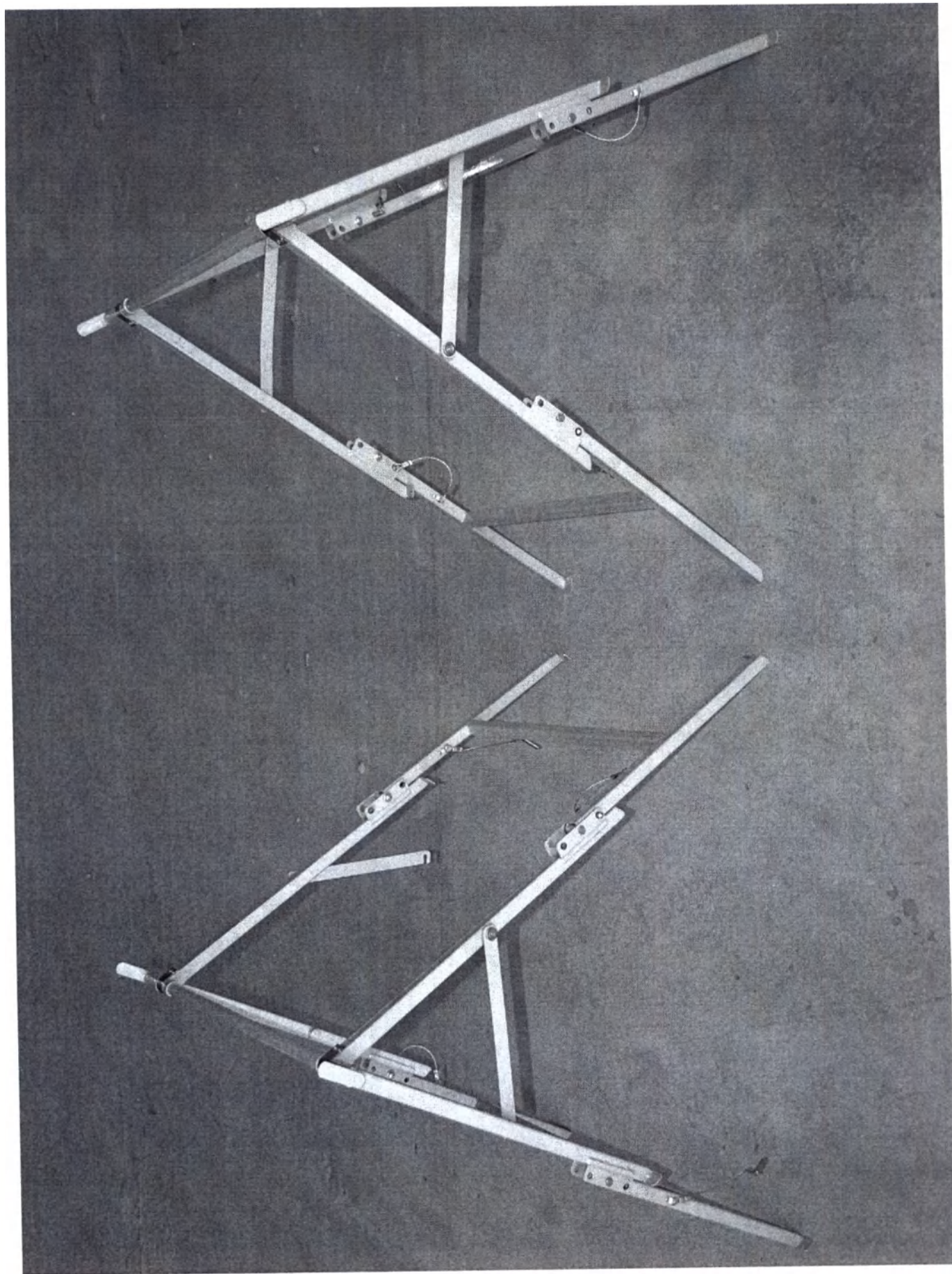
Фотография 25. Подставки складные под носилки ПНС-1 (комплект из 2 шт.). Общий вид (в развернутом состоянии).
