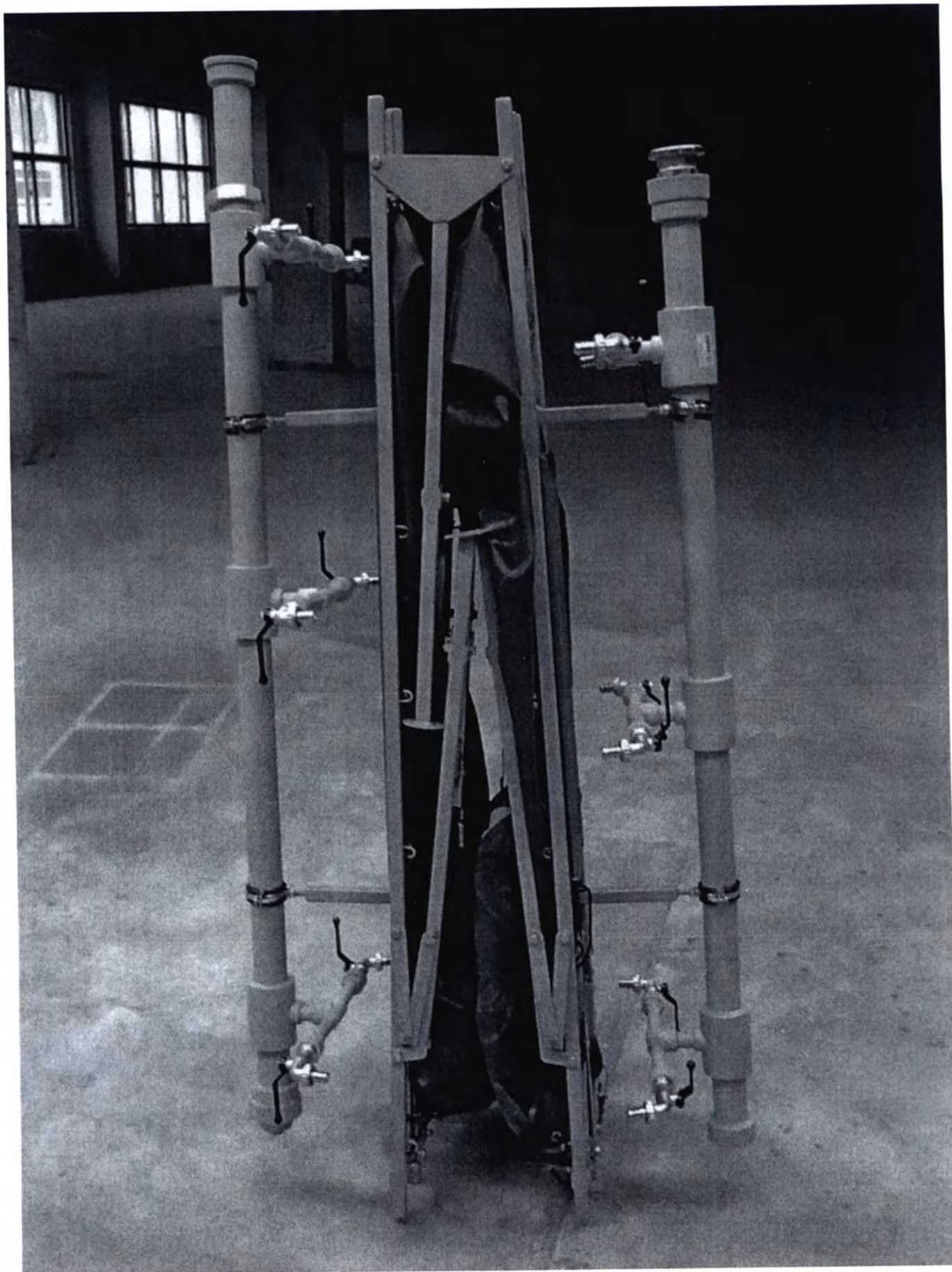
Фотография 17. Умывальник полевой складной УПС-12 (в сложенном состоянии). Общий вид.
