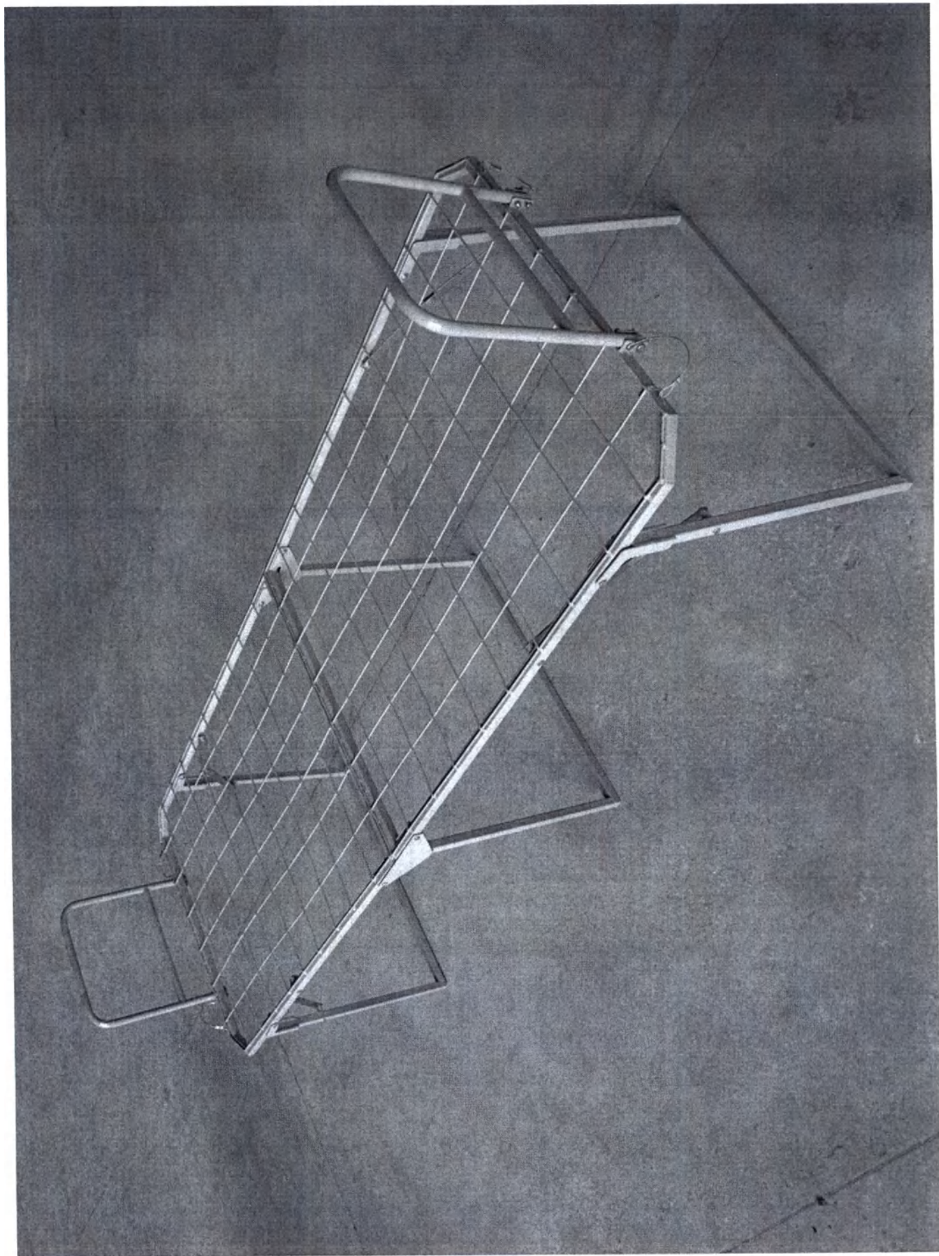
Фотография 1. Кровать складная КС (в развернутом состоянии). Общий вид.
