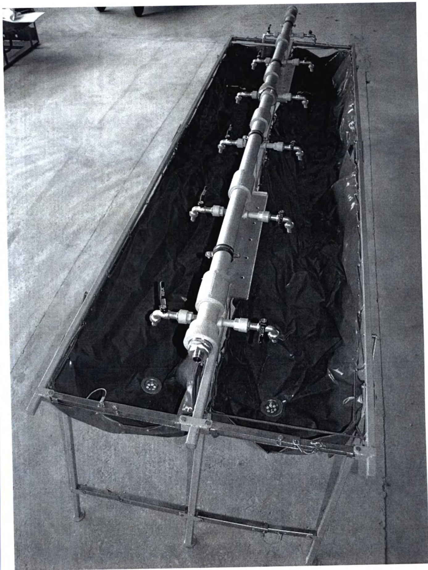
Фотография 16. Умывальник полевой складной УПС-12 (в развернутом состоянии). Общий вид.
