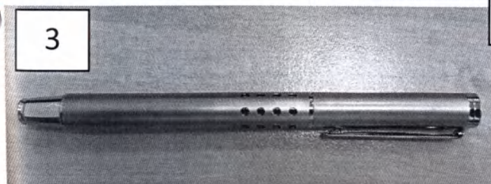
1- шнур питания, 2- вставки плавкие, 3- скалыватель волокна, 4- защитное окно, 5-заглушка внешней блокировки, 6- Инструмент волоконный стерильный многообразный «IPG Surgical Fiber Reusable S» с торцевым выходом, диаметр сердцевины XXX мкм (РУ №РЗН 2019/8729)), 7 – образец маркировки Инструмента волоконного
