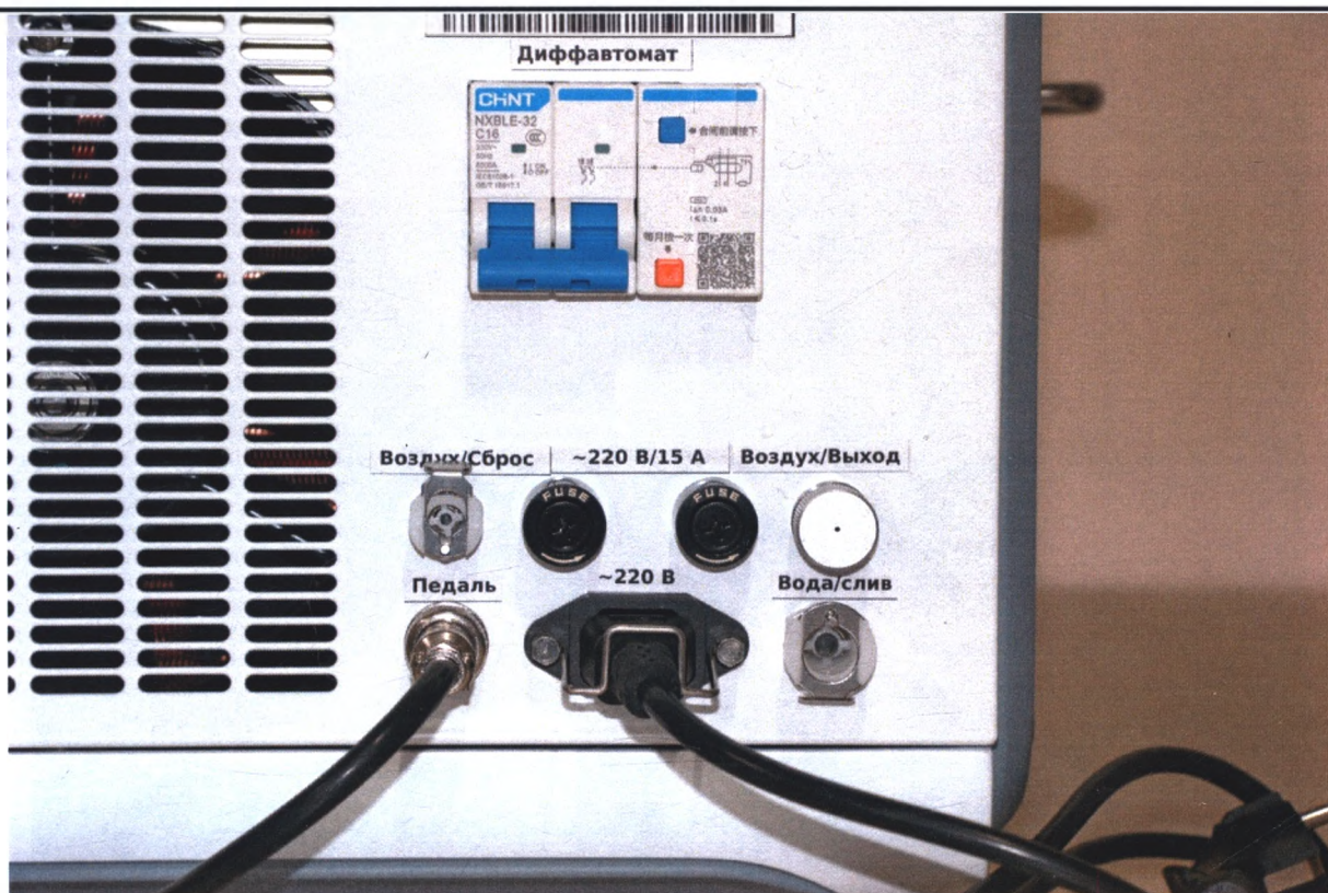
Задняя панель In-Motion D2
