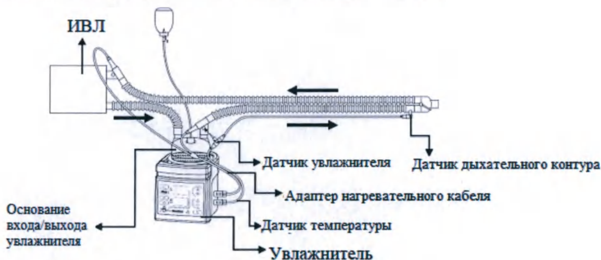
Рис.2 Система дыхательного контура из ненагретой проволоки
