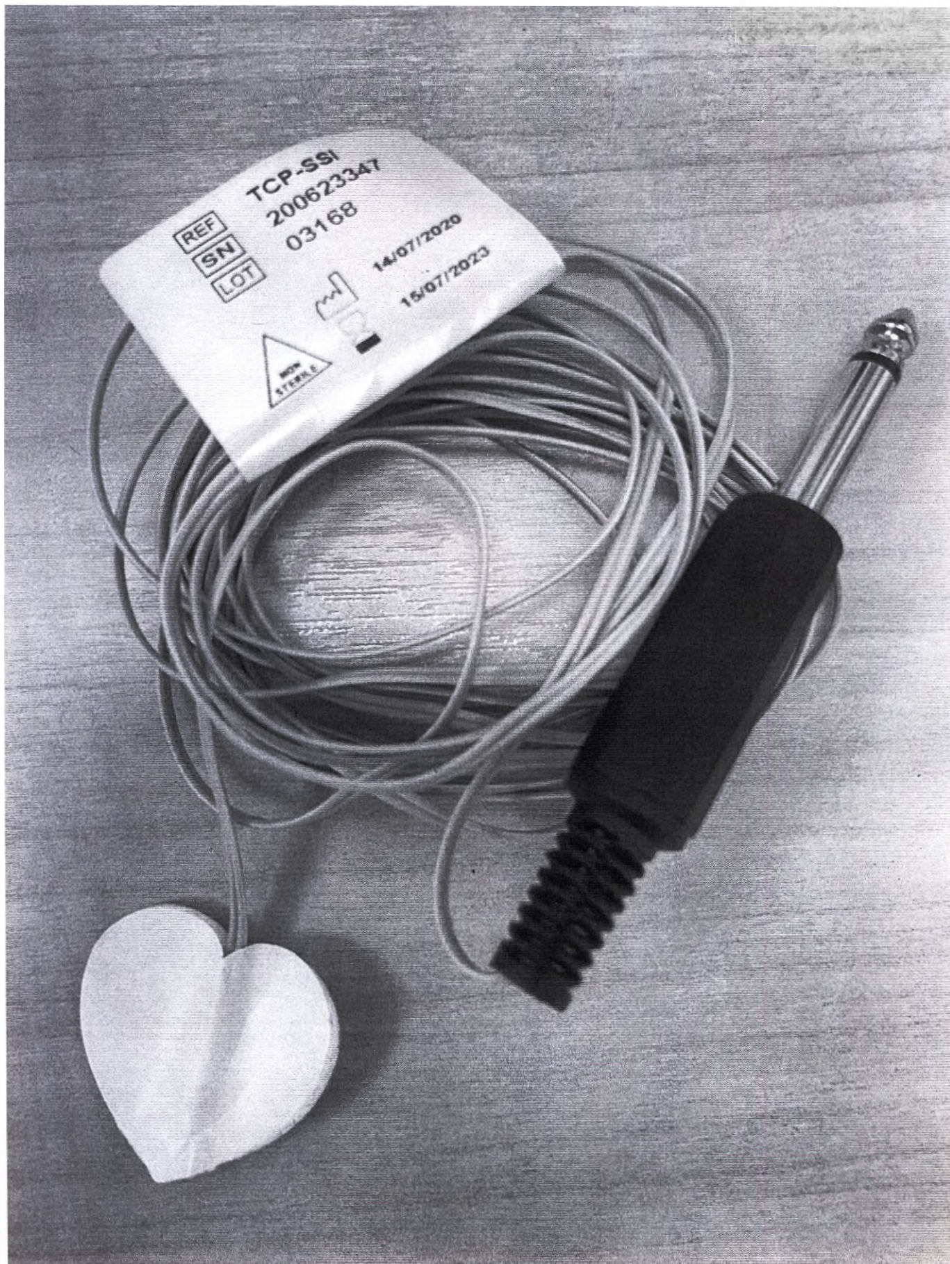
Одноразовый датчик температуры накожный для детей TCP-SSI
