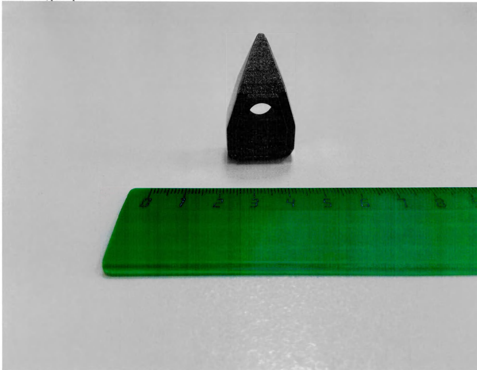
Вставка бедренная Legion, Ti6Al4V, дистальная, на примере варианта исполнения Вставка бедренная Legion, Ti6Al4V, дистальная, размер 4 – 10 мм
