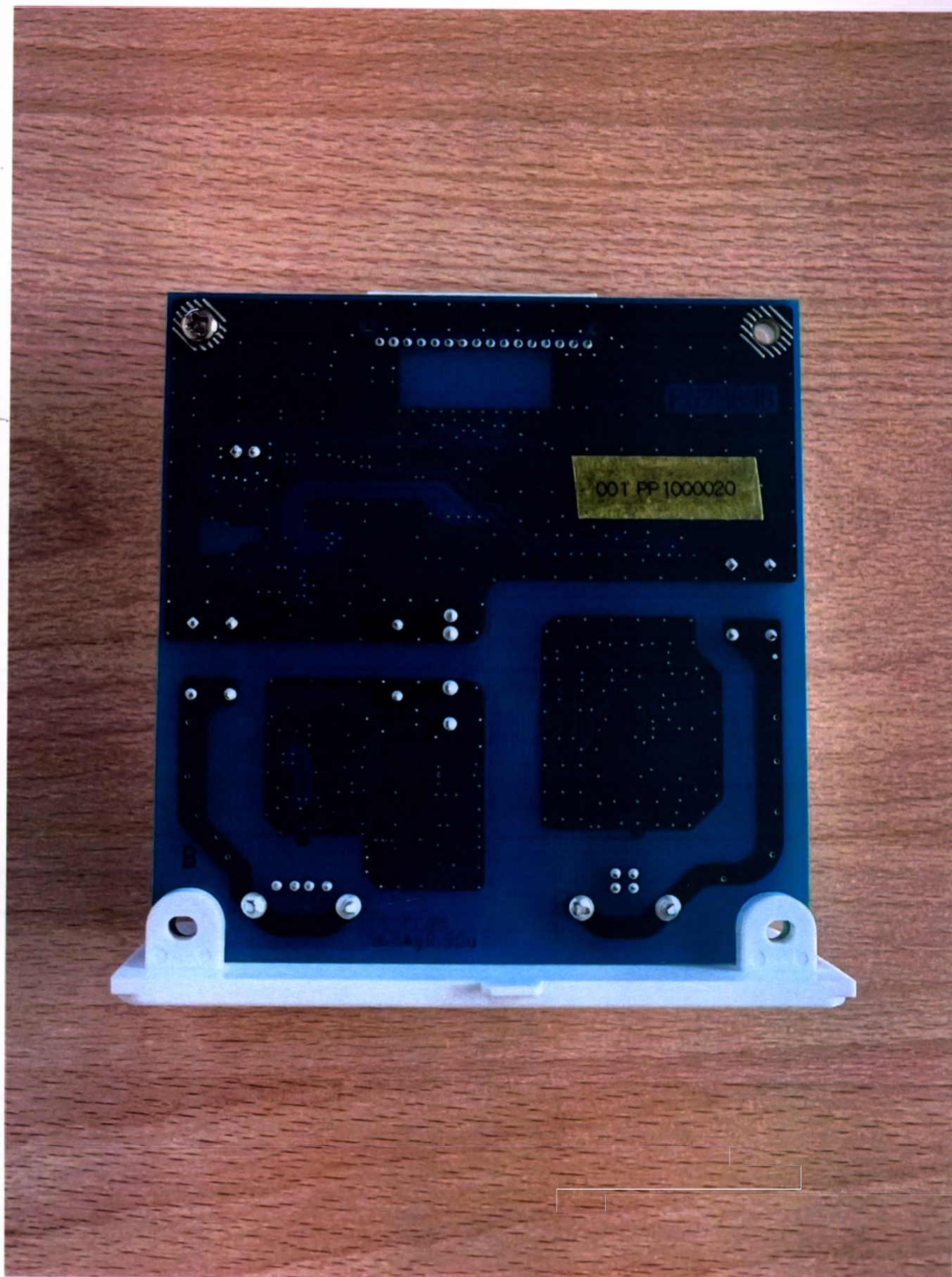
Модуль с разъёмами USB типа А и USB типа В. Вид сзади
