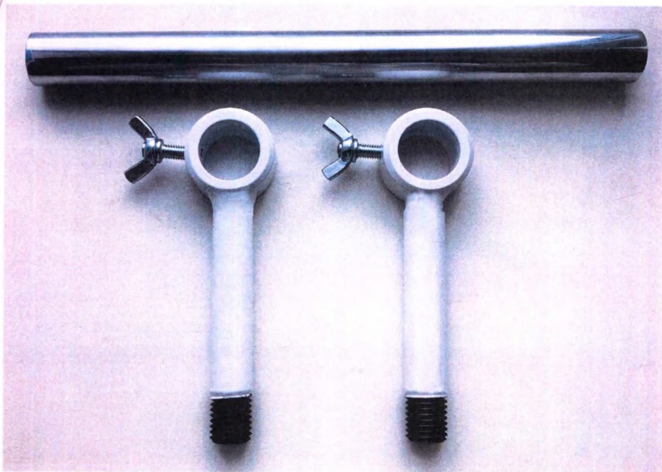
Общий вид Захват для переноса стерилизатора (1 комплект: ) - рым-болт – 2 шт - труба – 1 шт
