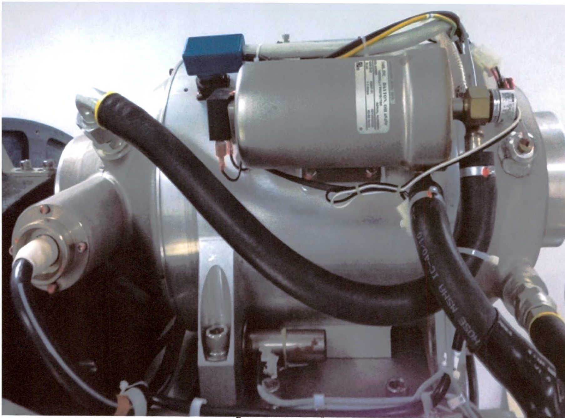
Рентгеновская трубка
