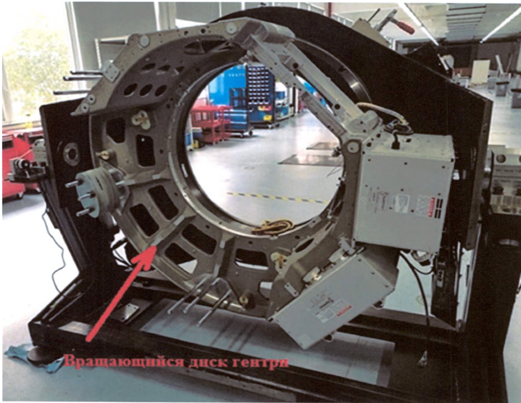
Вращающийся диск гентри
