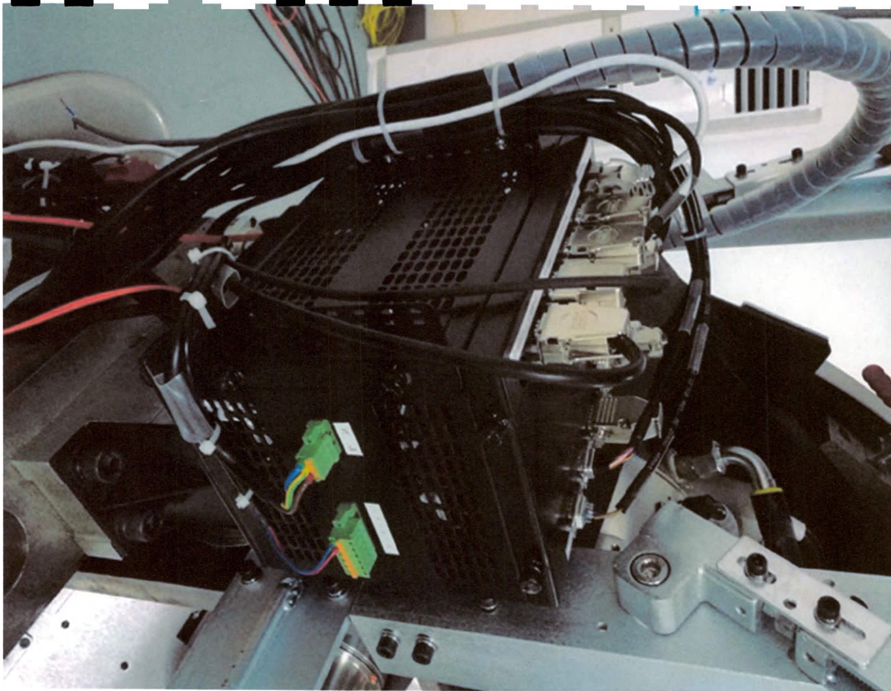
Стационарный блок управления сканированием
