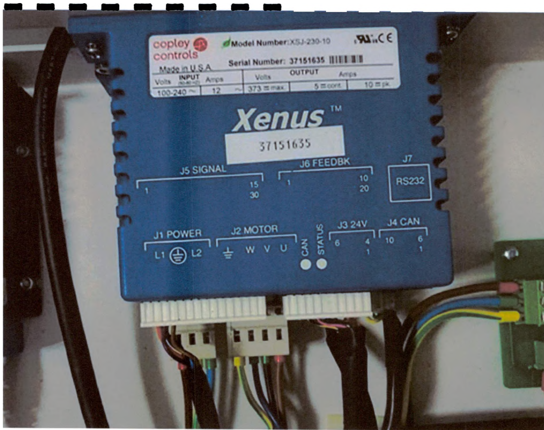
Блок управления вертикального движения стола
