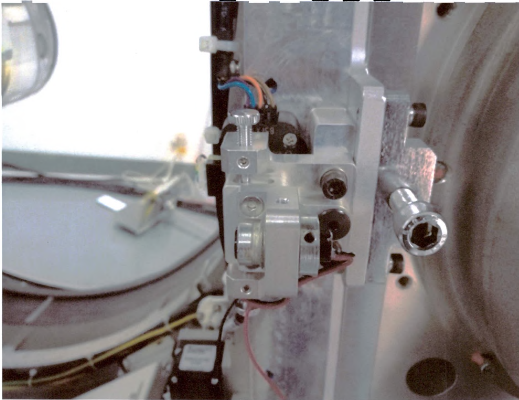
Лазерное устройство позиционирования
