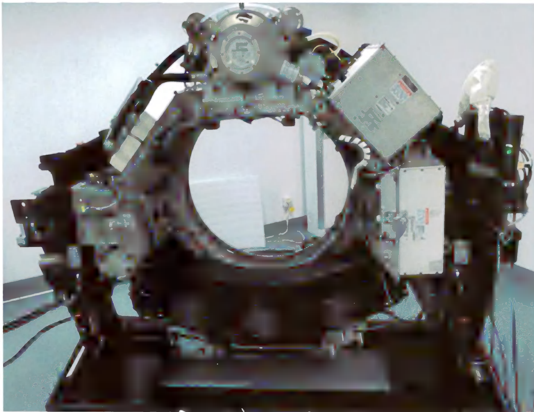
Гентри в сборе
