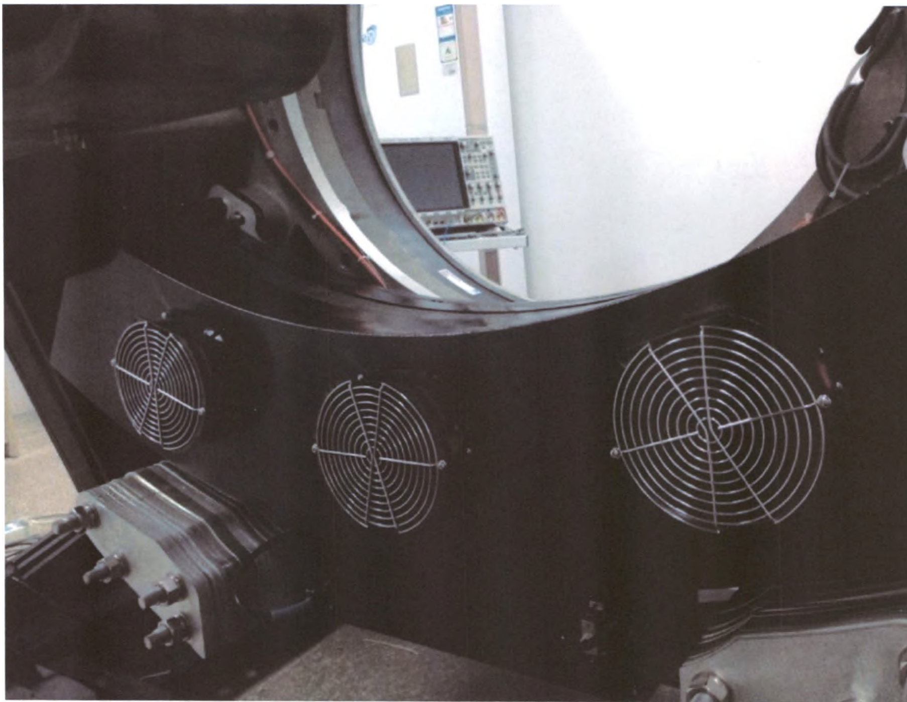
Блок детекторов
