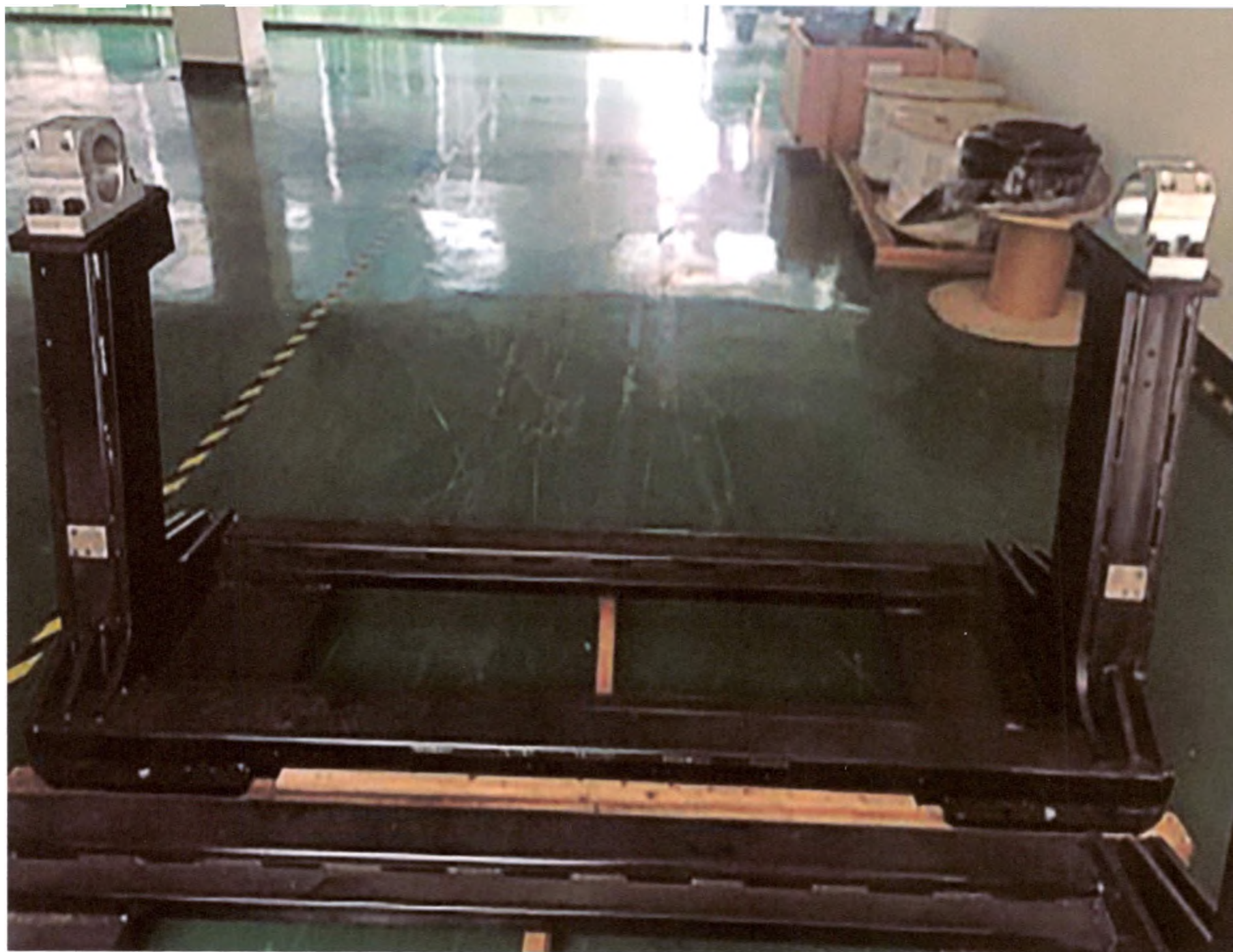
Рама гевтри
