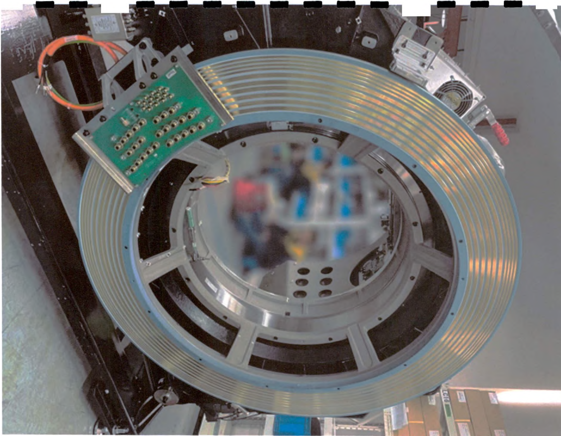
Контактное кольцо (Модель: 4C0000219)
