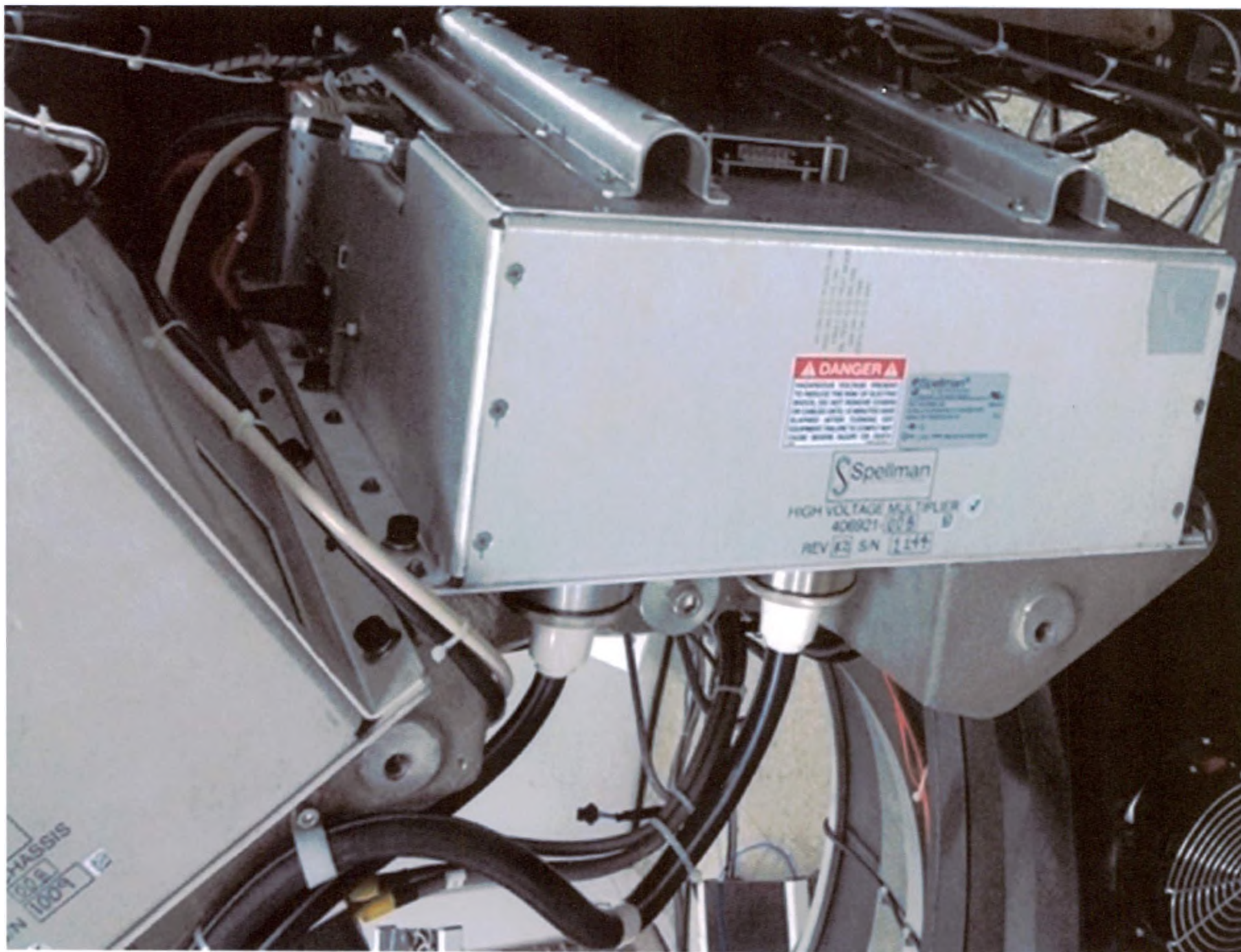
Генераторное устройство
