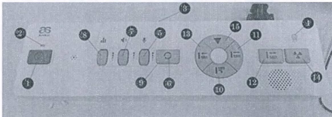
Рисунок 34 Блок управления со встроенной системой интерком
