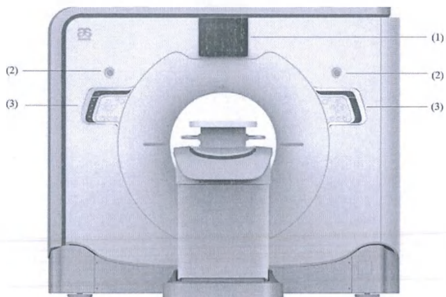
Рисунок 21 Гентри (вид спереди)
