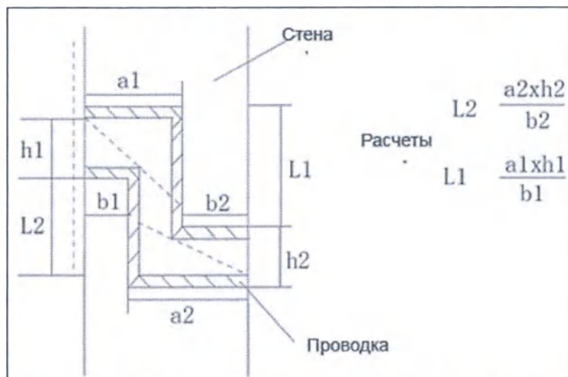
Рисунок 3 Метод S-формы свинцовой изоляции
