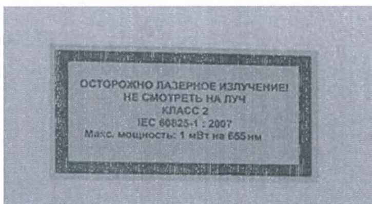
Рисунок 20 Классификация лазера
