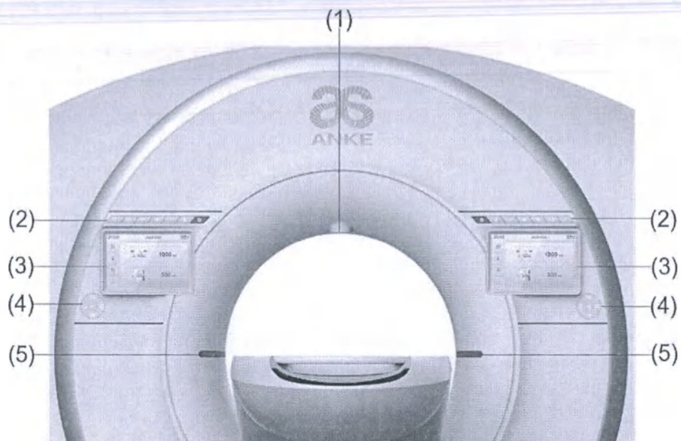
Рисунок 22 Гентри (вид спереди)
