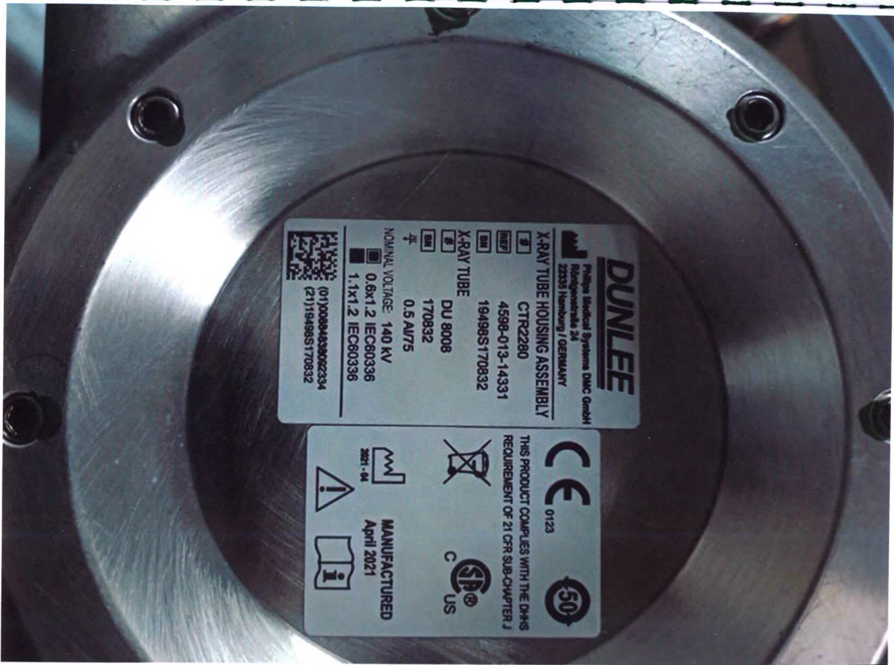
Маркировка рентгеновской трубки (для модели ANATOM 64 Precision)
