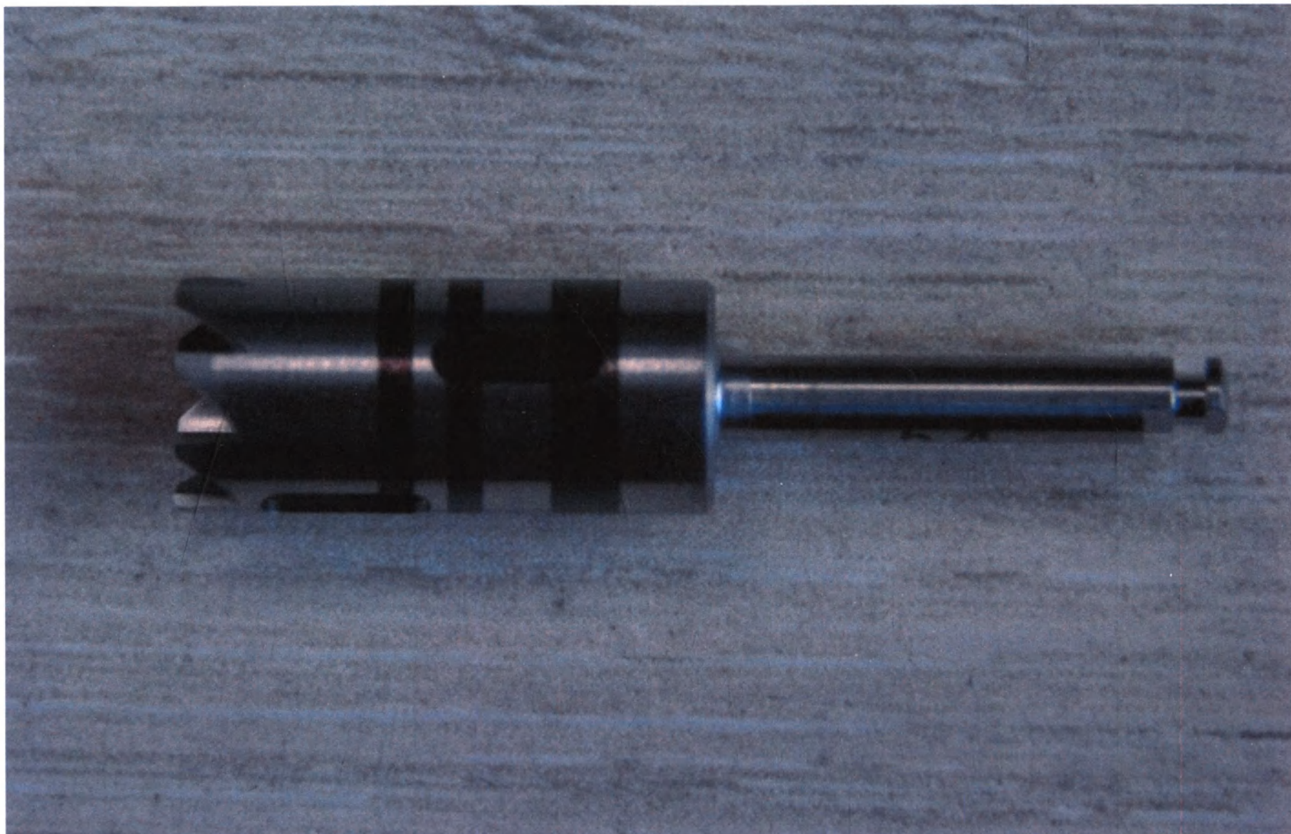
Трепанационное сверло 5.4, 6-13 мм (Trephine Drill 5.4, 6-13 mm)
