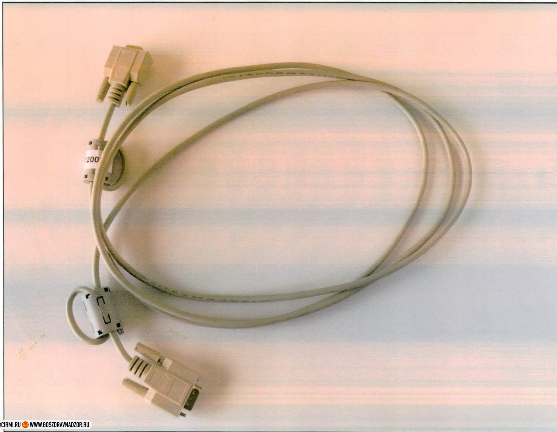
Кабель RS-232 (Кабель для соединения компьютера с анализатором)
