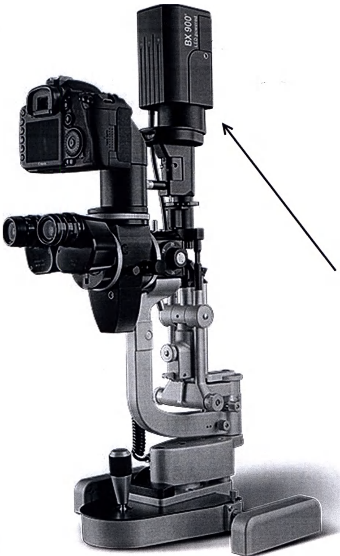
Видеосистема для подключения к щелевой лампе
