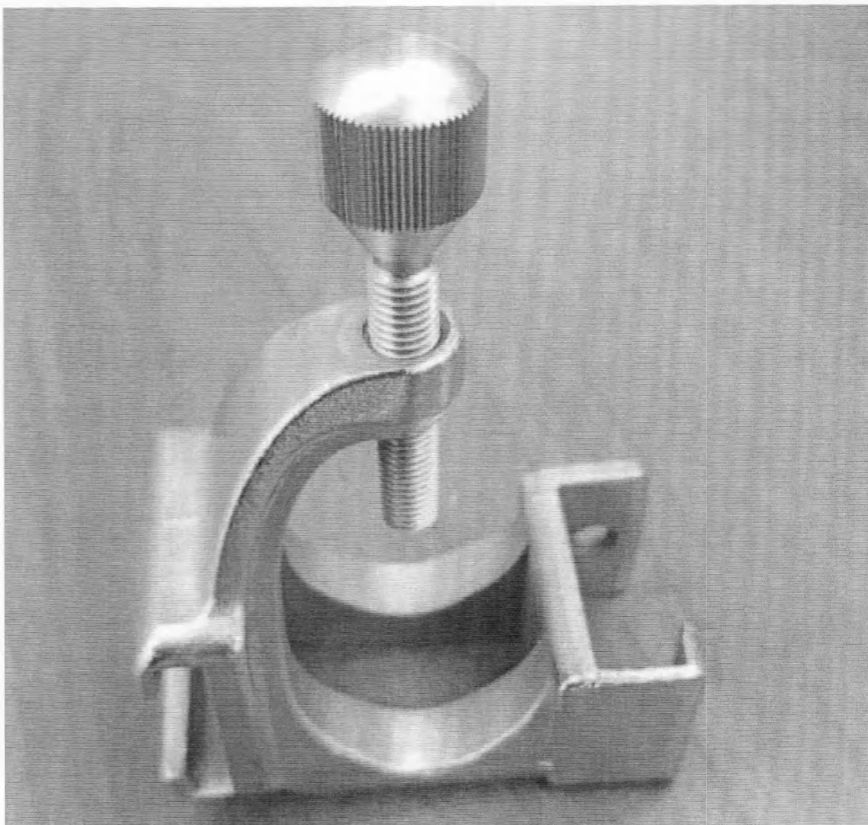
Рисунок 11 – Кронштейн 3150.17000000
