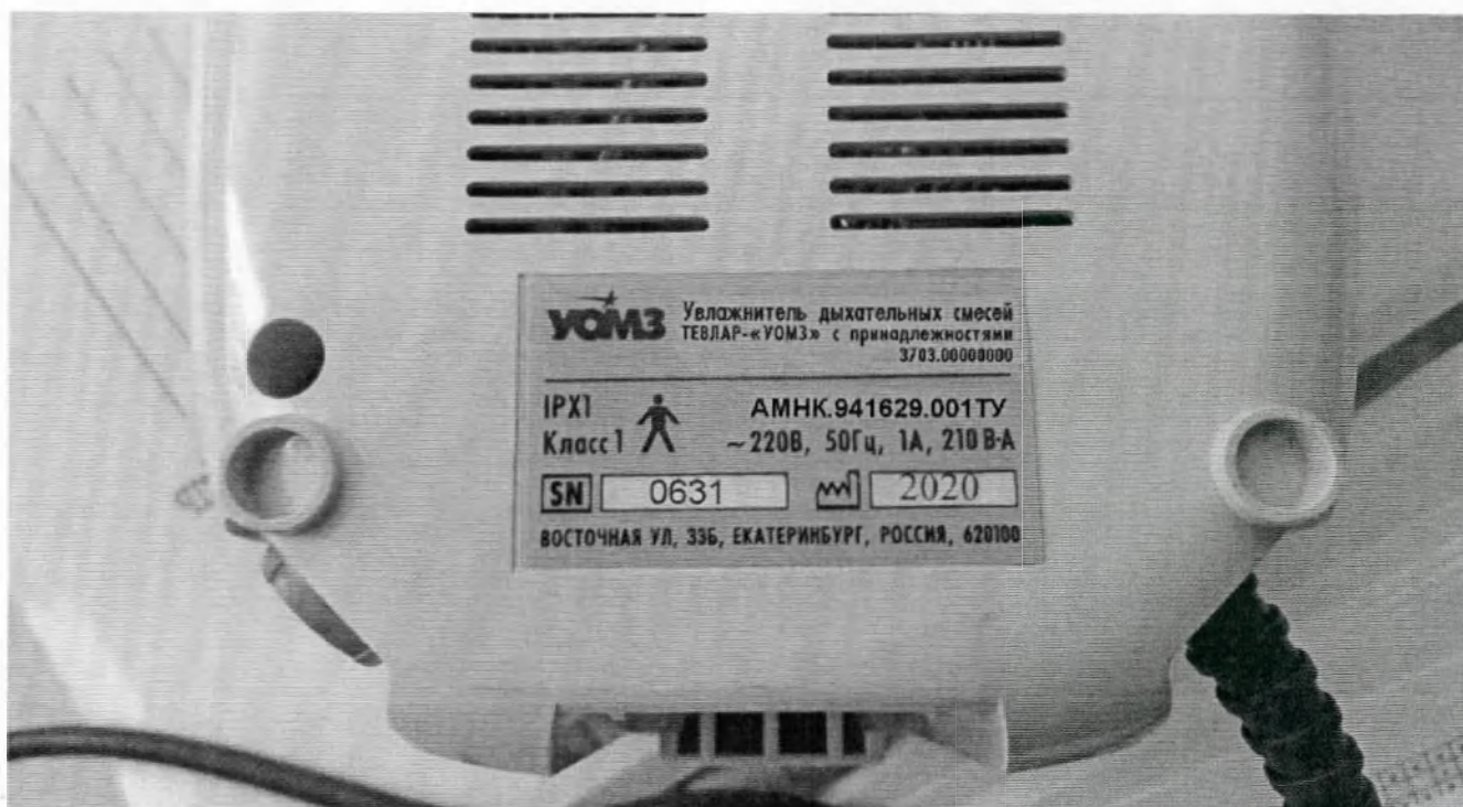
Рисунок 6 – Блок управления 3703.01100000, маркировка
