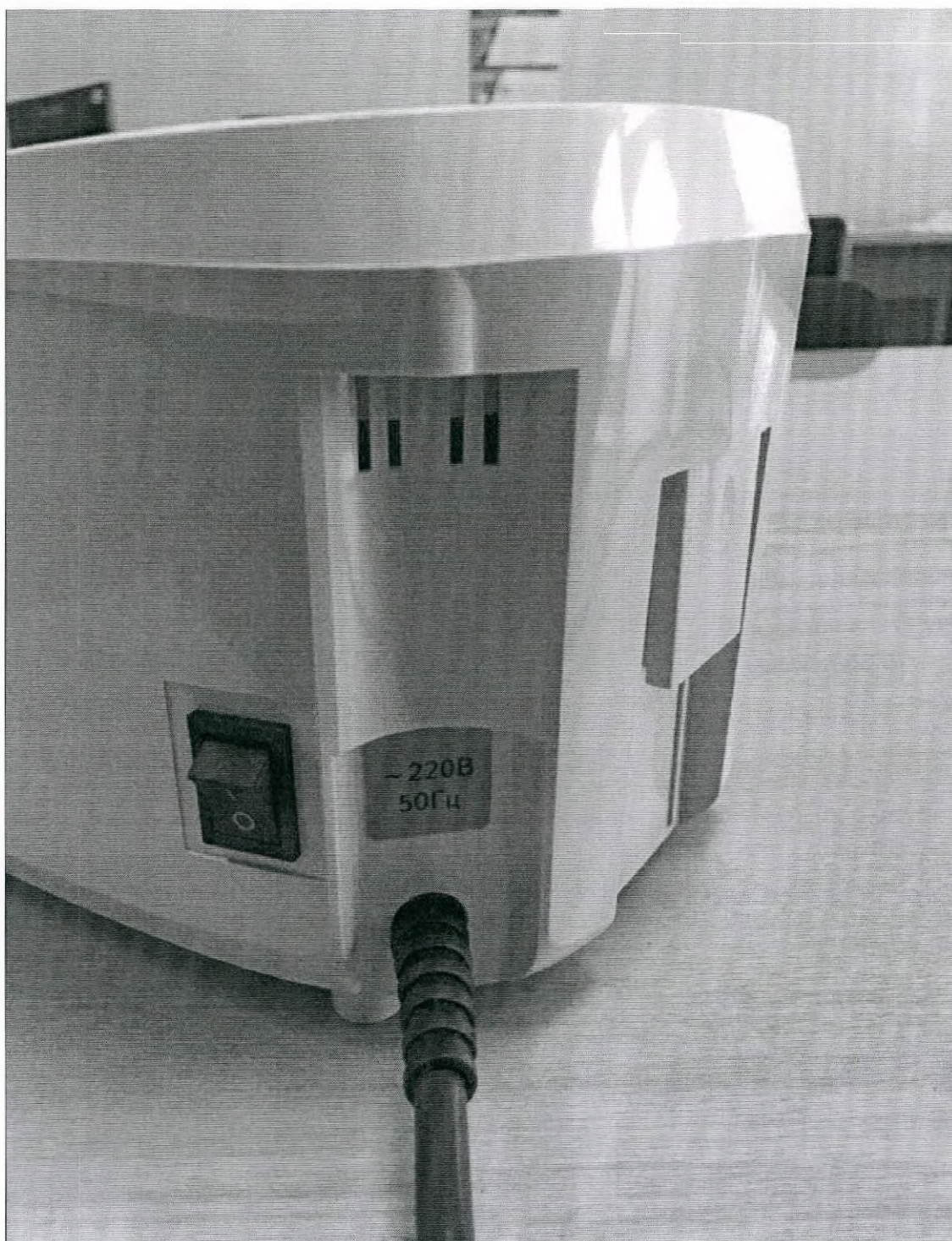
Рисунок 3 – Блок управления 3703.01100000, маркировка
