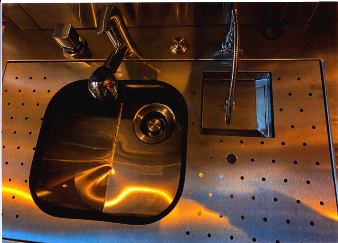
Рисунок 5 – Перфорированная съемная панель с вырезом под раковину для рабочей жидкости, без выреза под перфорированный лоток («Стол врача для работы с тканевым материалом для морфологических исследований TANARTIS®, с принадлежностями «Meridian VI»)
