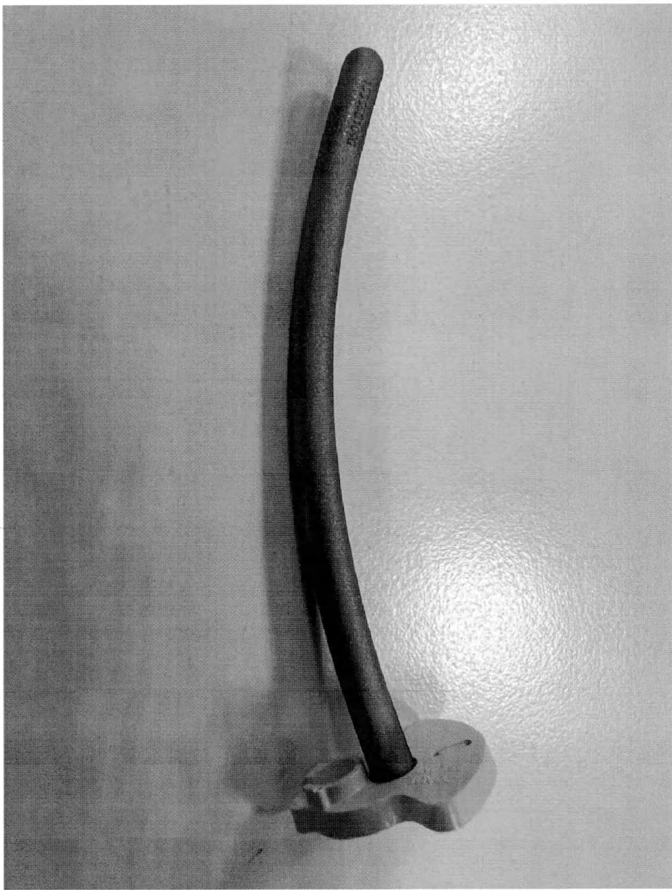
Рисунок 79. Стержень изогнутый ROD 5.5 MM CHROMALOY PRE-BENT 90 MM (общий вид)
