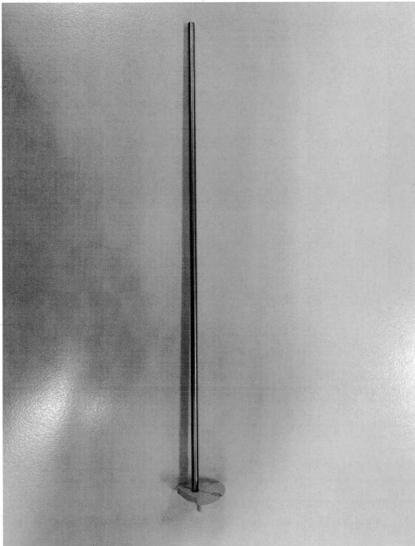
Рисунок 141. Стержень ROD 3.5 MM X 240 MM (общий вид)
