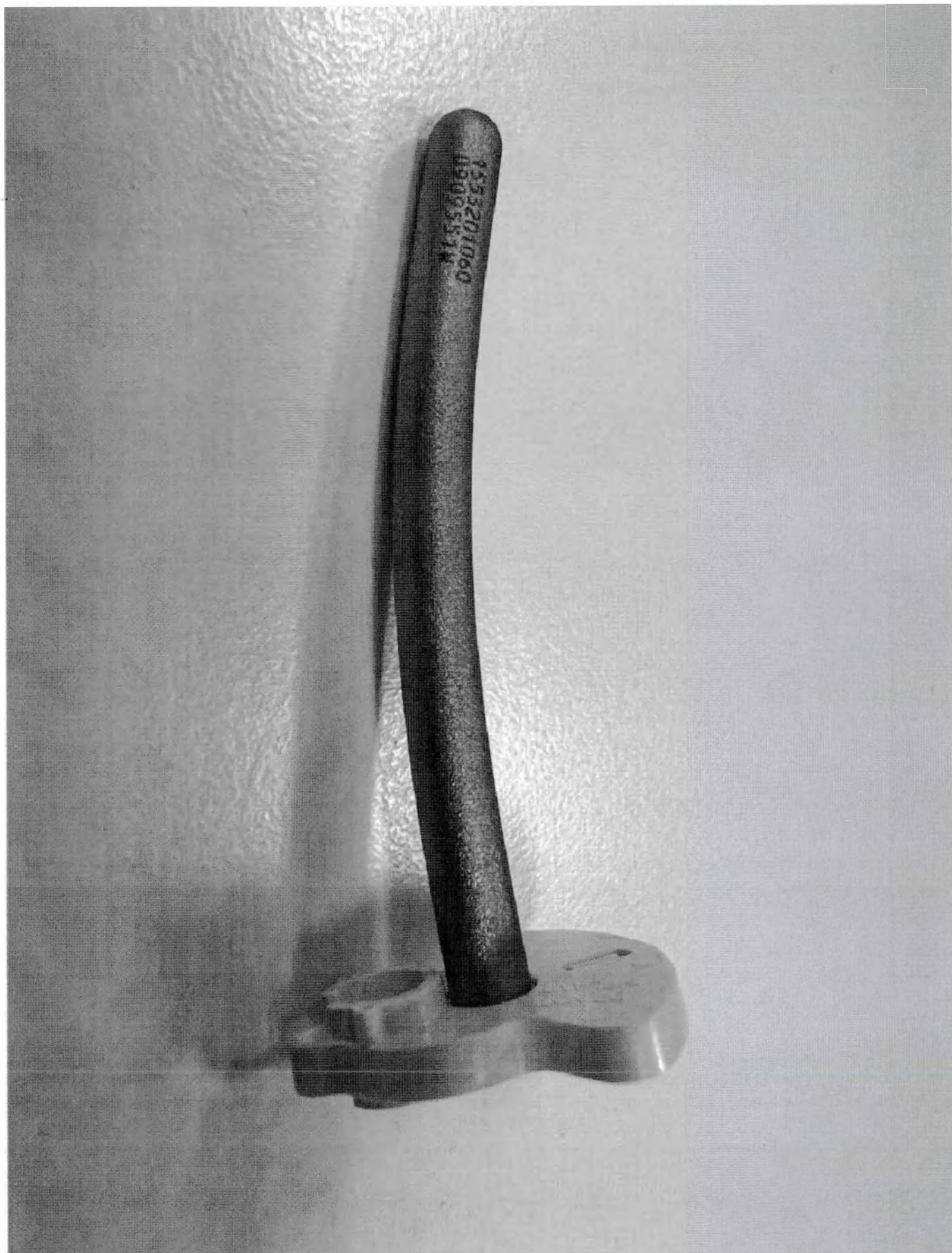
Рисунок 43. Стержень изогнутый ROD 5.5 MM LINED PRE-BEND 60 MM (общий вид)
