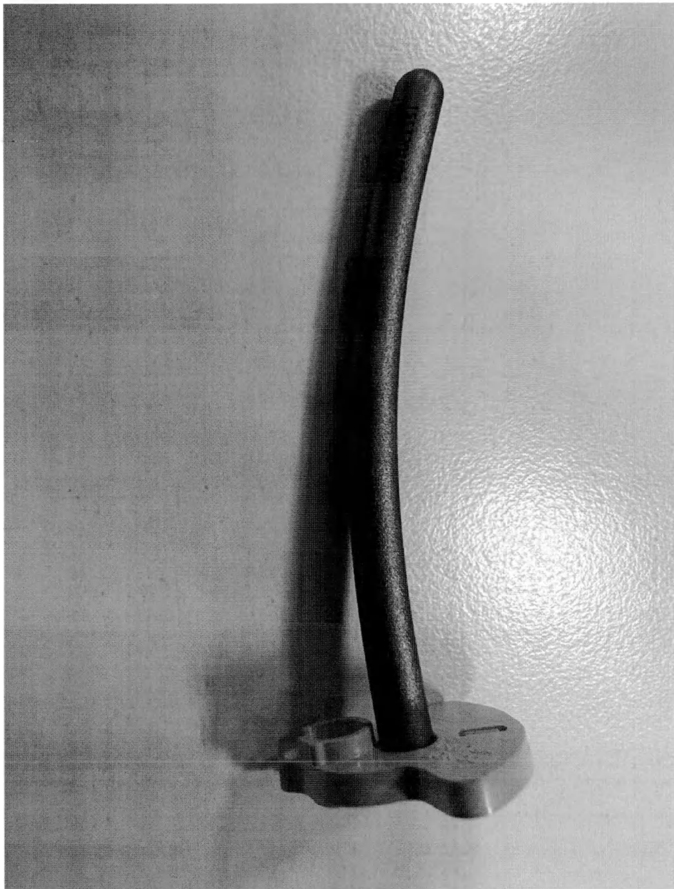
Рисунок 46. Стержень изогнутый ROD 5.5 MM LINED PRE-BEND 70 MM (общий вид)
