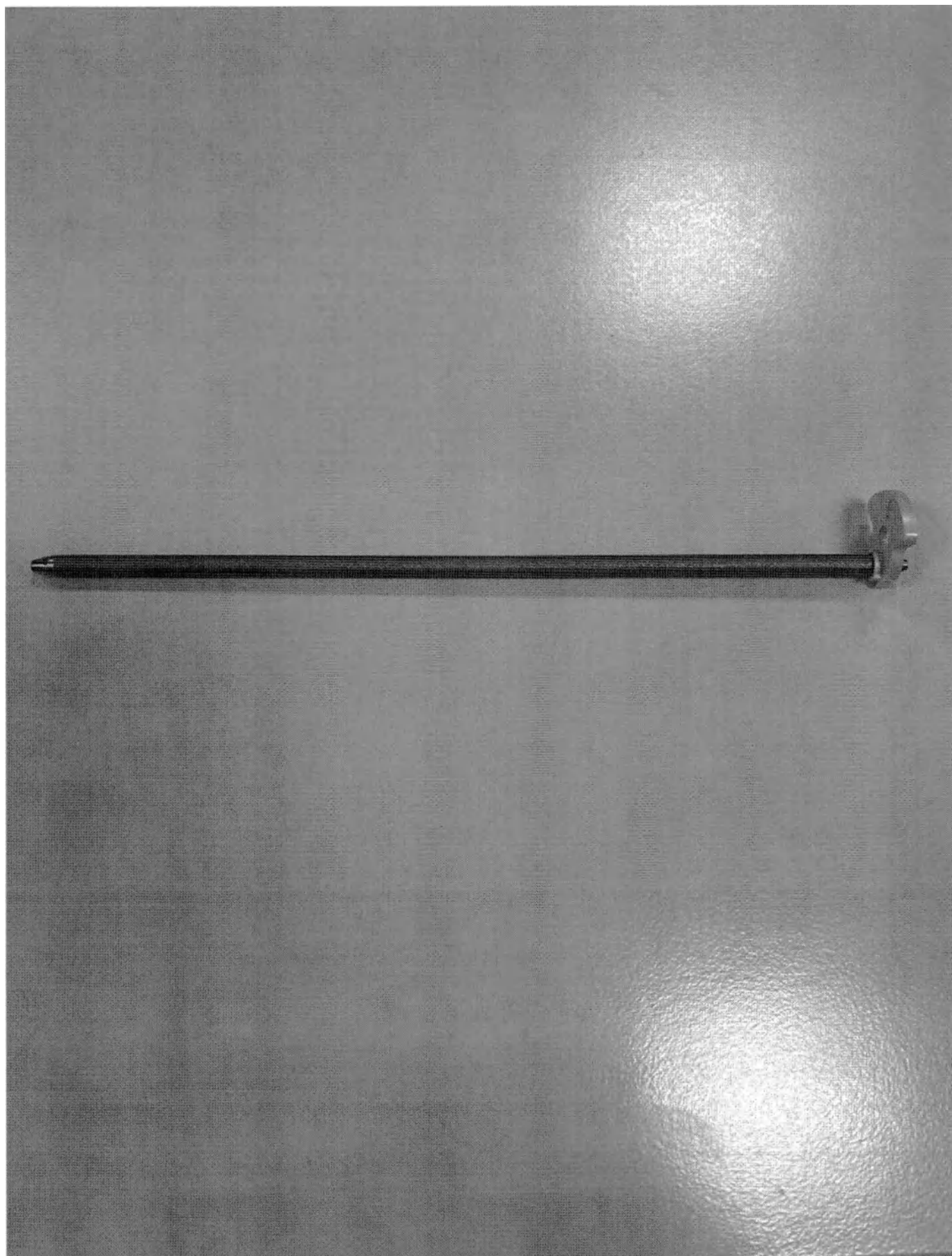
Рисунок 177. Стержень чрескожный прямой ROD 5.5 MM LONGITUDE CHROMALOY 210 MM (общий вид)
