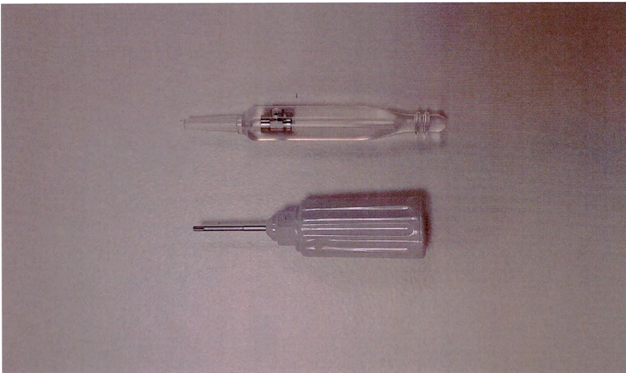
Набор колпачка штекера электрода JenSight – колпачок электрода (сверху) и ключ с тарированным усилием (снизу)
