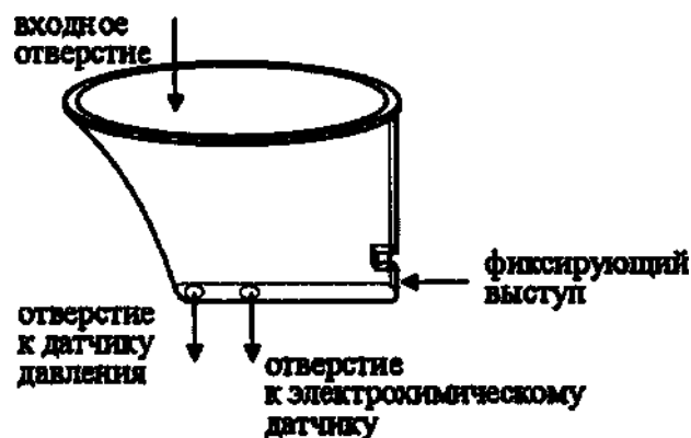
Рисунок 3 – Мундштук-воронка
