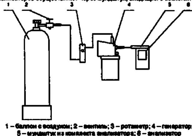
Рисунок 1 – Схема газовой системы при подаче на анализатор ГС от генератора газовых смесей паров этанола в воздухе GUTH модель 10-40
