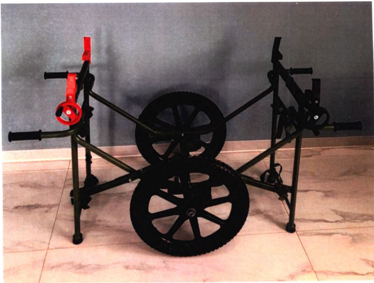
Рама складная с откидными опорами / колеса одинарного типа
