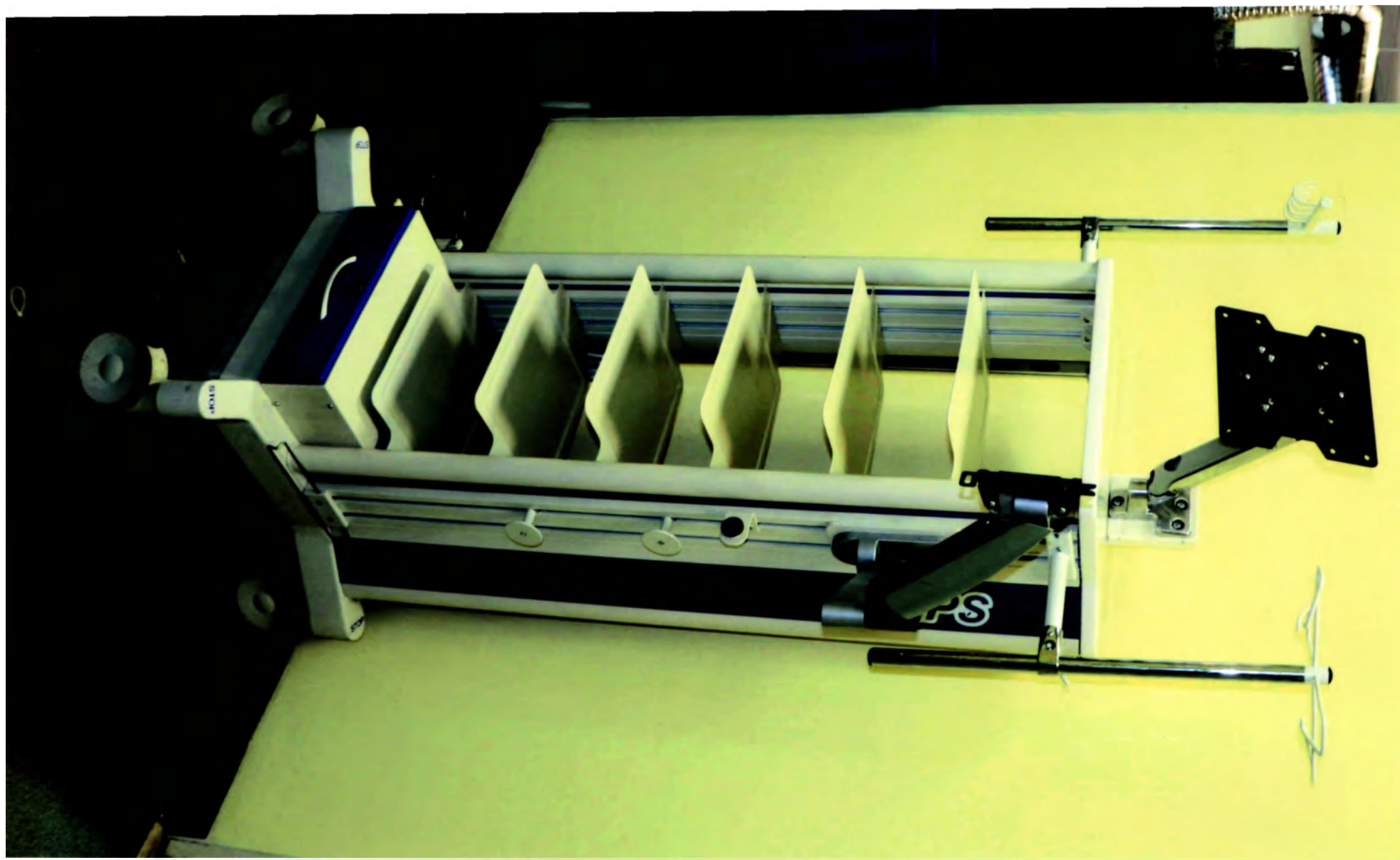
Стойка для медицинской техники CMT ELEPS с принадлежностями в исполнениях: CMT-01 ELEPS и CMT-02 ELEPS по ТУ 9452-039-12966357-2016
