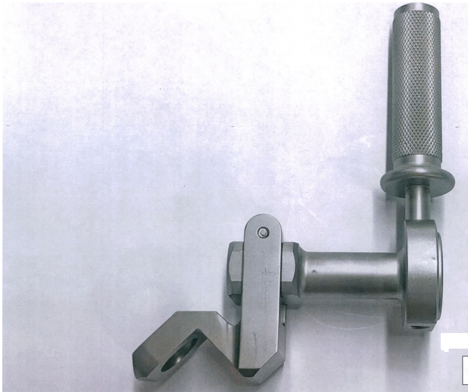
Соединитель экстрактора NEOS R
