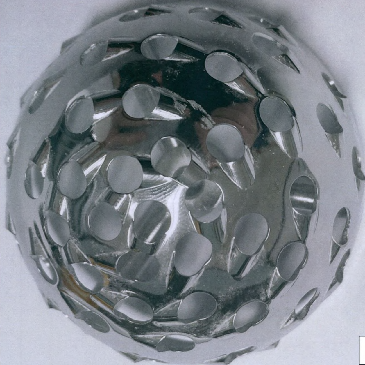
Фреза ацетабулярная, диаметр 41 мм
