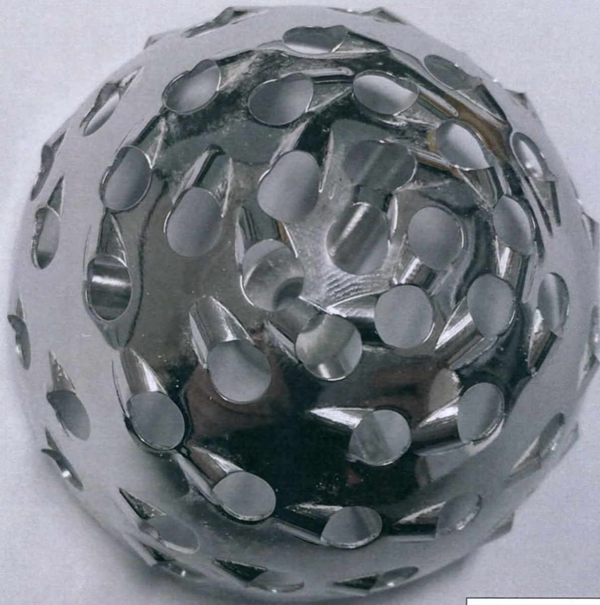
Фреза ацетабулярная, диаметр 54 мм
