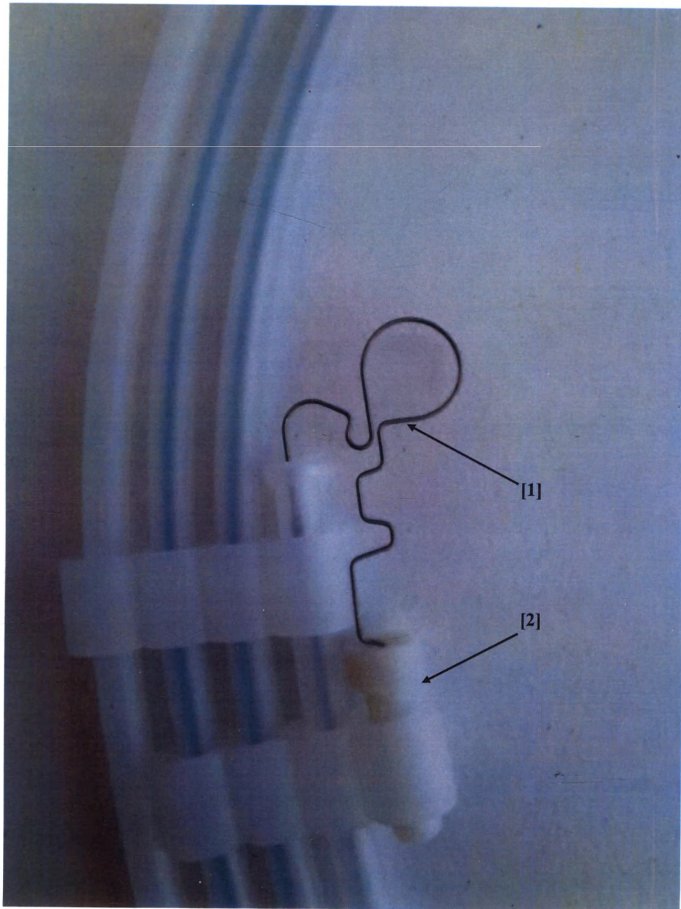
Формирующий мандрен [1] и проксимальная втулка [2] (для вариантов исполнения с кончиком типа Bern)
