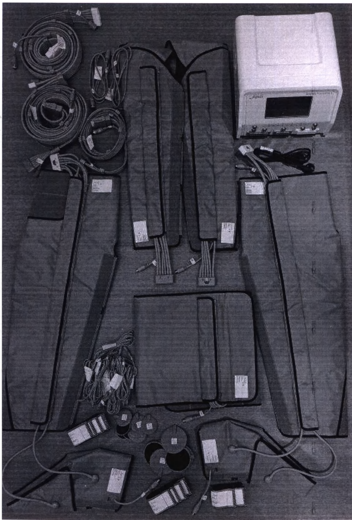
Аппарат физиотерапевтический комбинированного воздействия Scorula PressoPro 4 Рисунок 3
