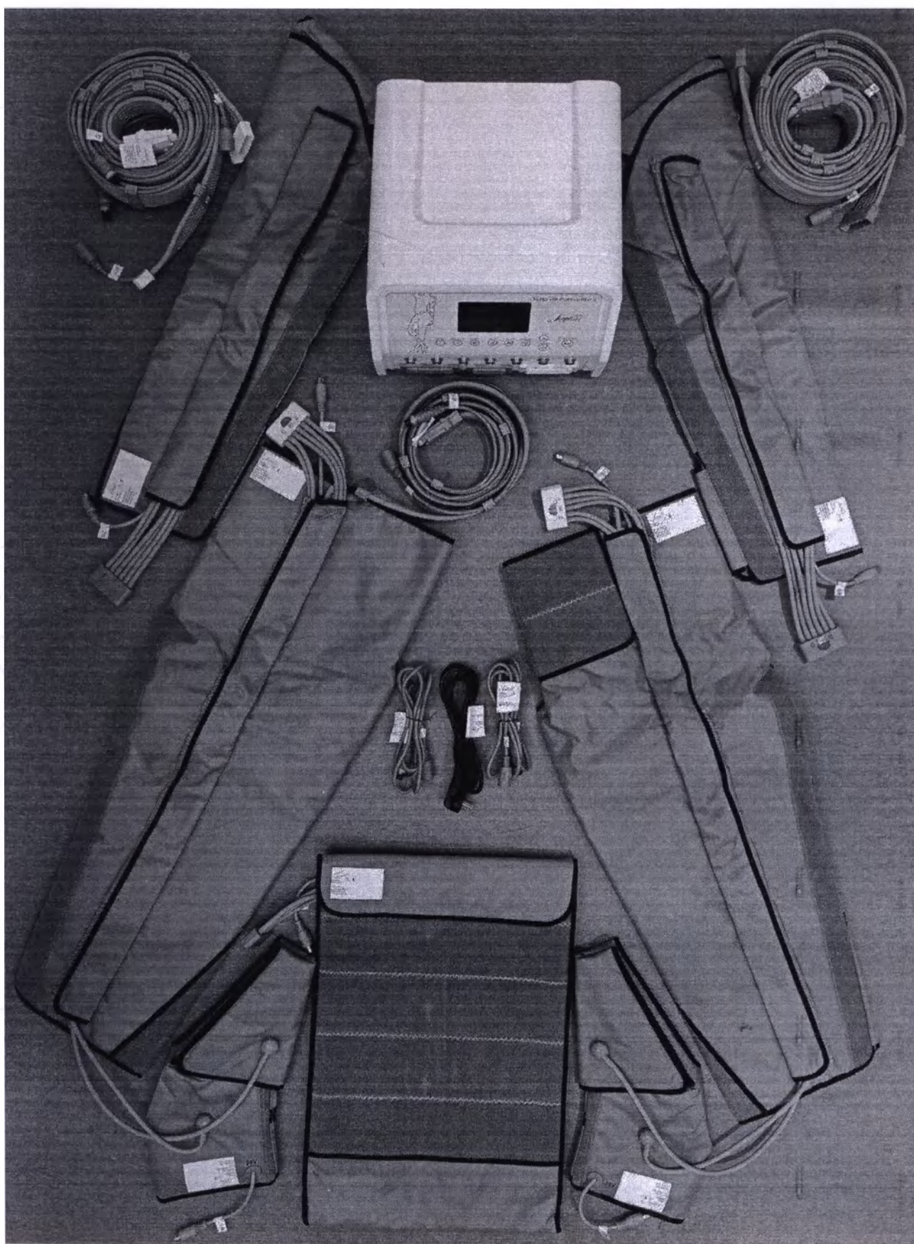
Аппарат физиотерапевтический комбинированного воздействия Scorula PressoPro 2 Рисунок 1
