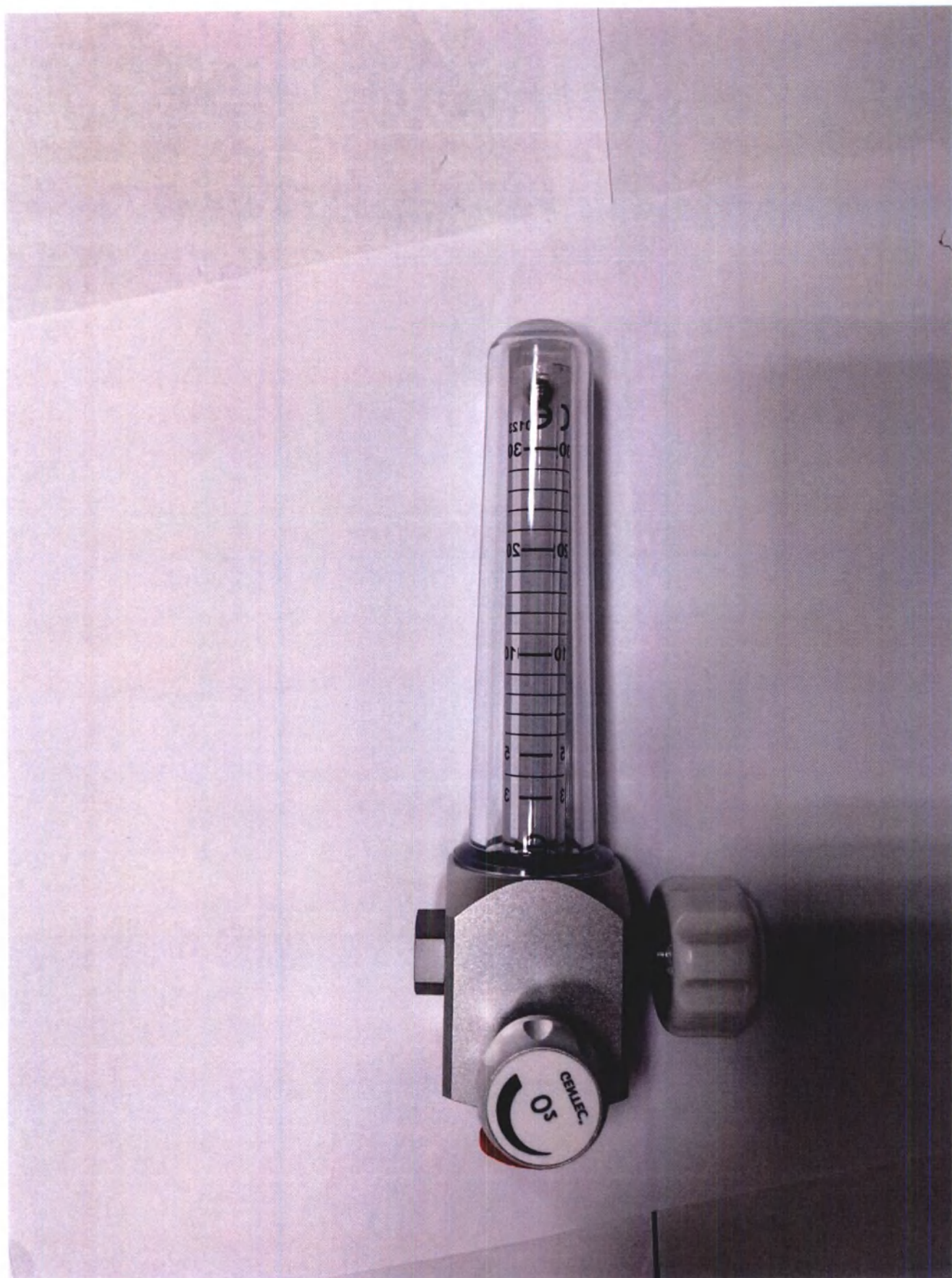
«Флоуметр медицинский, модель FM197-30L(ASD-L)»
