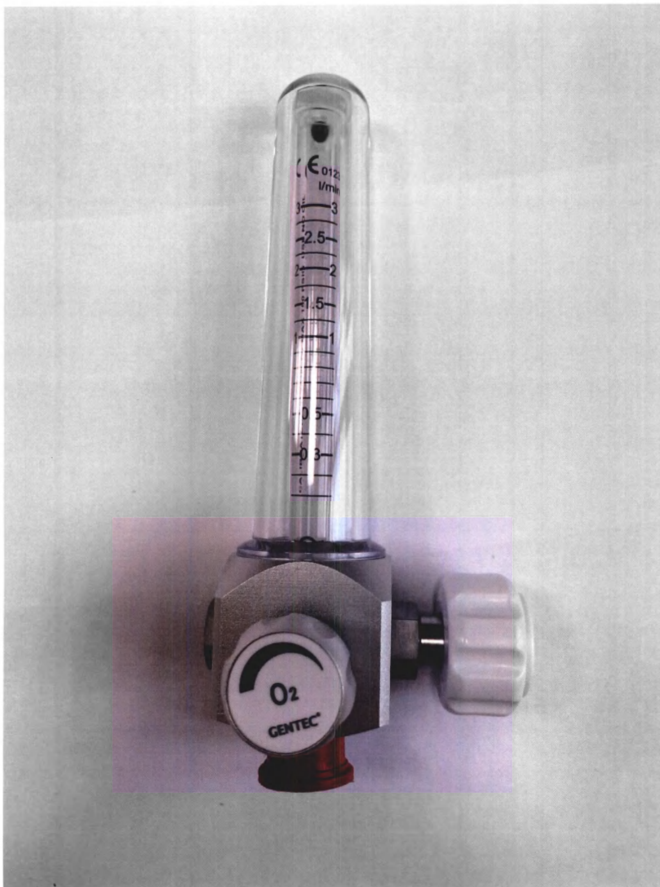
«Флоуметр медицинский, модель FM197-3L(ASD-L)»
