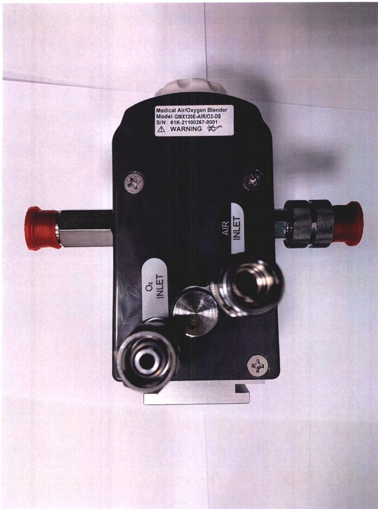
«Смеситель кислородно-воздушный медицинский Gentec®», модель GMX120E-AIR/O2» (вид снизу)
