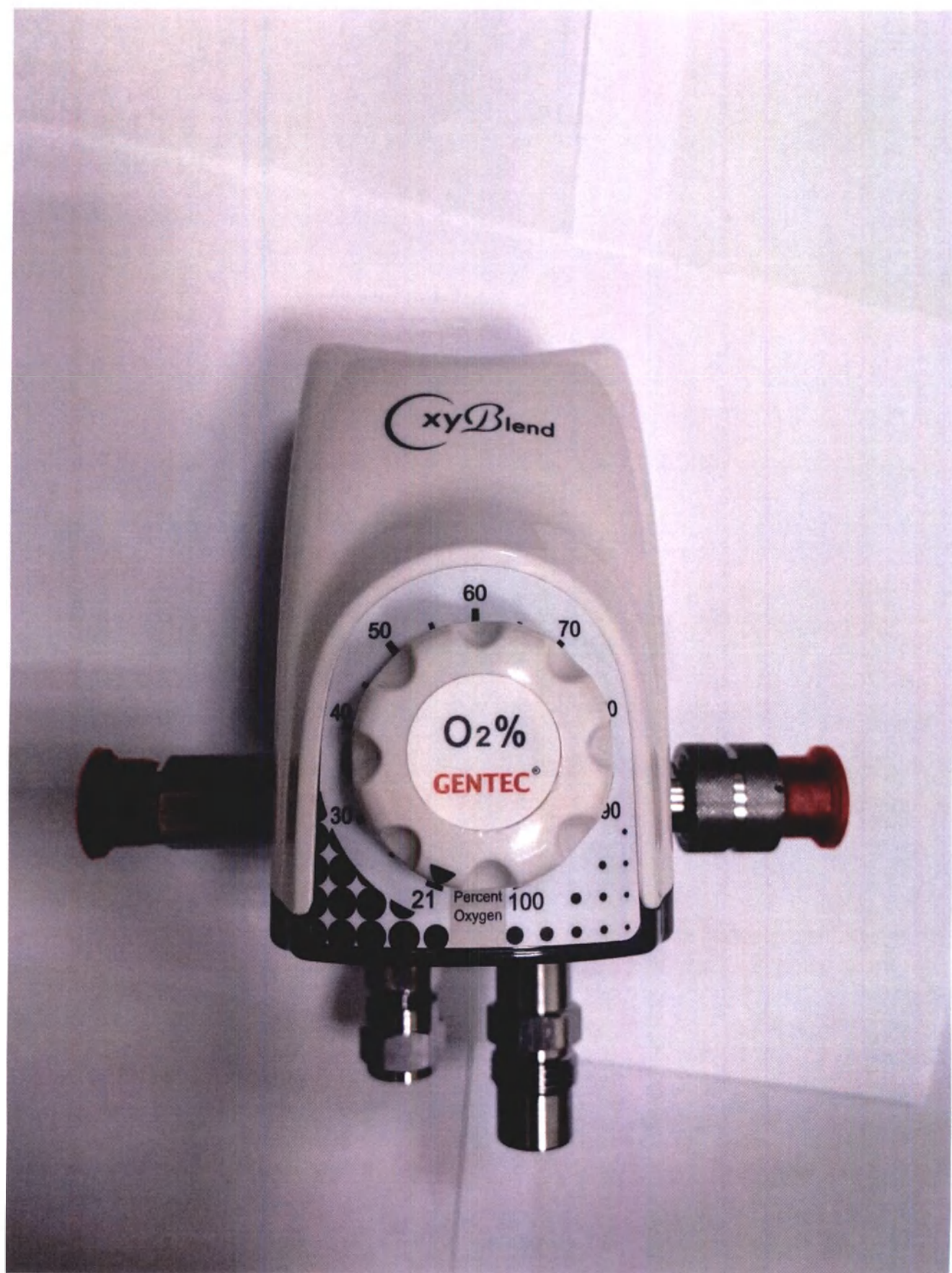
«Смеситель кислородно-воздушный медицинский Gentec®, модель GMX120E-AIR/O2» (вид спереди)
