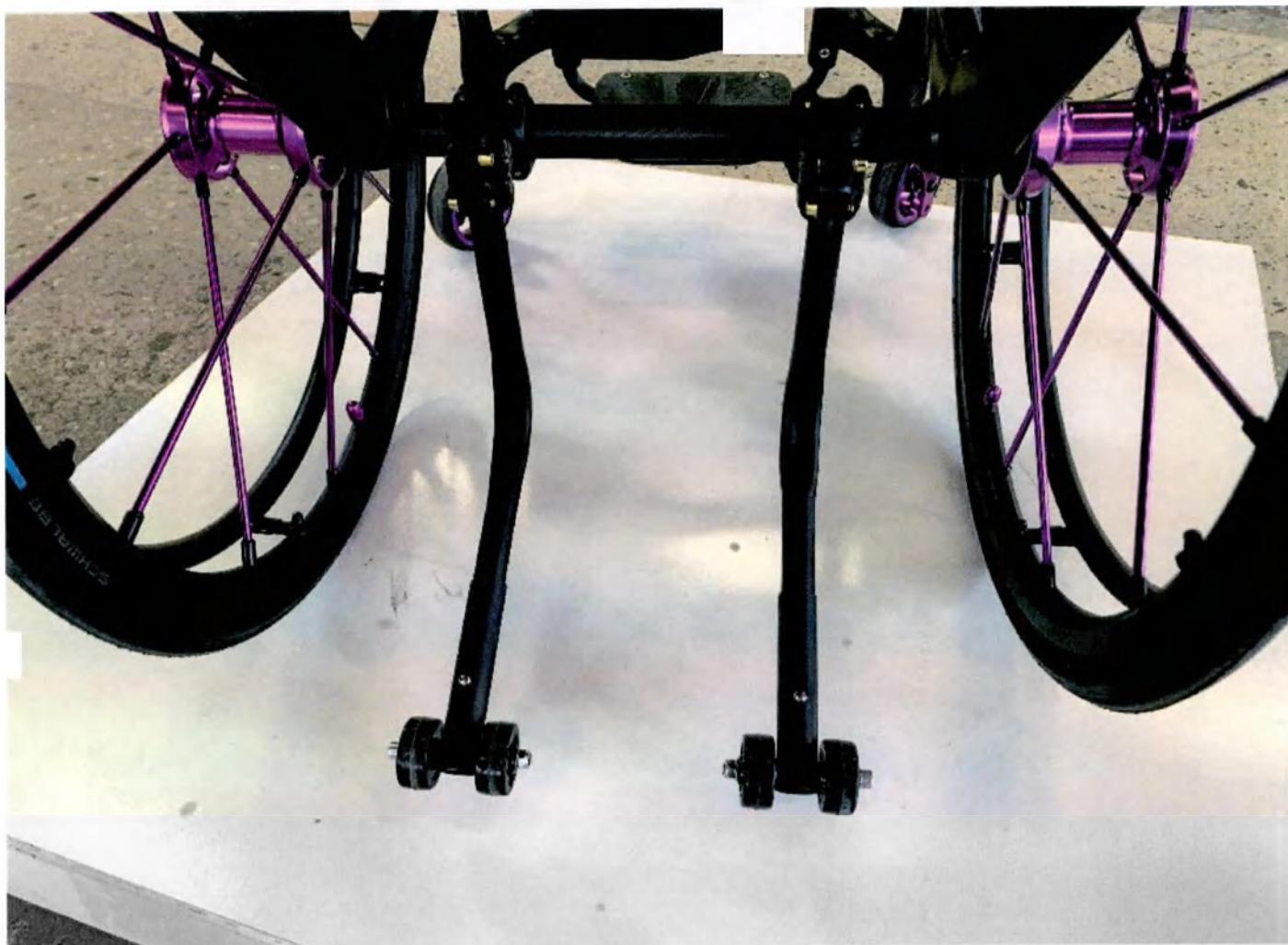
Рисунок 15. Антипрокидыватель
