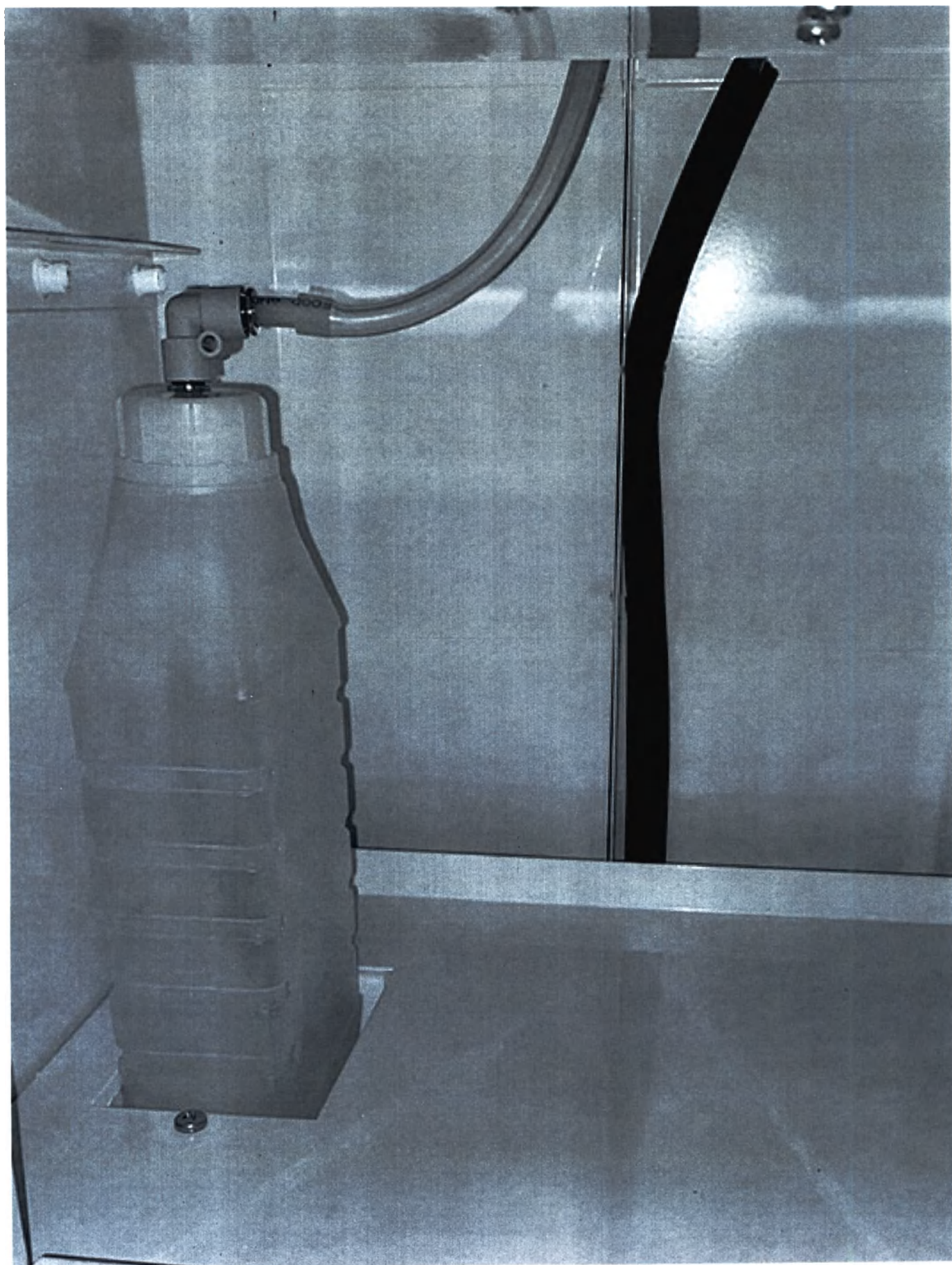
Фотографическое изображение медицинского изделия: Аппарат автоматический для аэрозольной дезинфекции по ТУ 32.50.50-072-11769436-2018 в варианте исполнения АЭРО-ДЕЗ-«КРОНТ»-01 (Соединение крышки для распыления с Емкостью ДС объемом 1\pm 0,1 л.)
