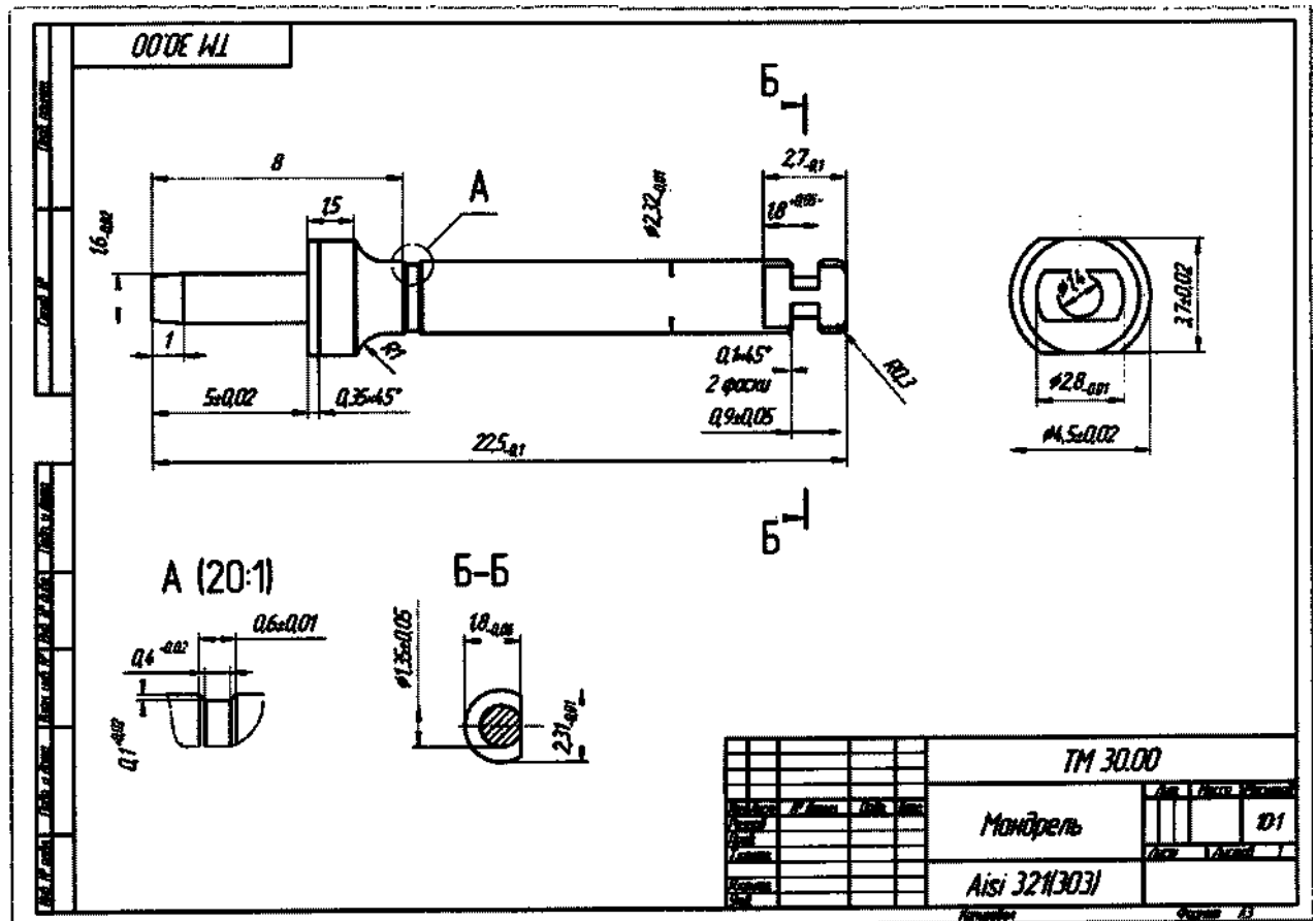
Чертёж 2. Мандрель
