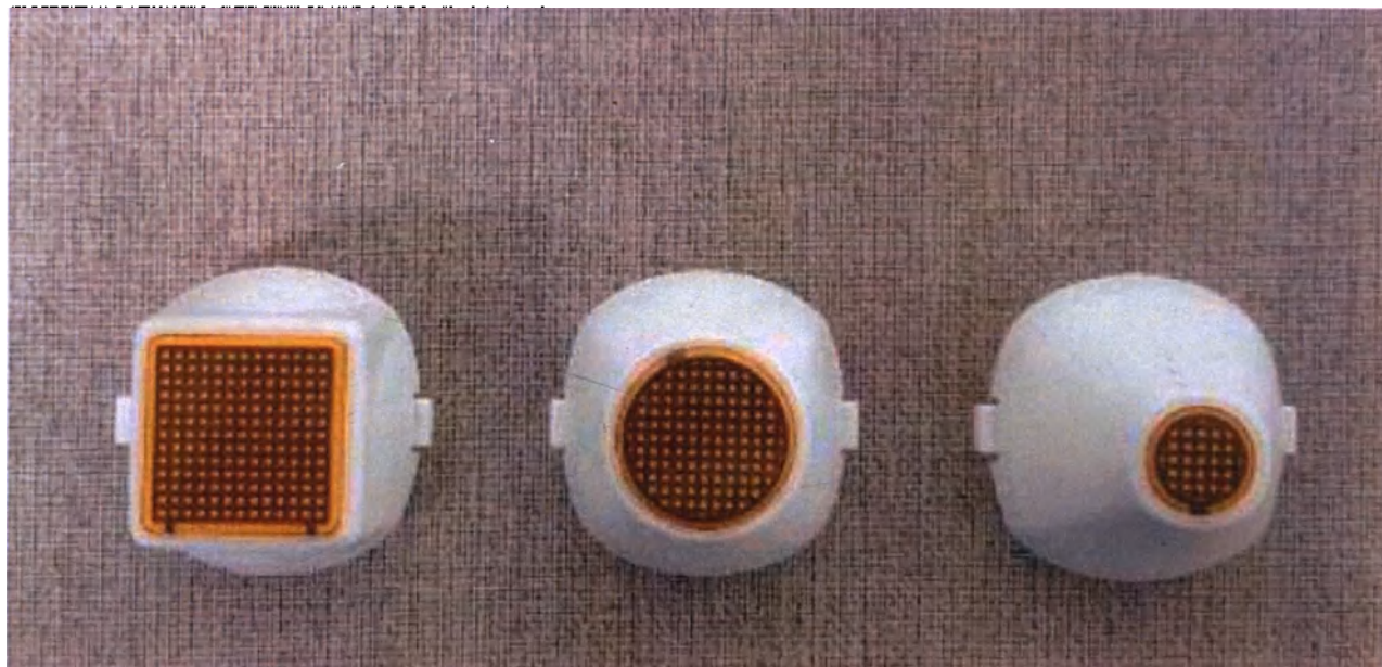
Фотографическое изображение 8 – Насадка для теплового RF, тип TRF Tip-S, тип TRF Tip-R, тип TRF Tip-E
