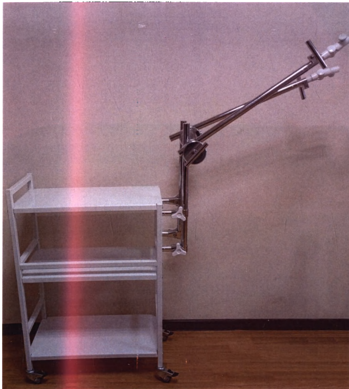
Тележка (индуктородержатель) в сборе
