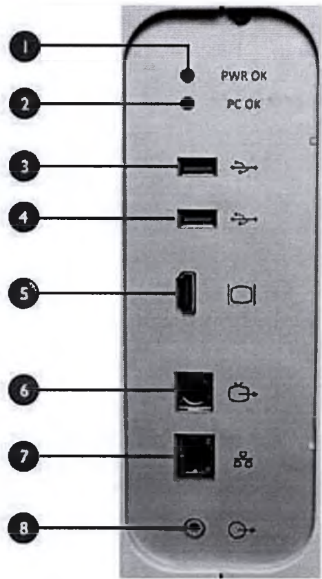
Задняя панель
