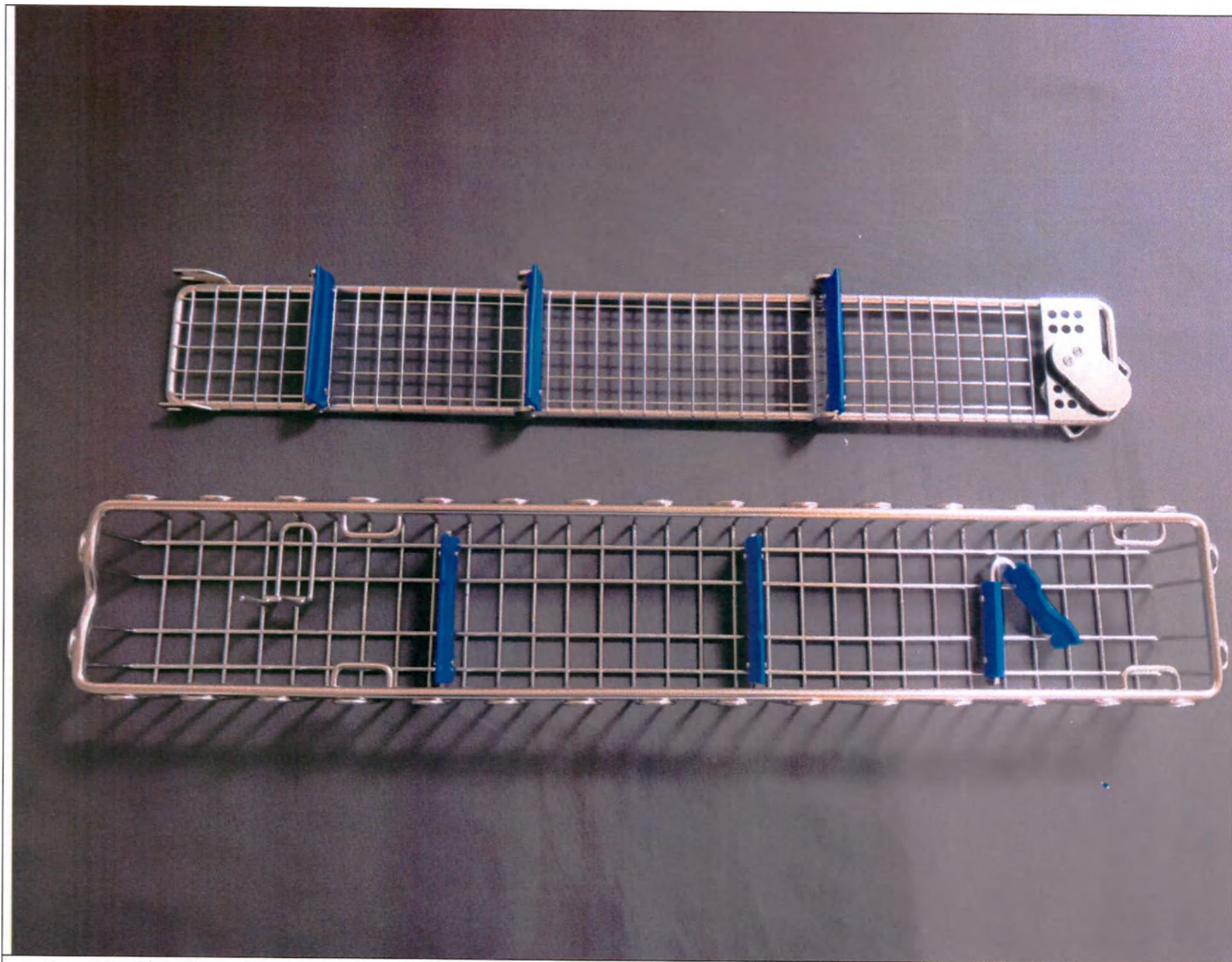
Рис. 115. Контейнер проволочный для дезинфекции/стерилизации/хранения, размеры: 460 x 80 x 52 мм
