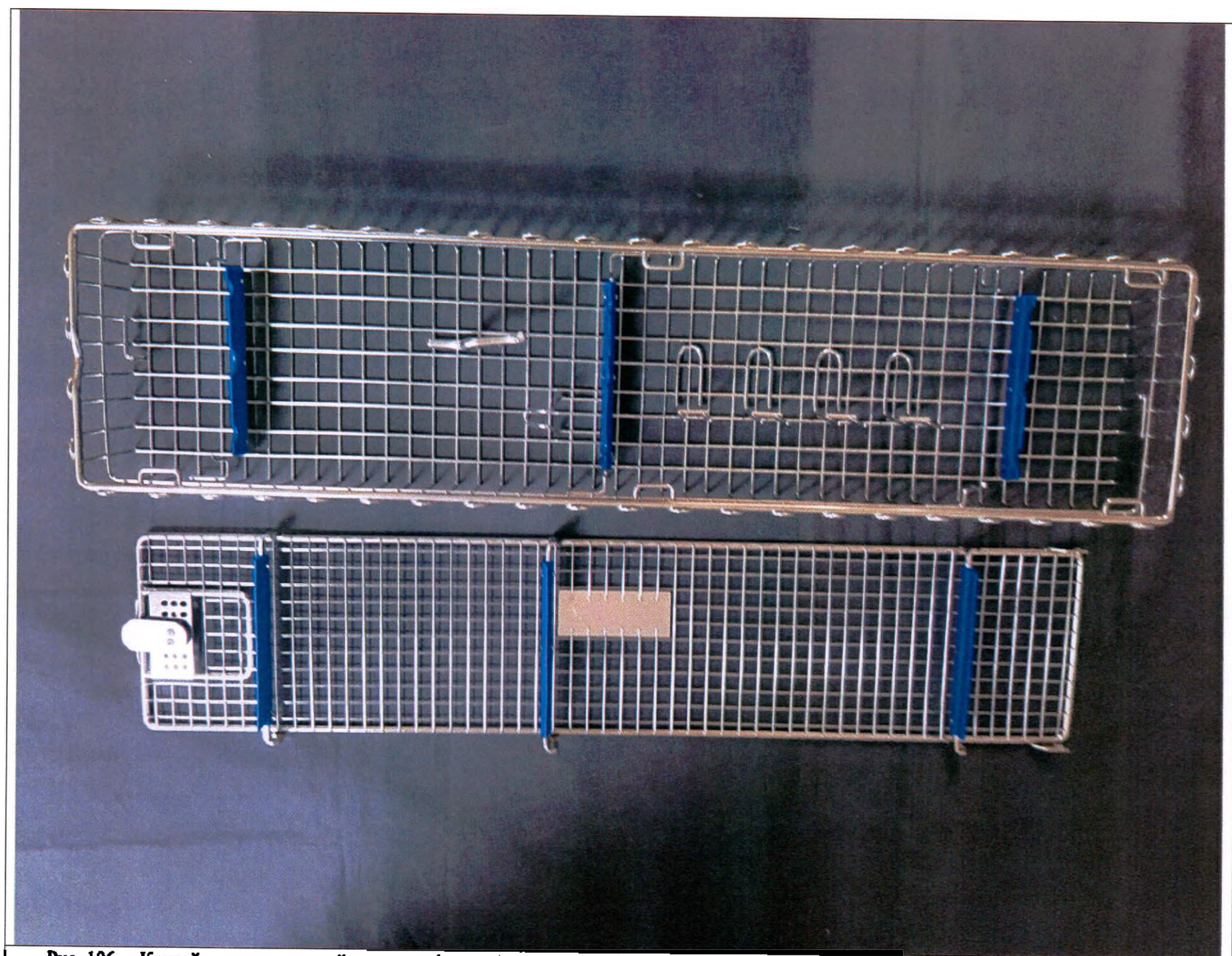
Рис. 106. Контейнер проволочный для дезинфекции/стерилизации/хранения, размеры: 622 x 150 x 78 мм.
