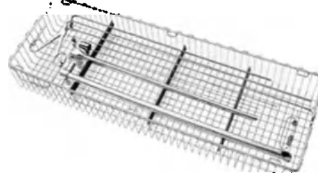
Контейнер проволочный для дезинфекции/стерилизации/хранения, размеры: 640 x 216 x 78 мм Wire container for disinfection / sterilization / storage, dimensions: 640 x 216 x 78 mm
