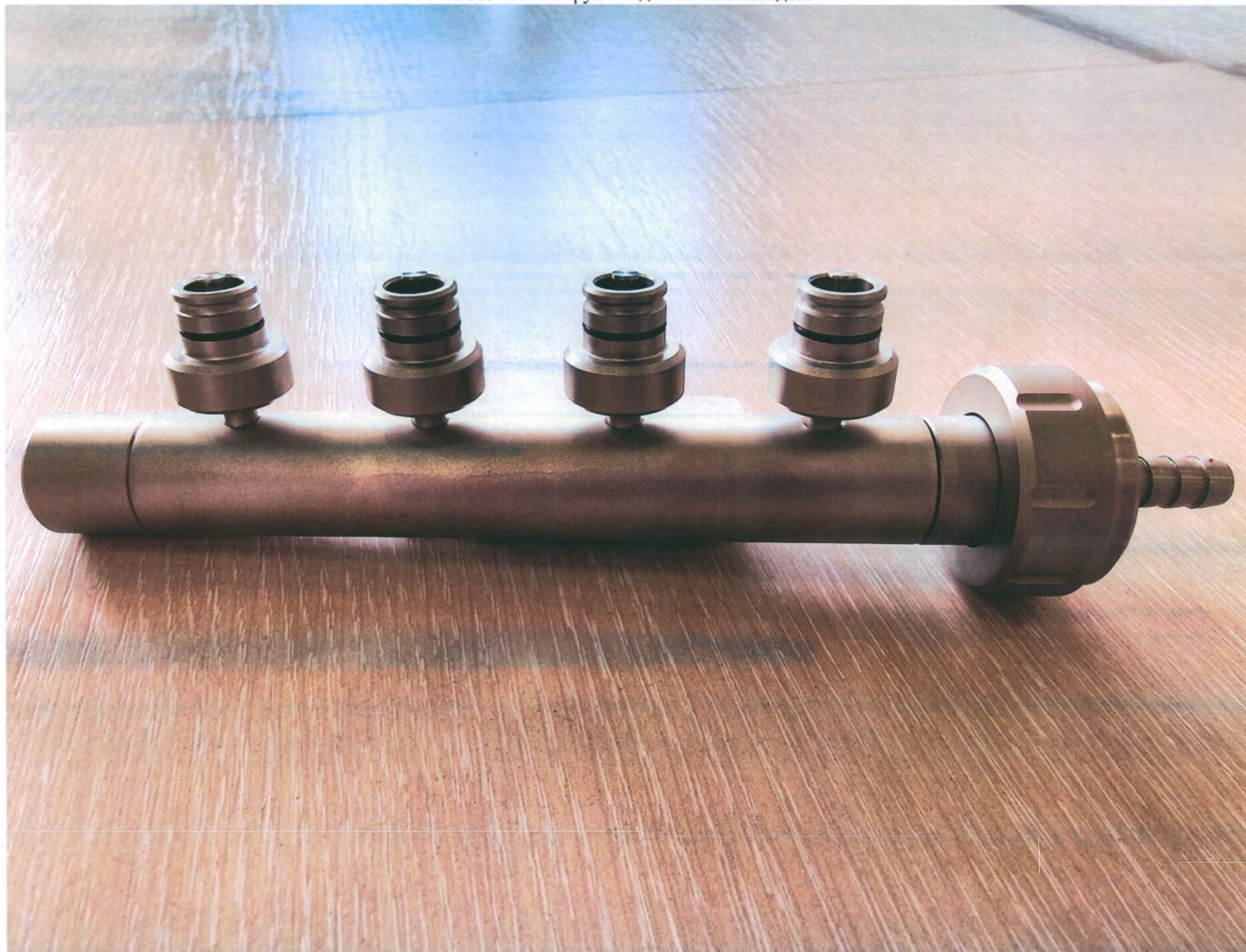
Фото 47. Инструмент для чистки насадок.
