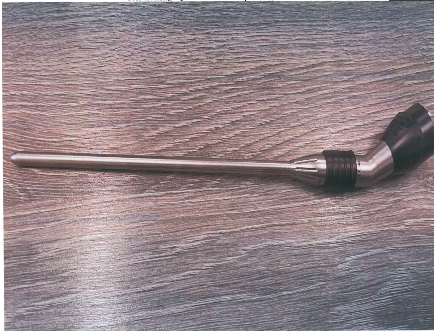
Фото 19. Насадка угловая XXL ALPHA, общая длина 250 мм.
