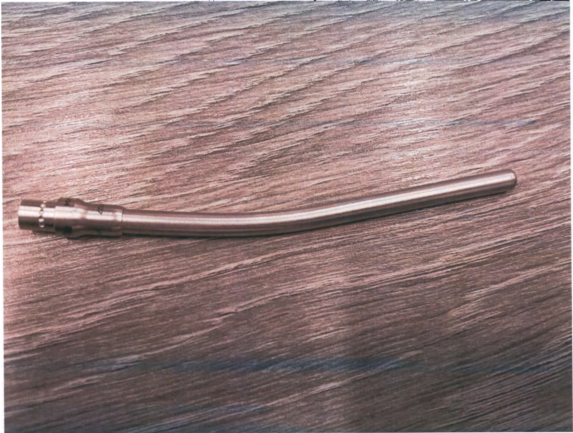
Фото 37. Насадка телескопическая изогнутая, общая длина 120 мм.
