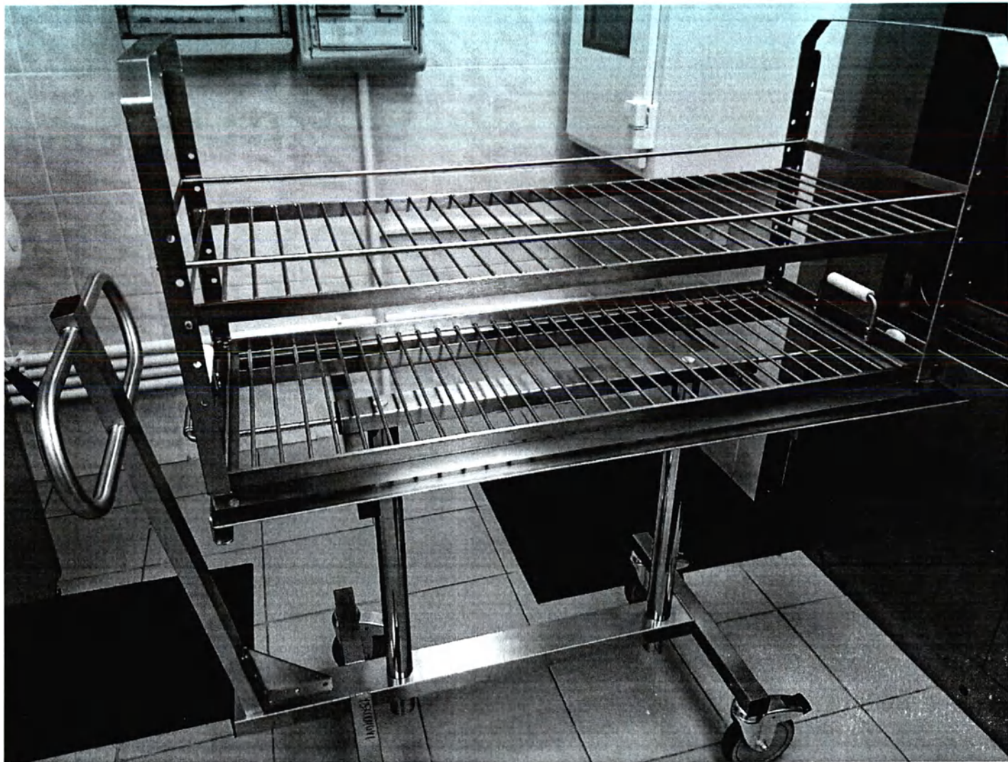
42. Тележка передвижная для 1 стеллажа 720х600х1110 со стеллажом на колесиках с фиксированными полками 625х615х1100
