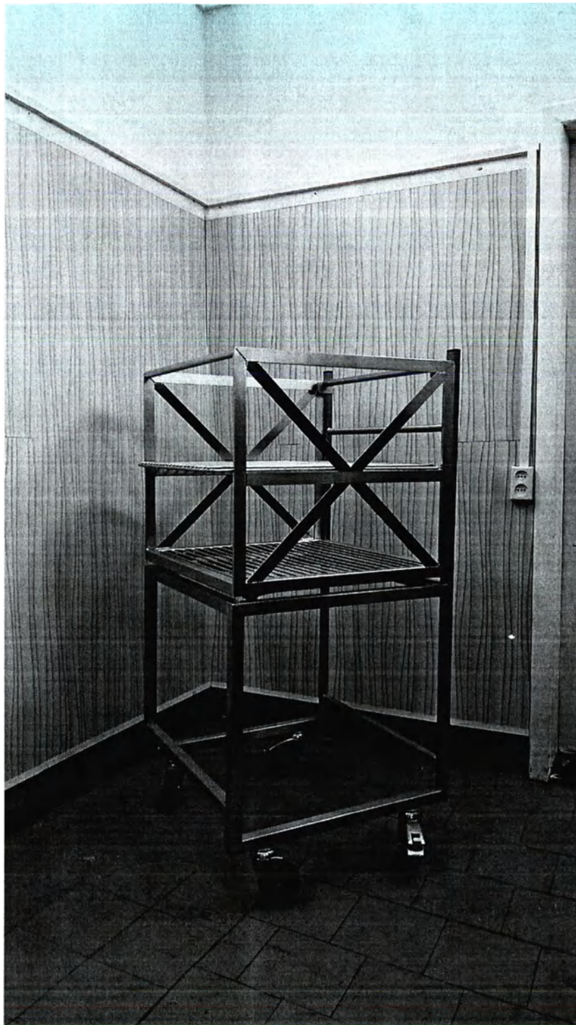
19. Тележка передвижная для 1 стеллажа 625x600x1250 со стеллажом на колесиках с выдвижными полками 460x430x550
