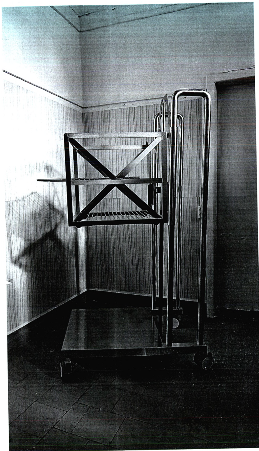
55. Тележка передвижная для 2 стеллажей 810x820x1589 со стеллажом на колесиках с выдвижными полками 460x430x550
