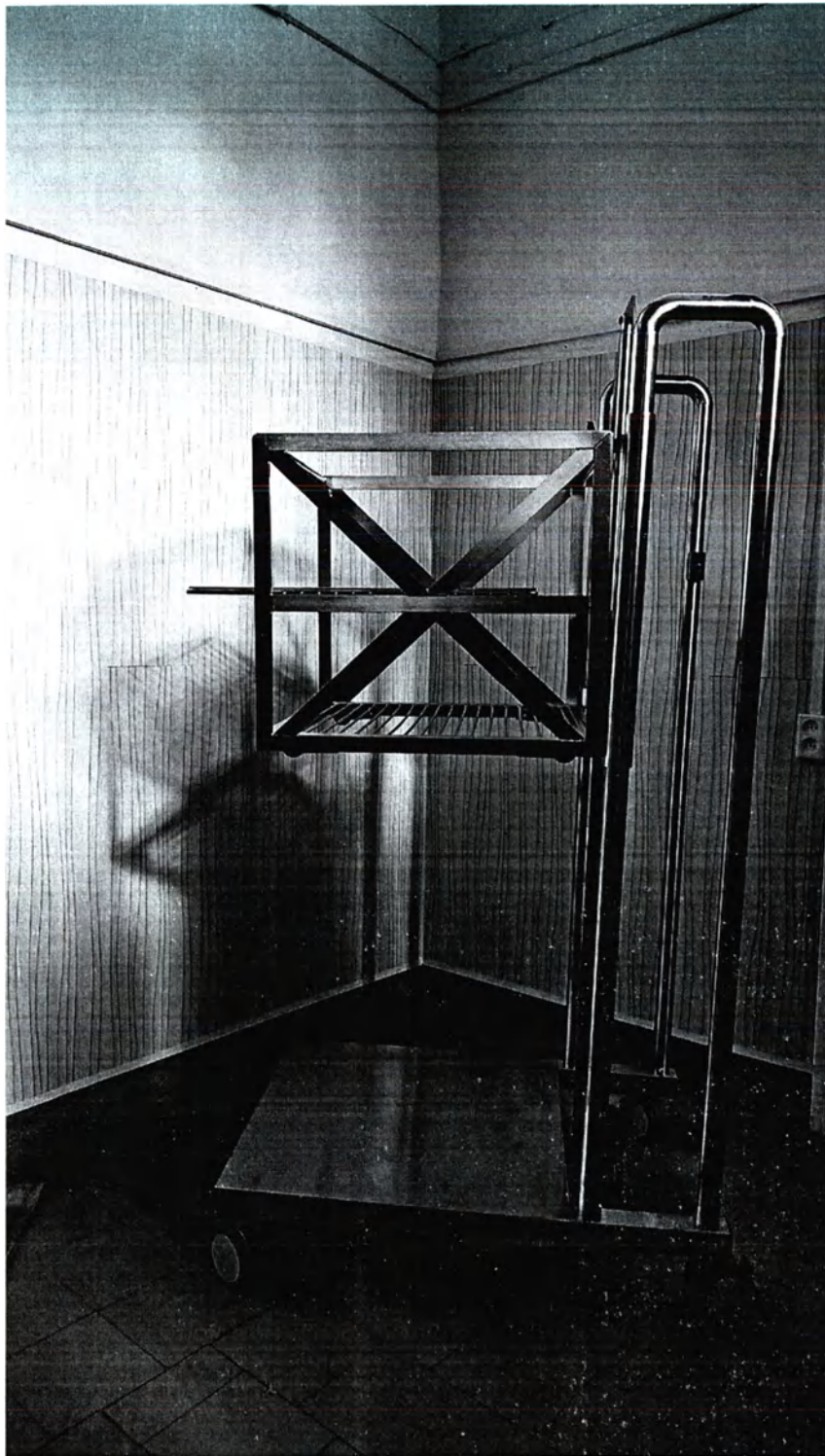
61. Тележка передвижная для 2 стеллажей 810x820x2000 со стеллажом без колесиков с выдвижными полками 460x430x550
