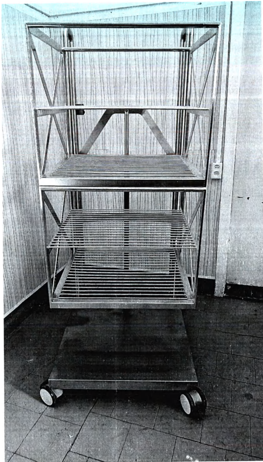
58. Тележка передвижная для 2 стеллажей 810x820x1589 со стеллажом без колесиков с фиксированными полками 625x615x1100
