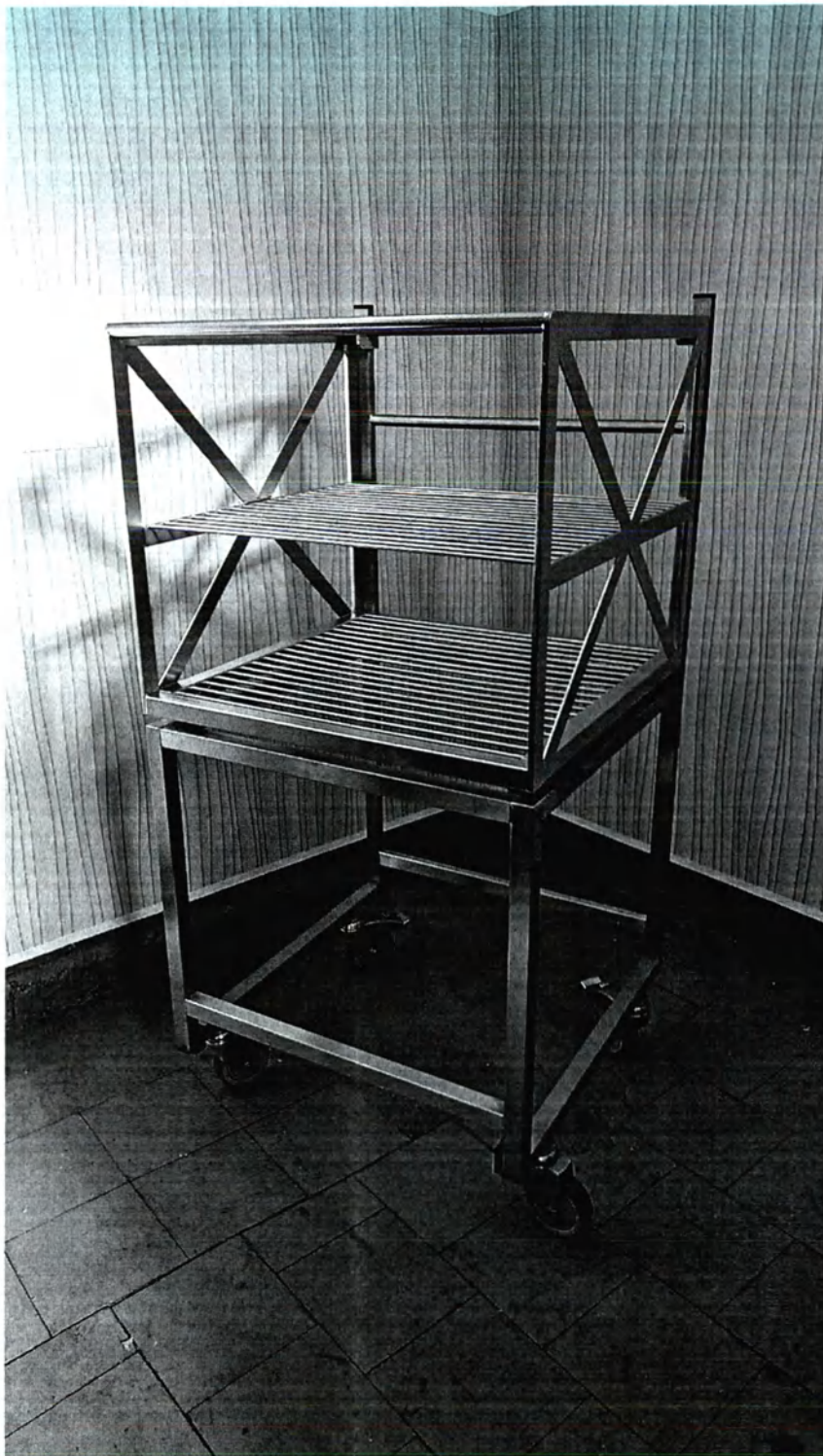
23. Тележка передвижная для 1 стеллажа 625х600х1250 со стеллажом на колесиках с фиксированными полками 460х430х550
