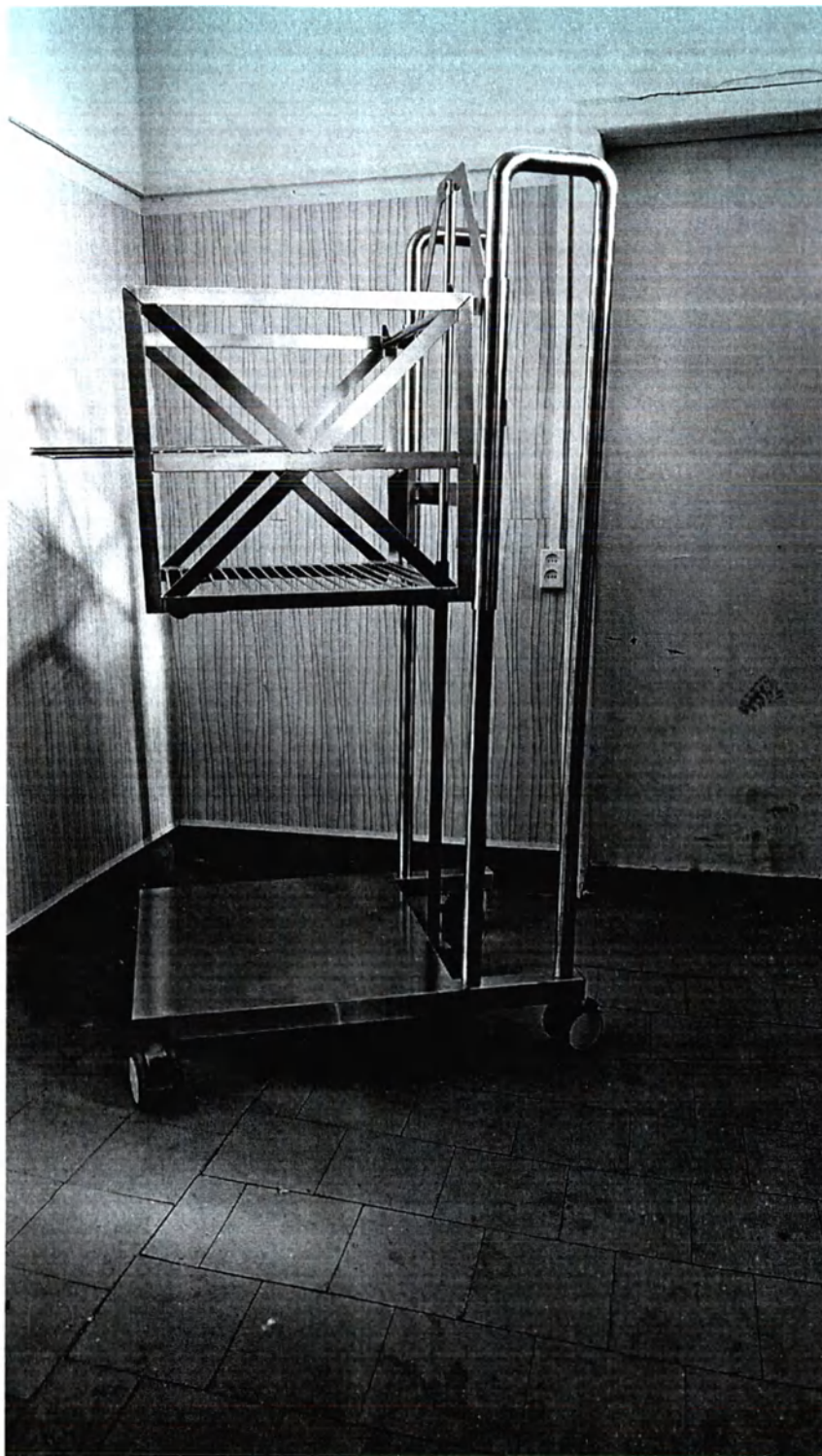
45. Тележка передвижная для 2 стеллажей 810x750x1589 со стеллажом без колесиков с выдвижными полками 460x430x550
