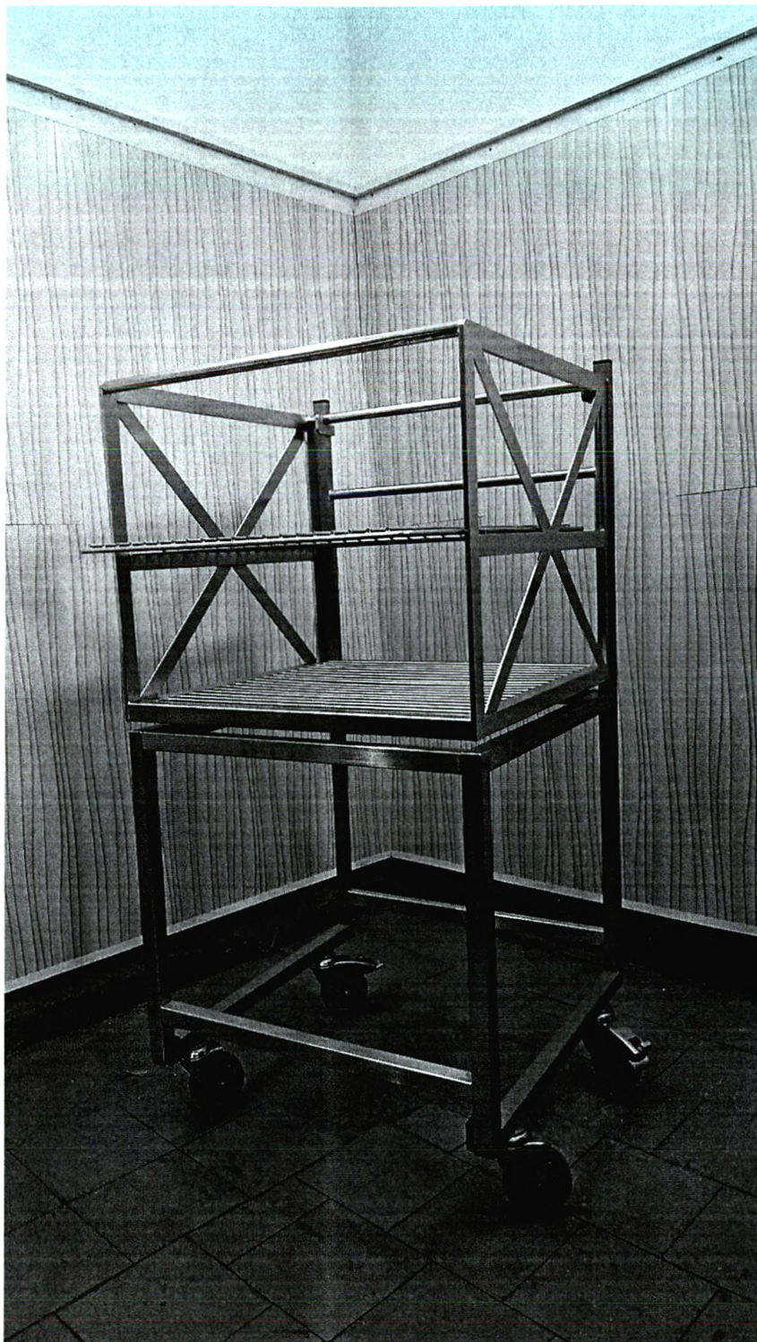
17. Тележка передвижная для 1 стеллажа 625х600х1250 со стеллажом без колесиков с выдвижными полками 460х430х550
