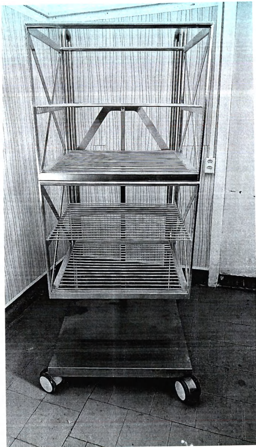
60. Тележка передвижная для 2 стеллажей 810x820x1589 со стеллажом на колесиках с фиксированными полками
