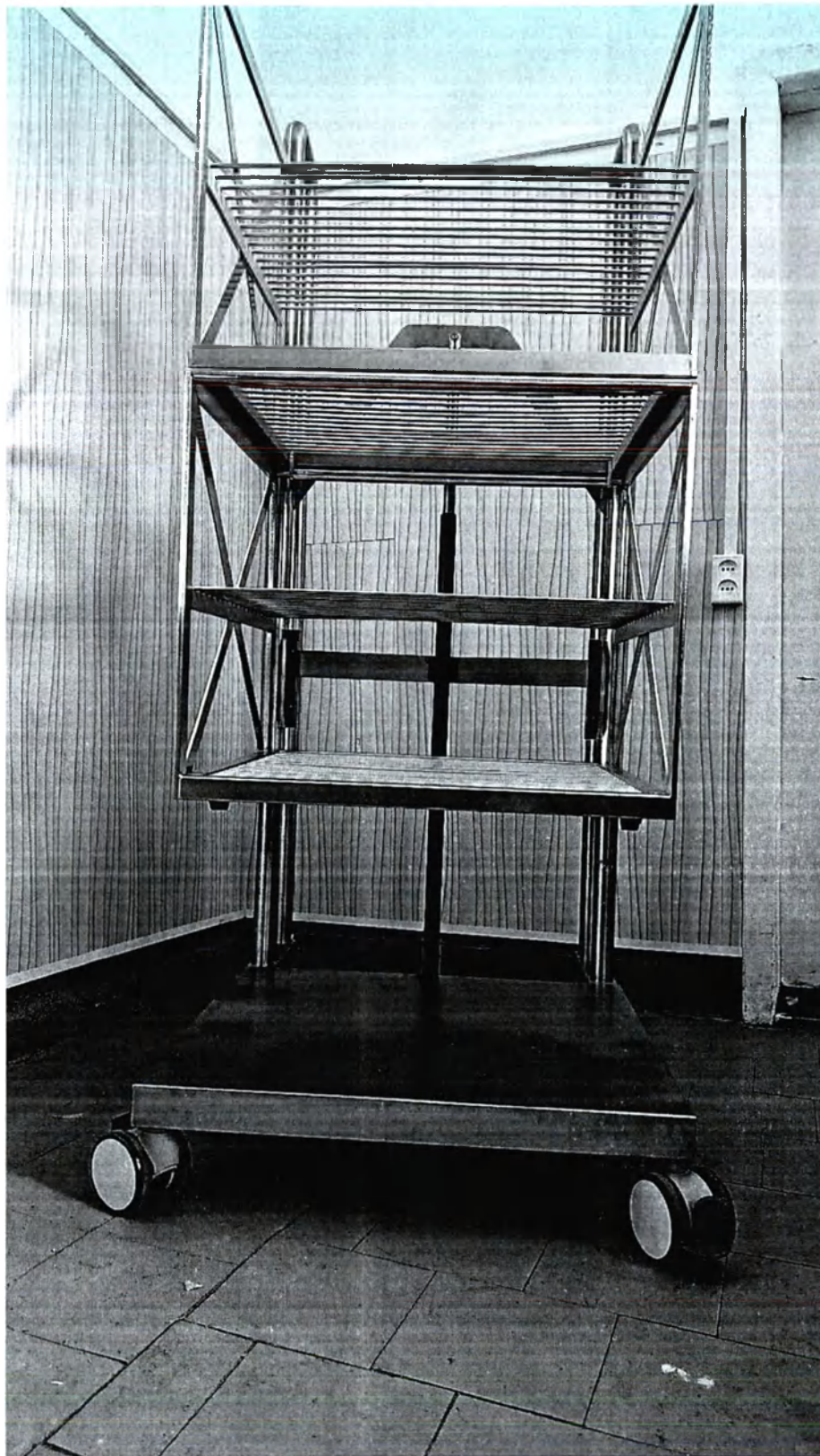
66. Тележка передвижная для 2 стеллажей 810x820x2000 со стеллажом без колесиков с фиксированными полками 625x615x1100
