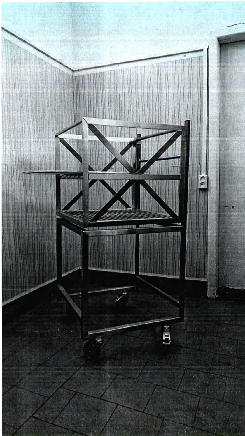
33. Тележка передвижная для 1 стеллажа 650х600х1340 со стеллажом без колесиков с выдвижными полками 460х430х550
