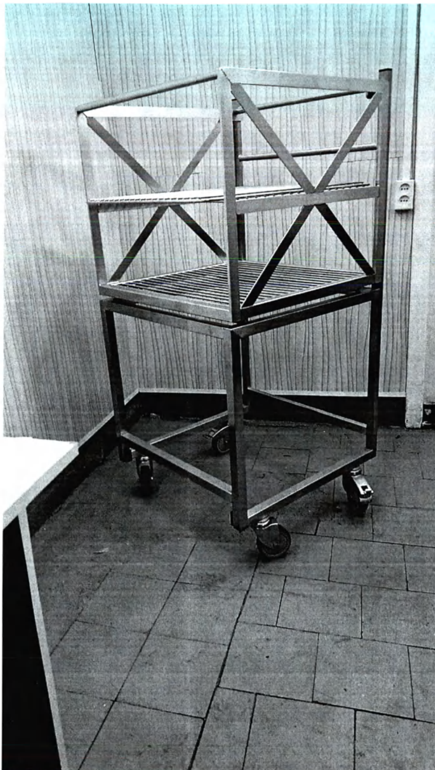
11. Тележка передвижная для 1 стеллажа 648х618х1325 со стеллажом на колесиках с выдвижными полками 460х430х550
