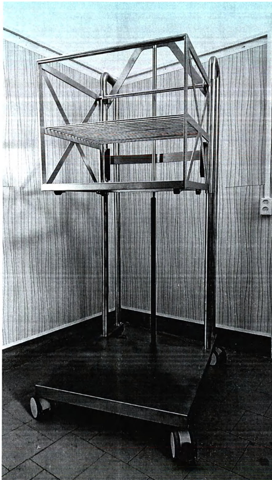
67. Тележка передвижная для 2 стеллажей 810x820x2000 со стеллажом на колесиках с фиксированными полками 460x430x550
