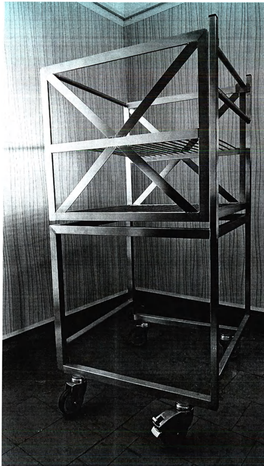
5. Тележка передвижная для 1 стеллажа 673x583x1328 со стеллажом без колесиков с фиксированными полками 460x430x550
