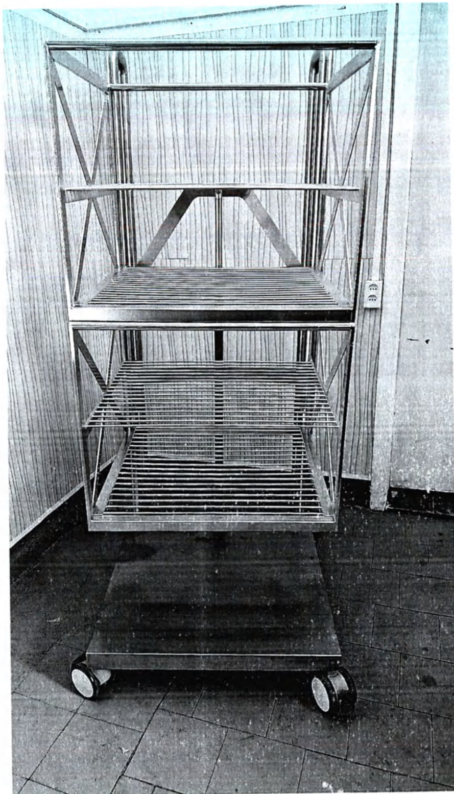
68. Тележка передвижная для 2 стеллажей 810x820x2000 со стеллажом на колесиках с фиксированными полками
