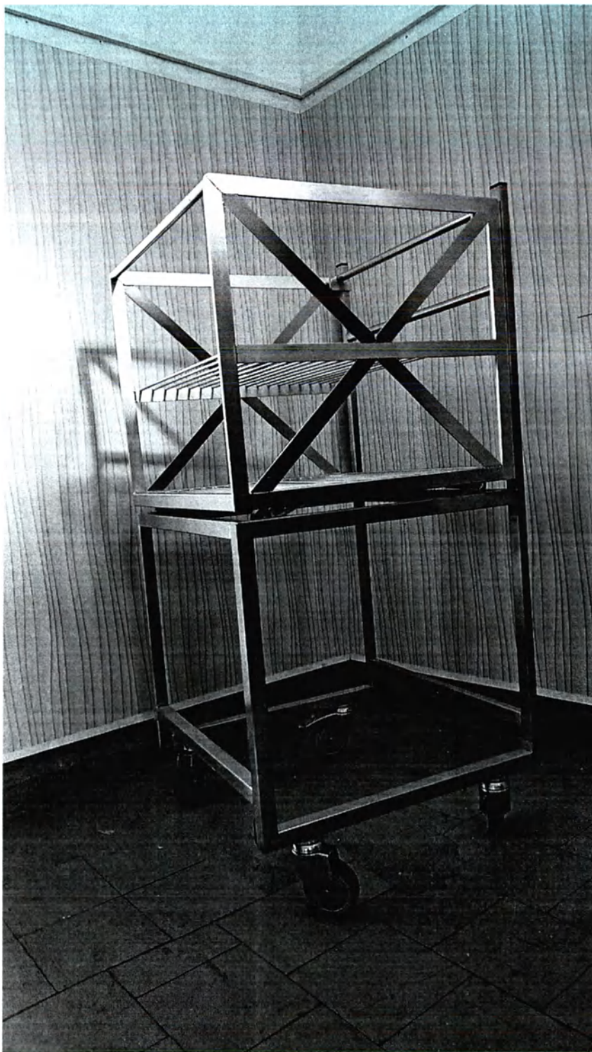
39. Тележка передвижная для 1 стеллажа 650x600x1340 со стеллажом на колесиках с фиксированными полками 460x430x550
