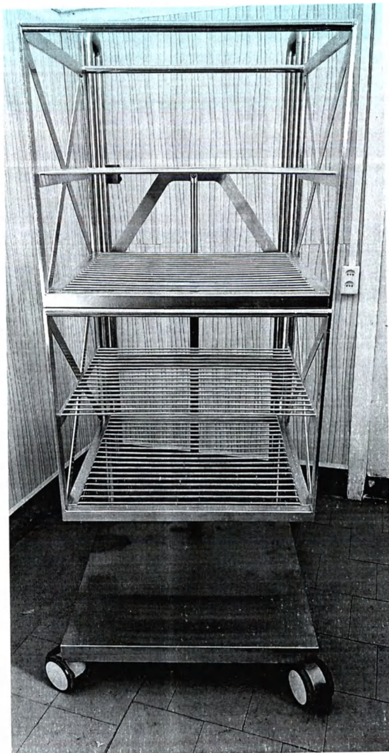
50. Тележка передвижная для 2 стеллажей 810x750x1589 со стеллажом без колесиков с фиксированными полками 625x615x1100
