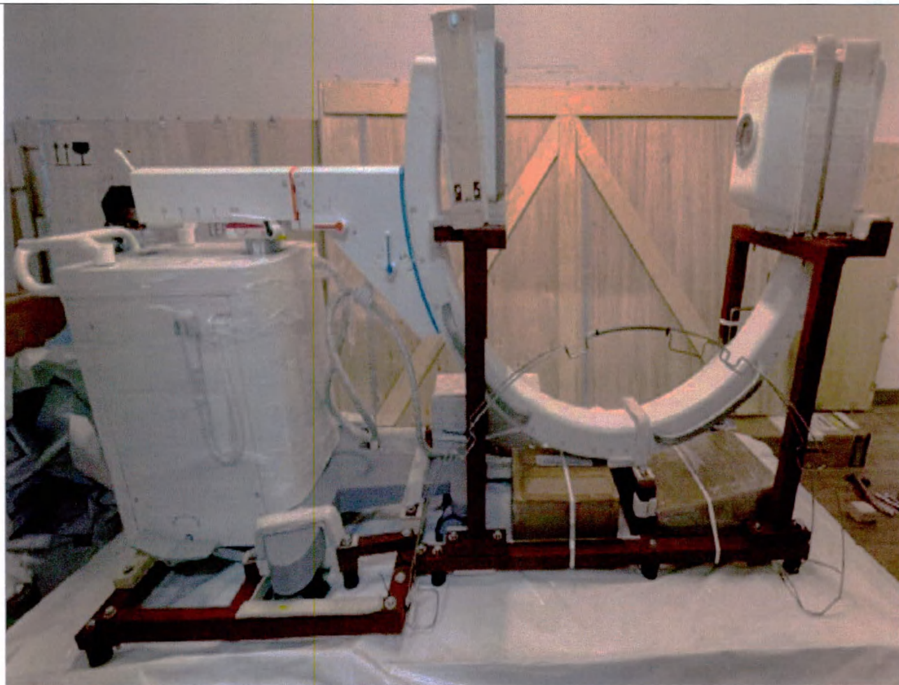
1. Пример расположения стойки С-дуги на поддоне
