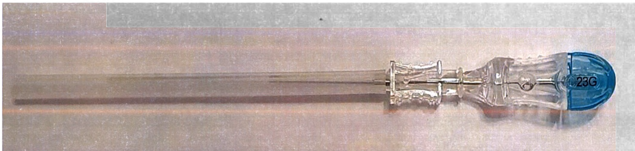
Игла инъекционная ACUS для анестезии, спинальная, срез Уайтэкра, тип Пенсил поинт, с интродьюсером и стилетом, размер 0.60мм×92мм/23G (аналогичный внешний вид размеров 0.60мм×110мм/23G)
