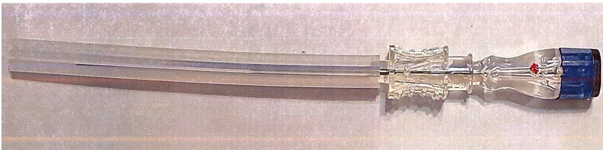
Игла инъекционная ACUS для анестезии, Срез Квинке, с интродьюсером и стилетом, размер 0.60мм×92мм/23G (аналогичный внешний вид размера 0.60мм×110мм/23G)
