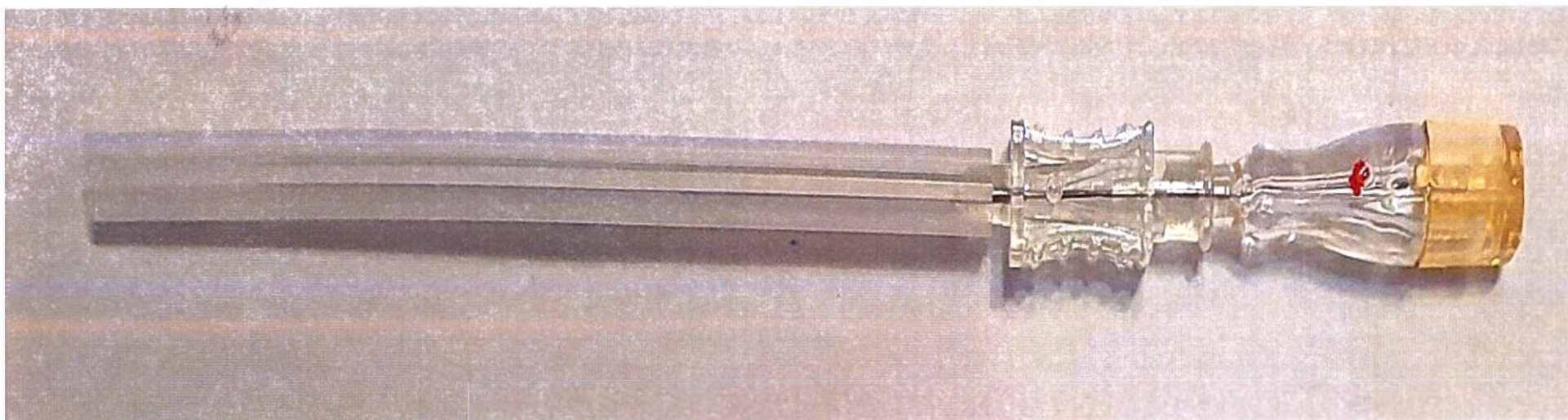
Игла инъекционная ACUS для анестезии, Срез Квинке, с интродьюсером и стилетом, размер 0.90мм×92мм/20G (аналогичный внешний вид размеров 0.90мм×110мм/20G, 0.90мм×120мм/20G)
