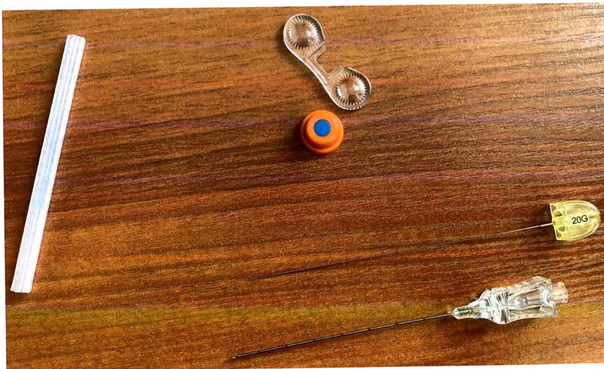
Игла инъекционная AKUS для анестезии, эпидуральная с крыльями, тип Туохи со стилетом, размер: 0,90 × 80 мм / 20G в разборном виде
