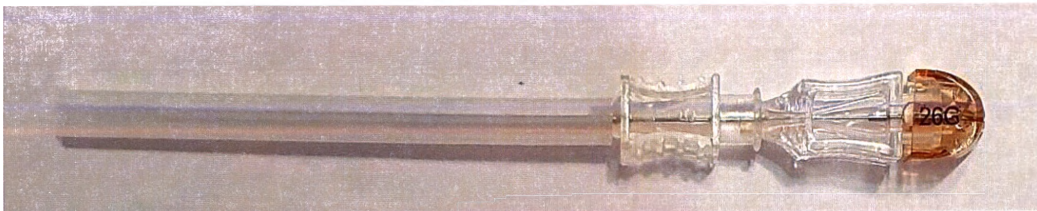
Игла инъекционная ACUS для анестезии, спинальная, срез Уайтэкра, тип Пенсил поинт, с интродьюсером и стилетом, размер 0.45мм×92мм/26G (аналогичный внешний вид размеров 0.45мм×110мм/26G)
