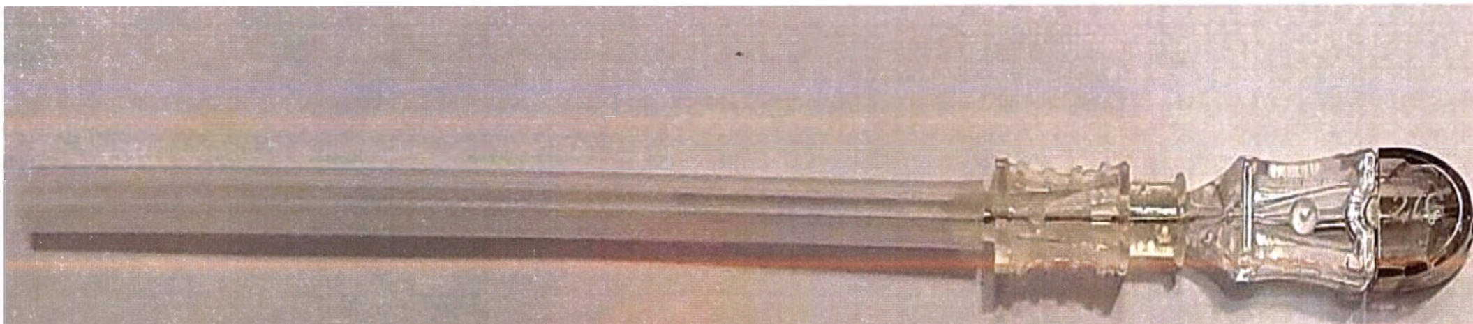
Игла инъекционная ACUS для анестезии, спинальная, срез Уайтэкра, тип Пенсил поинт, с интродьюсером и стилетом, размер 0.40мм×50мм/27G (аналогичный внешний вид размеров 0.40мм×92мм/27G, 0.40мм×110мм/27G, 0.40мм×126мм/27G)
