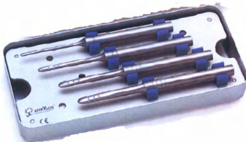
Рисунок 5 Набор с экспандерами кости, в комплекте
