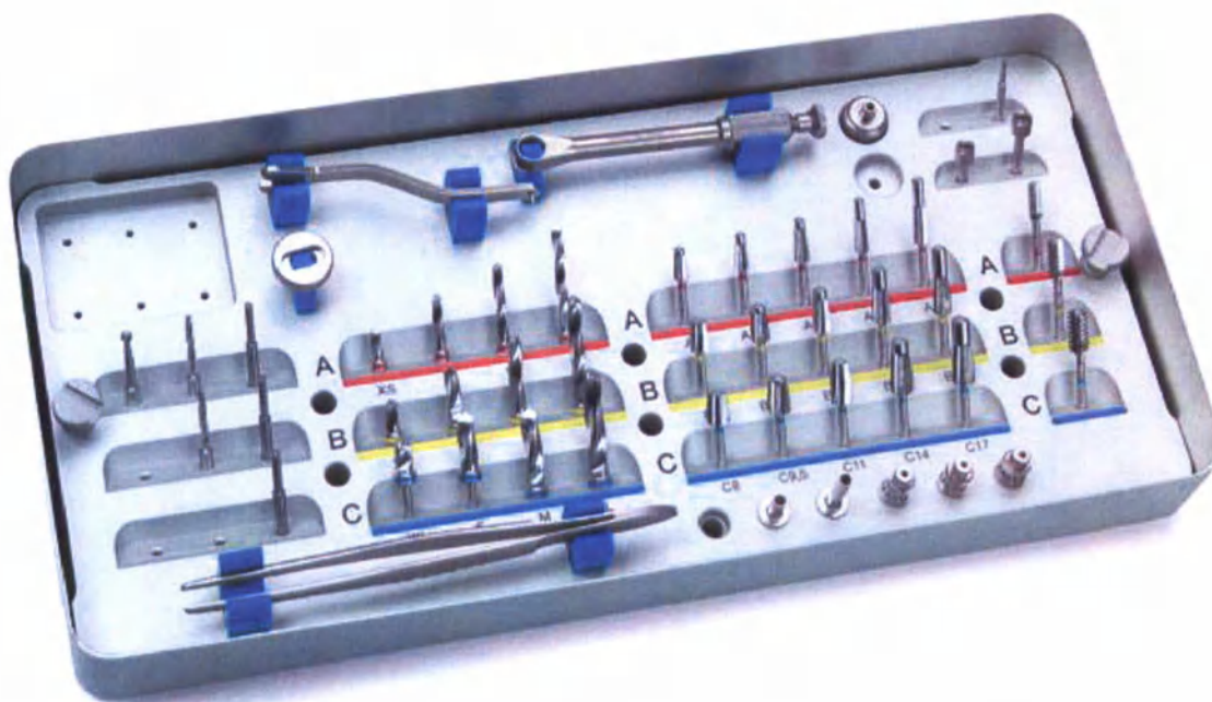
Рисунок 1 Хирургический набор для имплантатов A+B+C для ручного препарирования в комплекте
