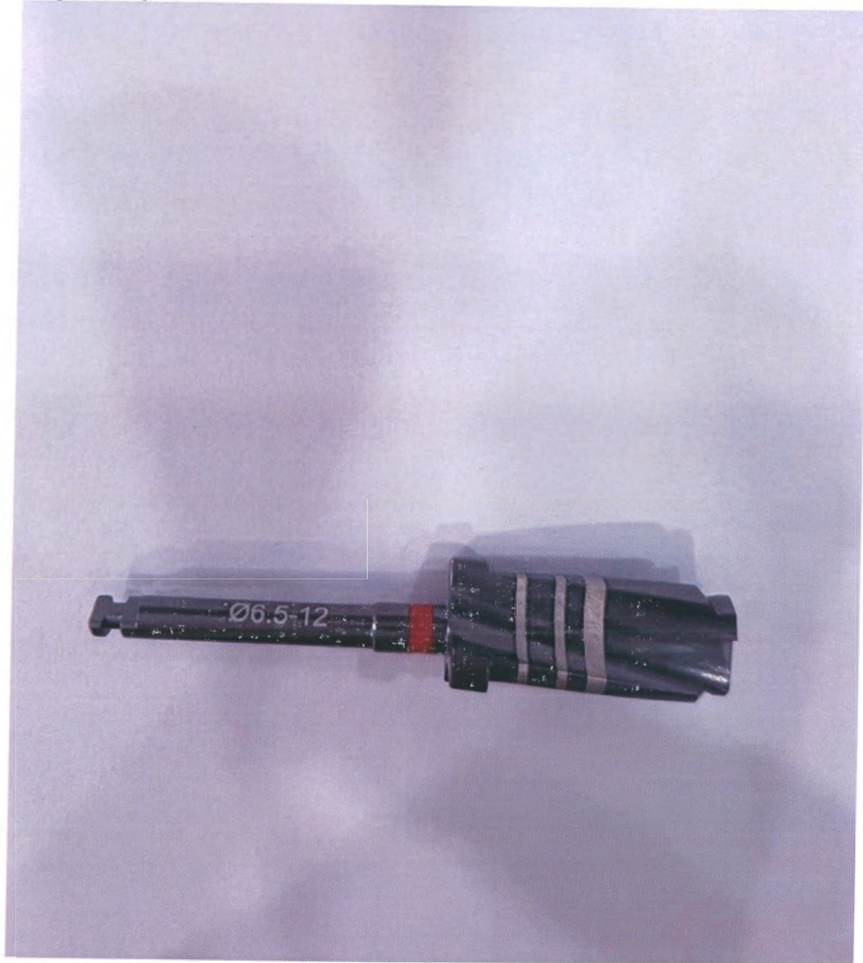
Сверло OneQ-SL DOTD6412
