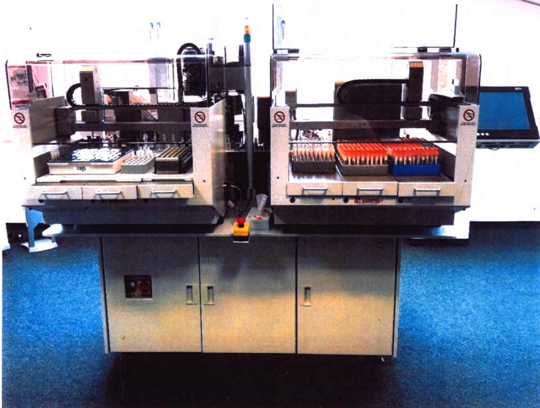
1. Система автоматизированная высокоскоростной сортировки, подготовки и распределения образцов биологических материалов PVS с принадлежностями: общий вид изделия
