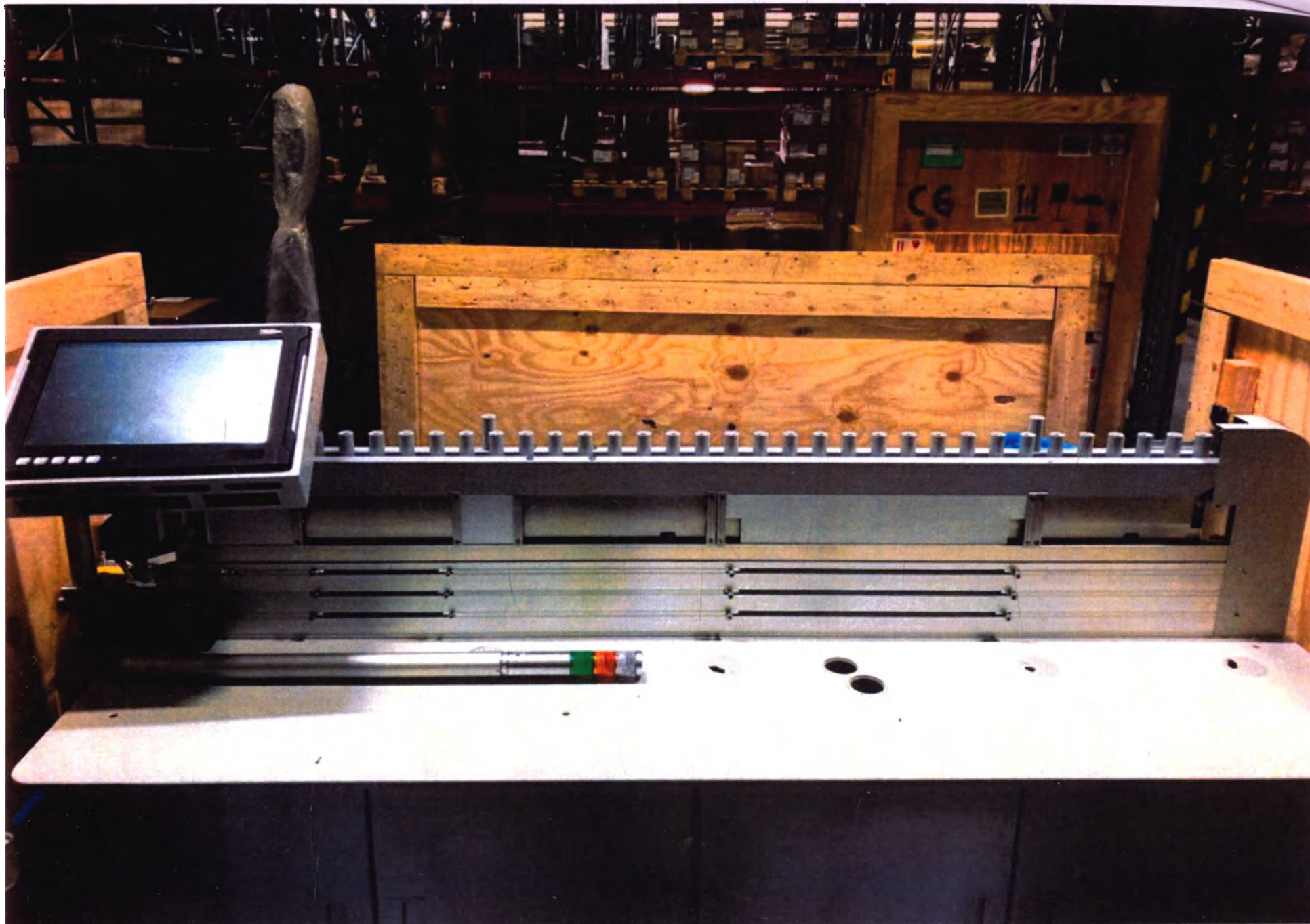
2. Модуль базовый со встроенным панельным компьютером.
