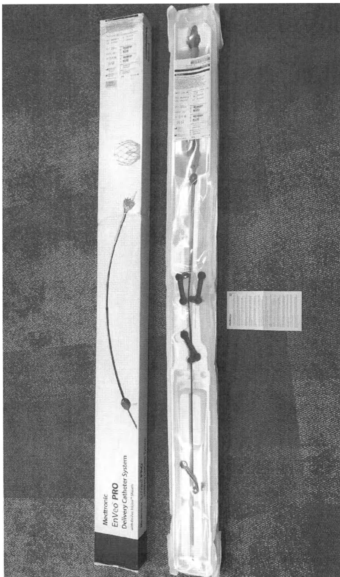
Пример упаковки Системы катетерной доставки EnVeo PRO, наружный диаметр 20 Fg (6,7 мм)
