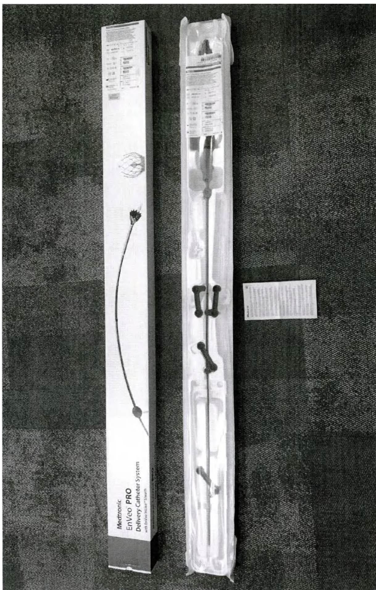
Пример упаковки Системы катетерной доставки EnVeo PRO, наружный диаметр 18 Fr (6 мм)
