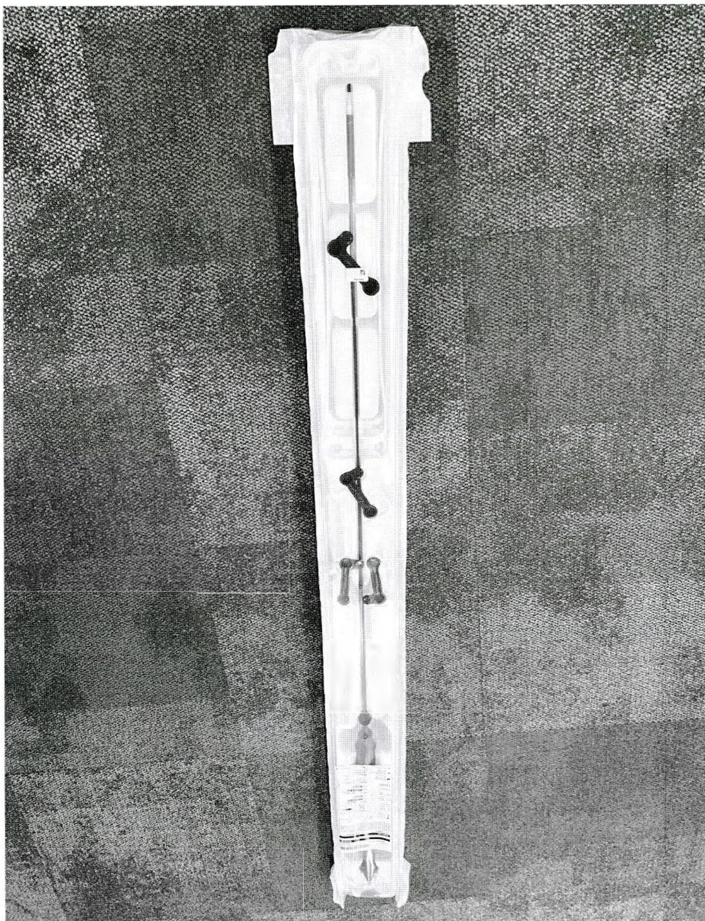
Система катетерной доставки Evolut PRO+, наружный диаметр 22 Fr (7,3 мм) (стерильная упаковка)
