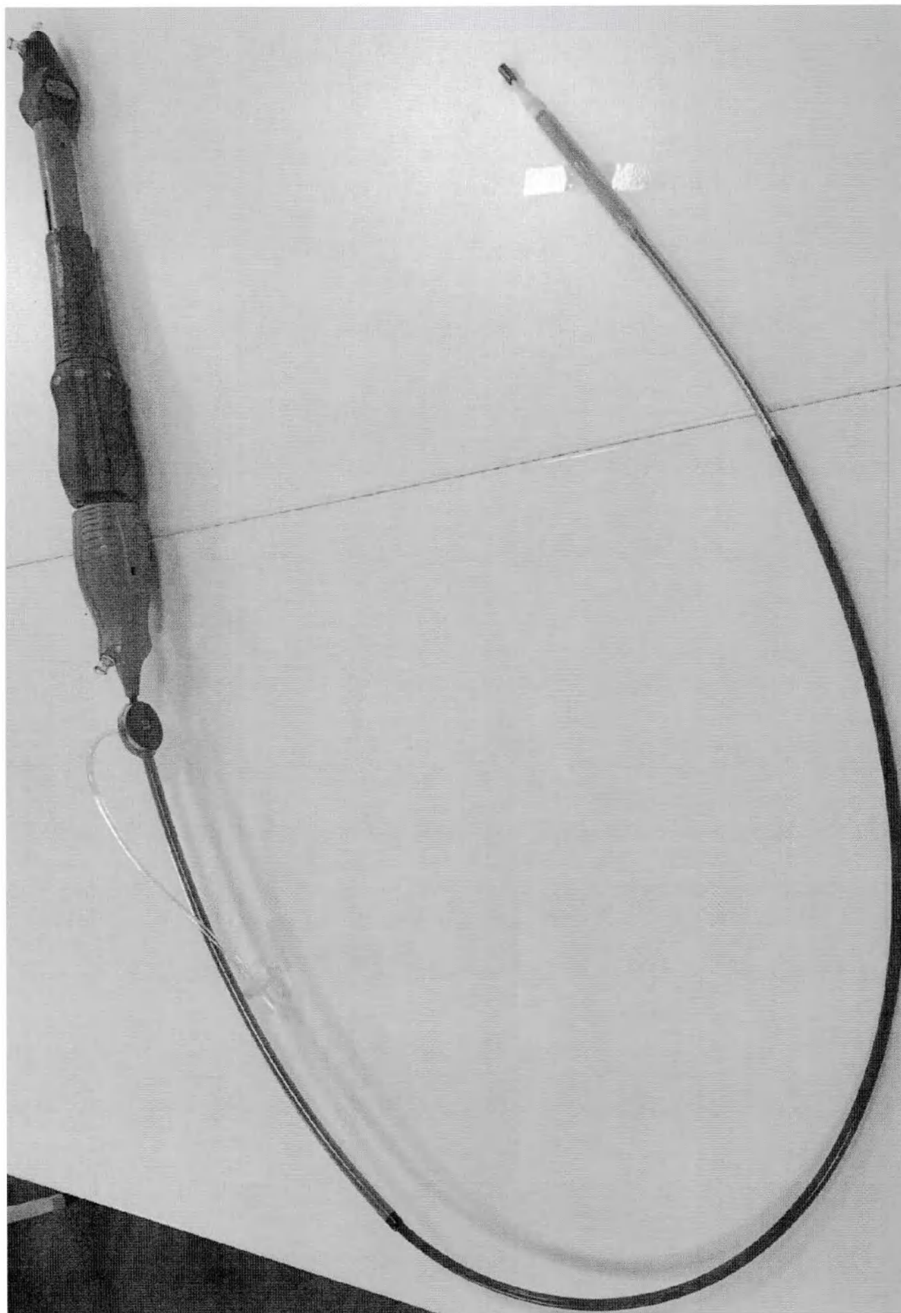
Система катетерной доставки EnVeo PRO, наружный диаметр 20 Fr (6,7 мм)
