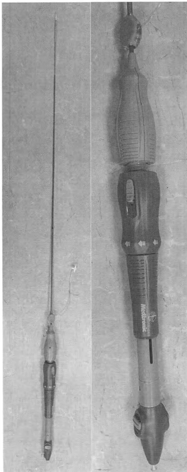
Система катетерной доставки Evolut PRO+, наружный диаметр 18 Fr (6 мм)
