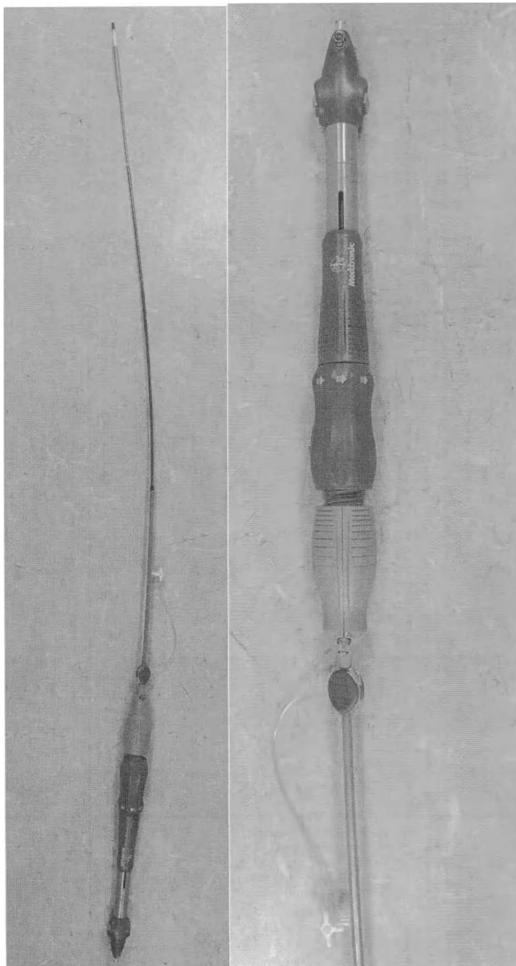
Система катетерной доставки Evolut PRO+, наружный диаметр 22 Fr (7,3 мм)
