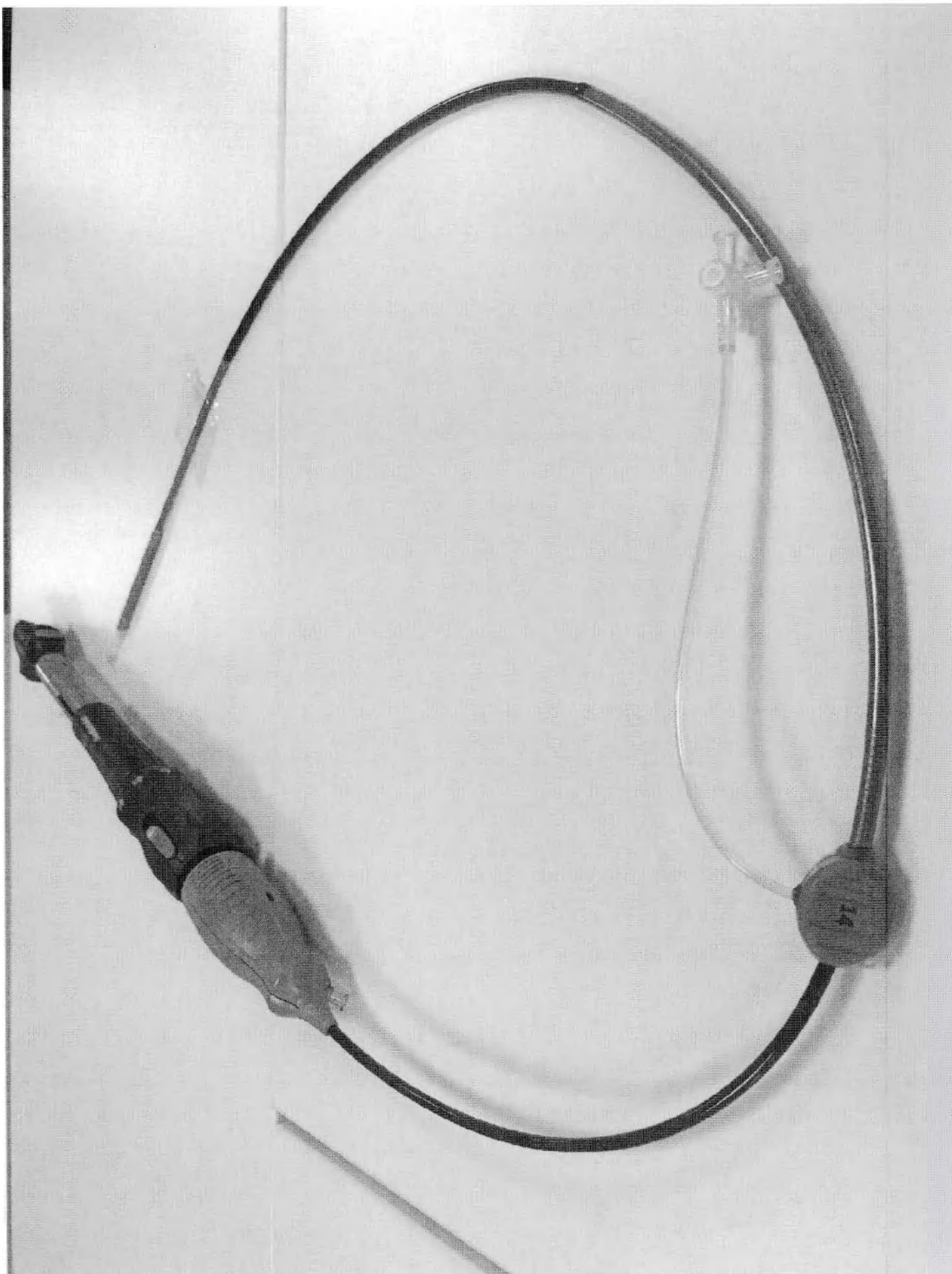
Система катетерной доставки EnVeo PRO, наружный диаметр 18 Fr (6 мм)
