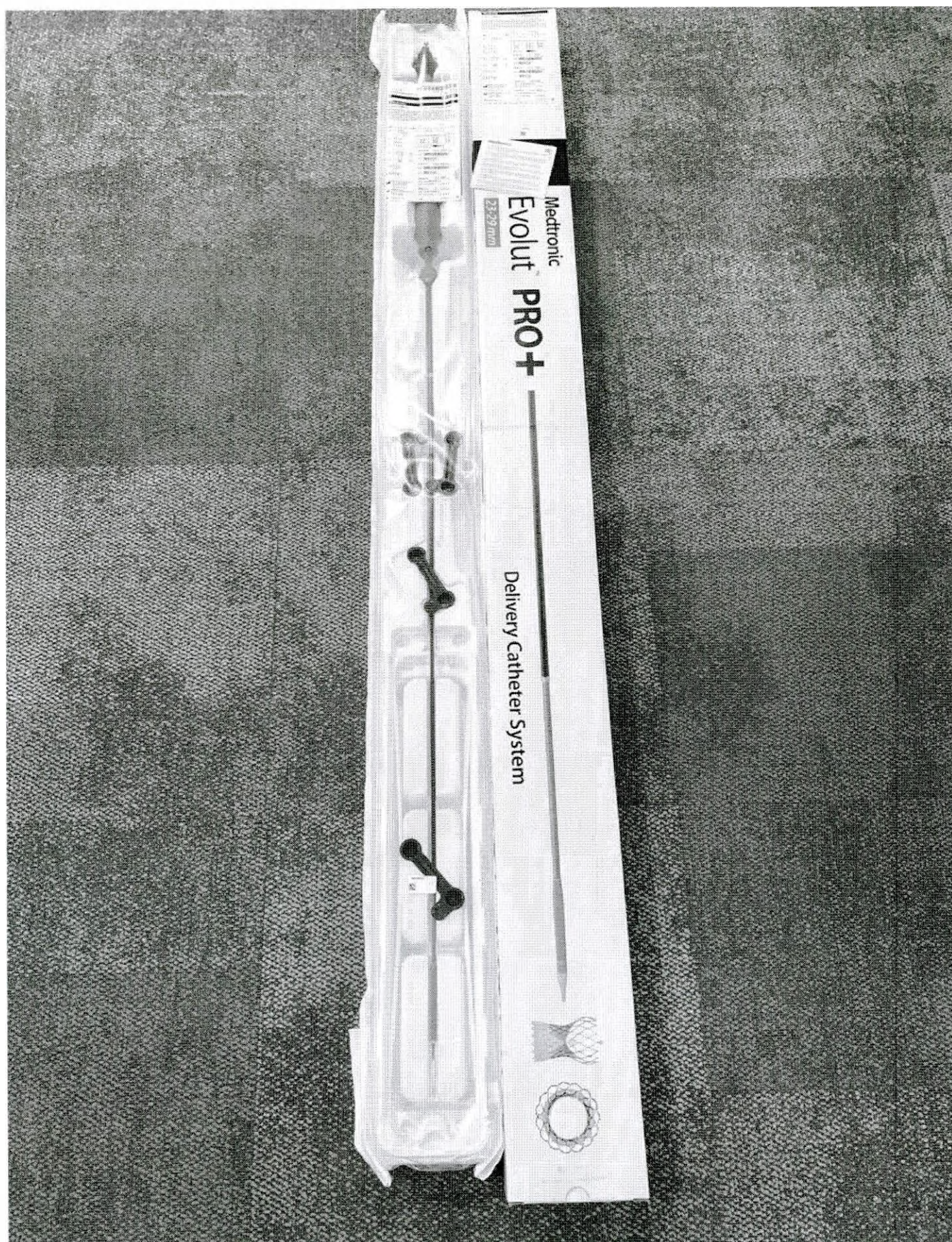
Система катетерной доставки Evolut PRO+, наружный диаметр 18 Fr (6 мм) (общий вид)
